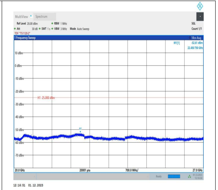
7-7-15MHz-5MHz-QPSK-QPSK-20825-20918-75RB#0-25RB# 0-20000~27000MHz-PASS
