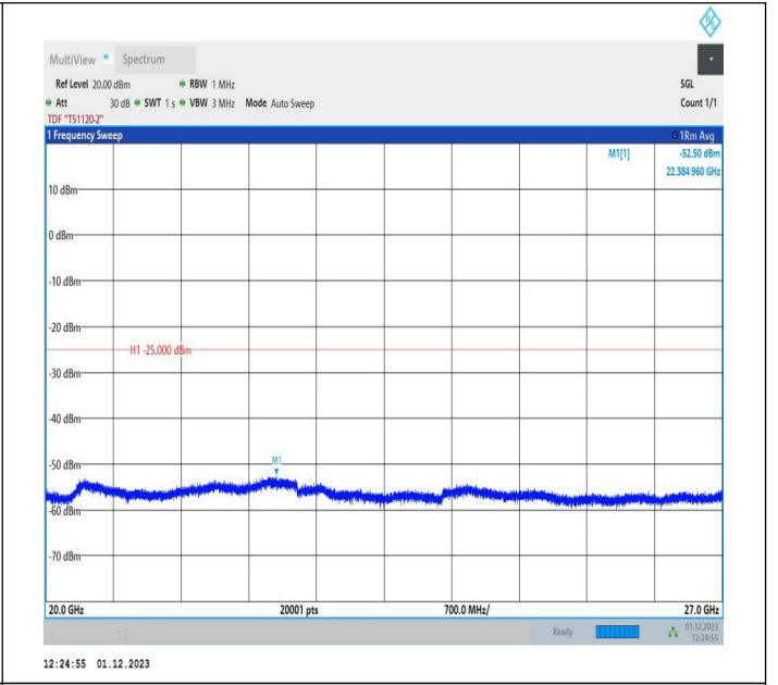
7-7-15MHz-5MHz-QPSK-QPSK-21076-21169-75RB#0-25RB# 0-20000~27000MHz-PASS
