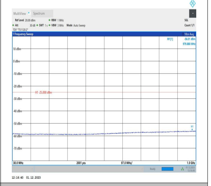
7-7-15MHz-5MHz-QPSK-QPSK-20825-20918-75RB#0-25RB# 0-30~1000MHz-PASS
