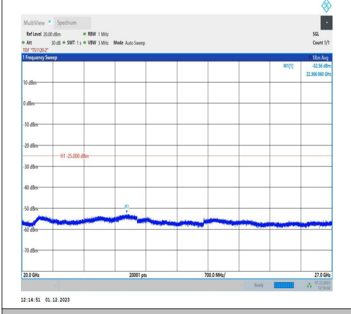
7-7-15MHz-5MHz-QPSK-QPSK-20825-20918-1RB#0-1RB#24 -20000~27000MHz-PASS
