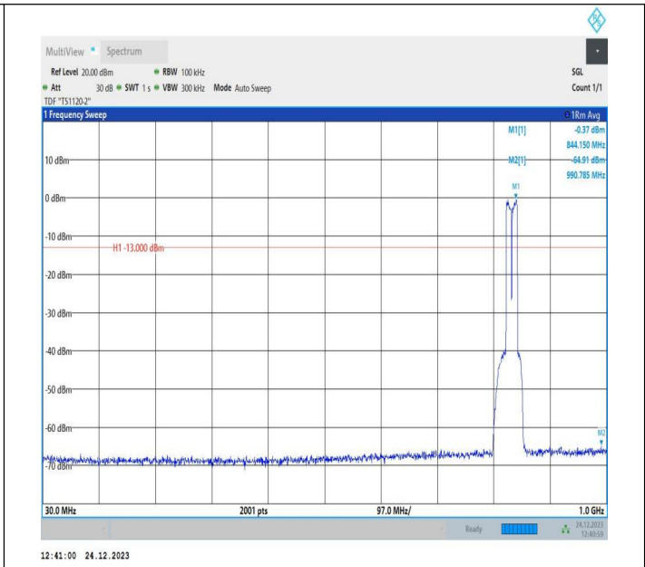
5-5-10MHz-10MHz-QPSK-QPSK-20476-20575-50RB#0-50RB #0-30~1000MHz-PASS
