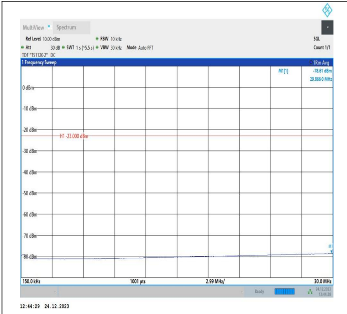
5-5-10MHz-10MHz-QPSK-QPSK-20501-20600-50RB#0-50RB #0-0.15~30MHz-PASS
