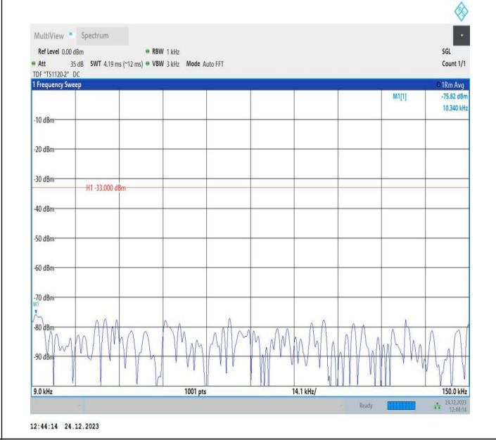
5-5-10MHz-10MHz-QPSK-QPSK-20501-20600-50RB#0-50RB #0-0.009~0.15MHz-PASS
