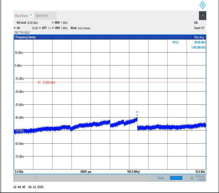
5-5-10MHz-10MHz-QPSK-QPSK-20501-20600-50RB#0-50RB #0-3000~10000MHz-PASS
