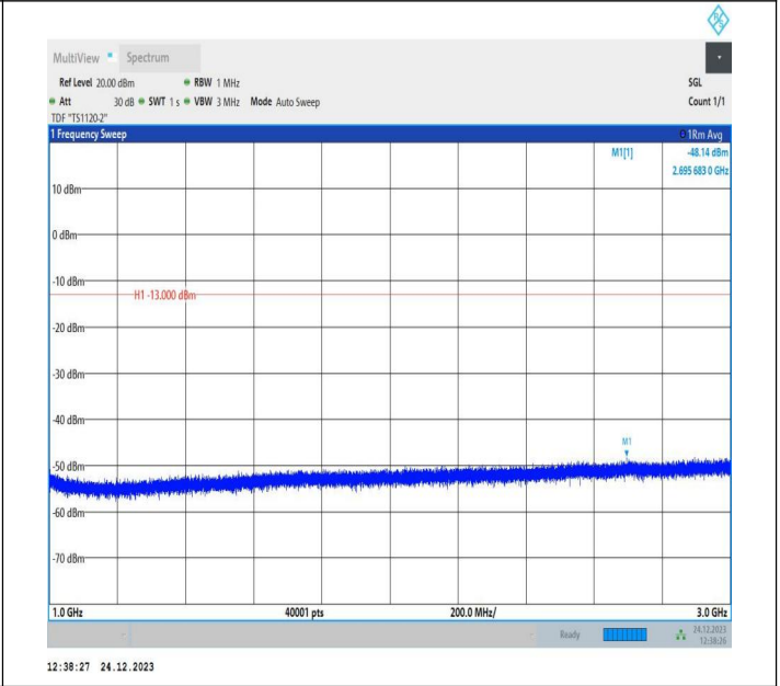
5-5-10MHz-10MHz-QPSK-QPSK-20476-20575-1RB#0-0RB#0 1000~3000MHz-PASS
