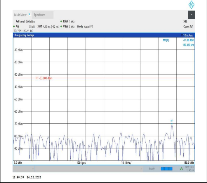
5-5-10MHz-10MHz-QPSK-QPSK-20476-20575-50RB#0-50RB #0-0.009~0.15MHz-PASS
