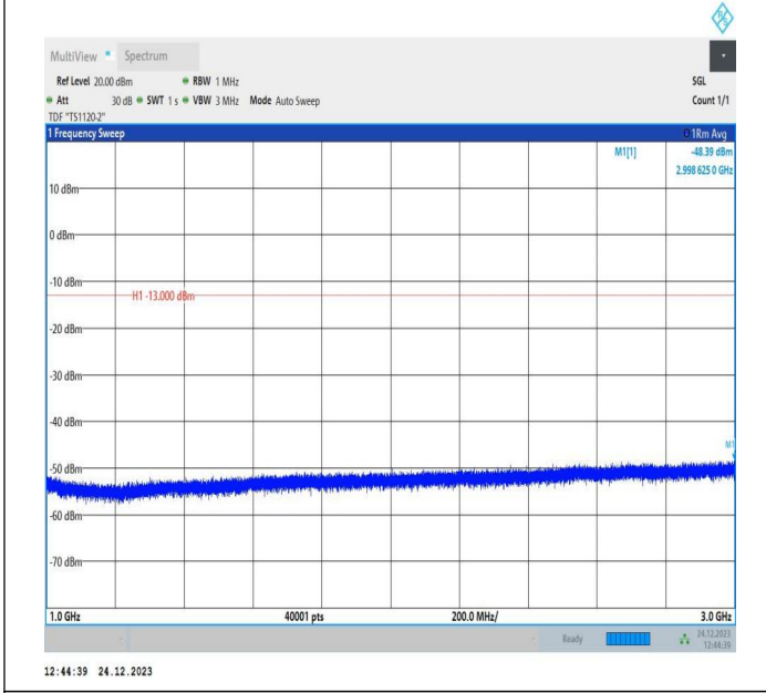
5-5-10MHz-10MHz-QPSK-QPSK-20501-20600-50RB#0-50RB #0-1000~3000MHz-PASS
