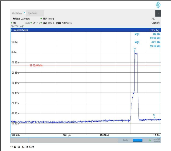
5-5-10MHz-10MHz-QPSK-QPSK-20501-20600-50RB#0-50RB #0-30~1000MHz-PASS
