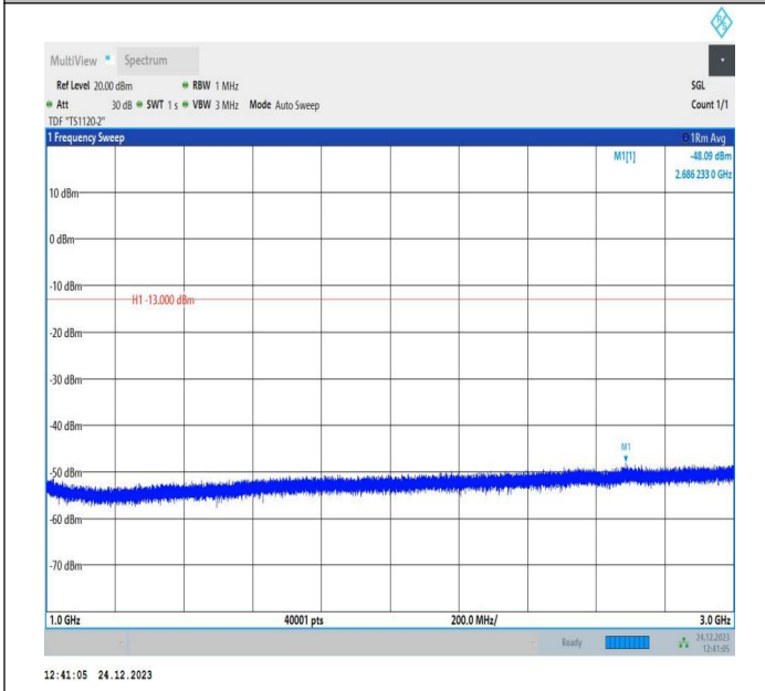
5-5-10MHz-10MHz-QPSK-QPSK-20476-20575-50RB#0-50RB #0-1000~3000MHz-PASS
