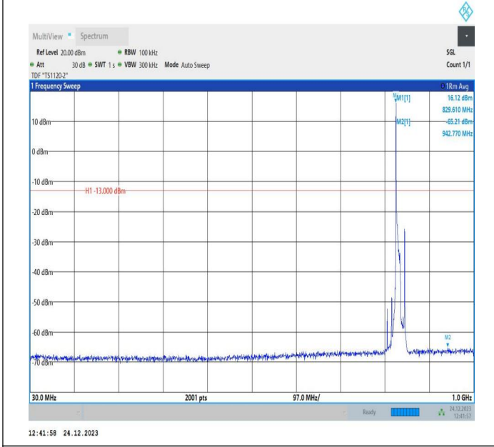
5-5-10MHz-10MHz-QPSK-QPSK-20501-20600-1RB#0-0RB#0 -30~1000MHz-PASS
