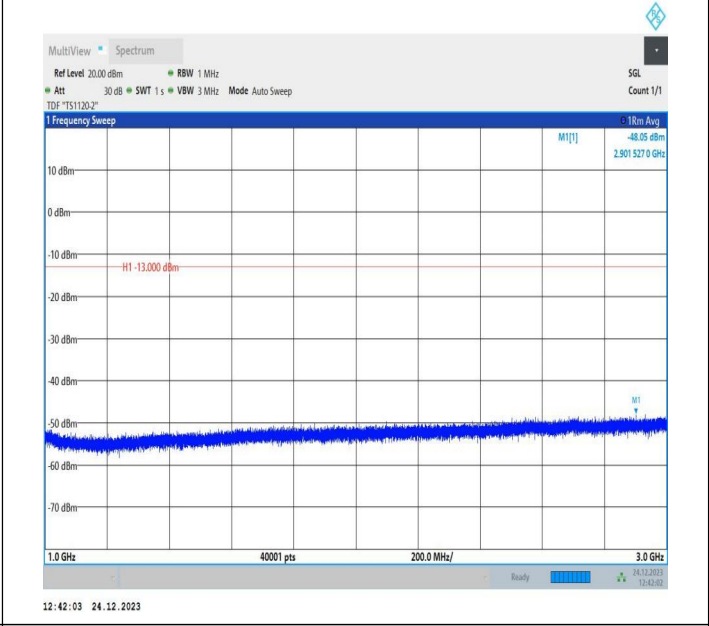
5-5-10MHz-10MHz-QPSK-QPSK-20501-20600-1RB#0-0RB#0 1000~3000MHz-PASS
