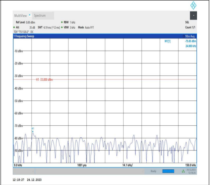
5-5-5MHz-10MHz-QPSK-QPSK-20528-20600-25RB#0-50RB# 0-0.009~0.15MHz-PASS
