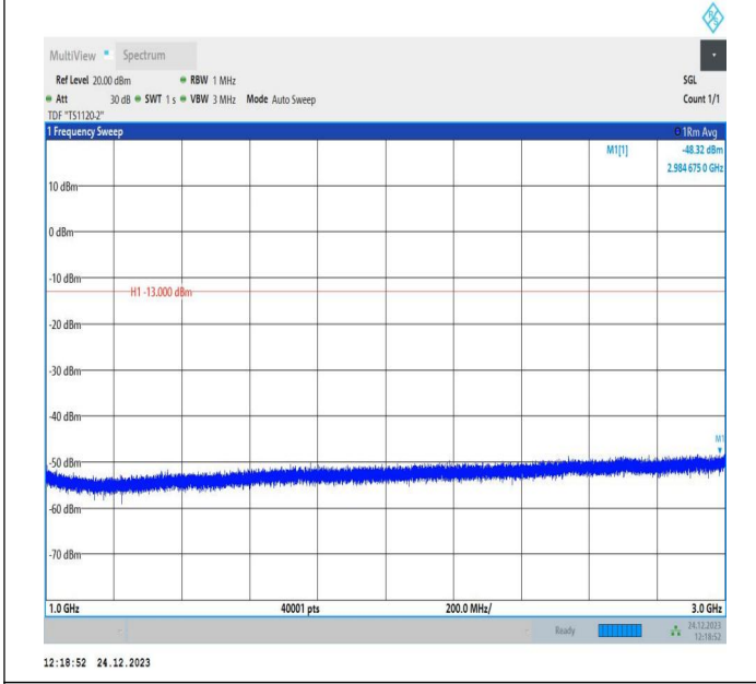
5-5-5MHz-10MHz-QPSK-QPSK-20528-20600-25RB#0-50RB# 0-1000~3000MHz-PASS
