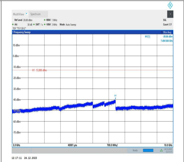
5-5-5MHz-10MHz-QPSK-QPSK-20528-20600-1RB#24-0RB#0 3000~10000MHz-PASS
