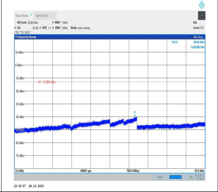
5-5-5MHz-10MHz-QPSK-QPSK-20528-20600-25RB#0-50RB# 0-3000~10000MHz-PASS
