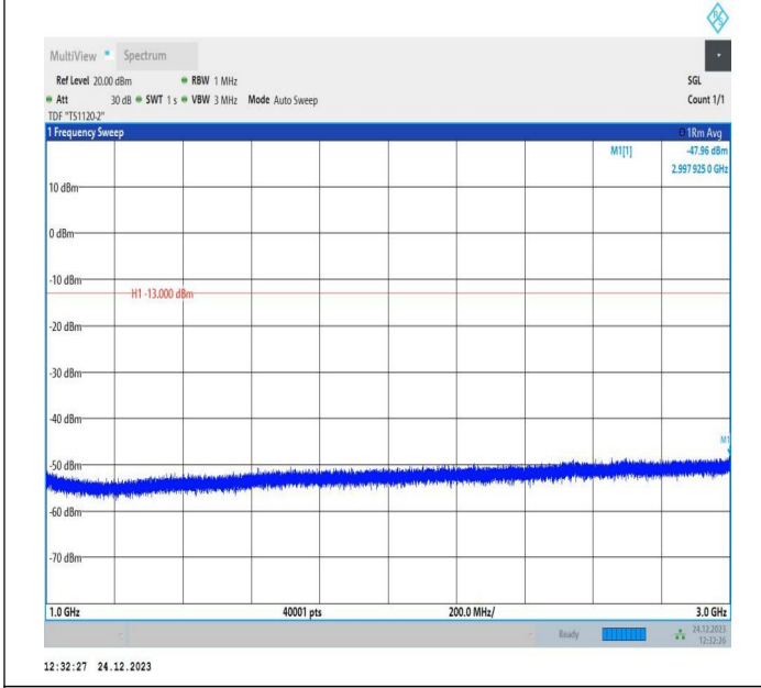
5-5-10MHz-5MHz-QPSK-QPSK-20550-20622-50RB#0-25RB# 0-1000~3000MHz-PASS
