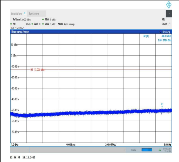
5-5-10MHz-10MHz-QPSK-QPSK-20450-20549-50RB#0-50RB #0-1000~3000MHz-PASS
