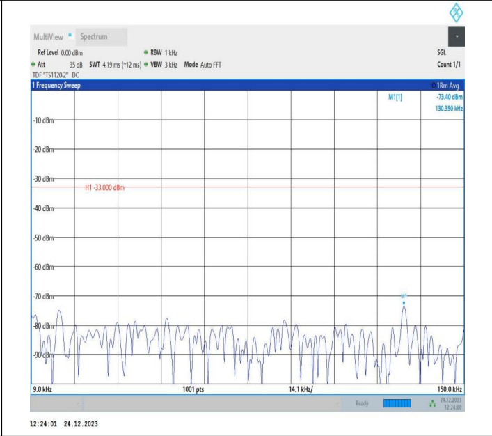
5-5-10MHz-5MHz-QPSK-QPSK-20450-20522-50RB#0-25RB# 0-0.009~0.15MHz-PASS
