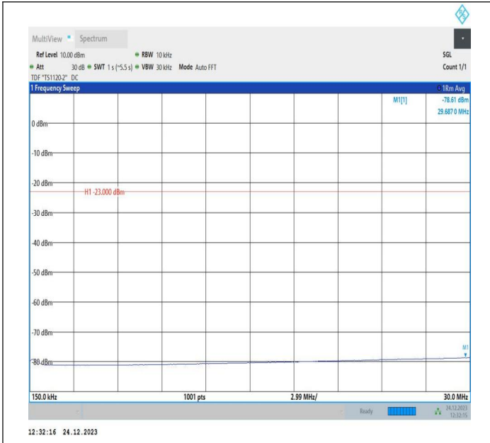
5-5-10MHz-5MHz-QPSK-QPSK-20550-20622-50RB#0-25RB# 0-0.15~30MHz-PASS
