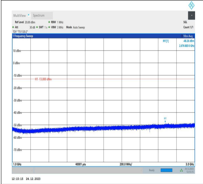
5-5-5MHz-10MHz-QPSK-QPSK-20478-20550-25RB#0-50RB# 0-1000~3000MHz-PASS
