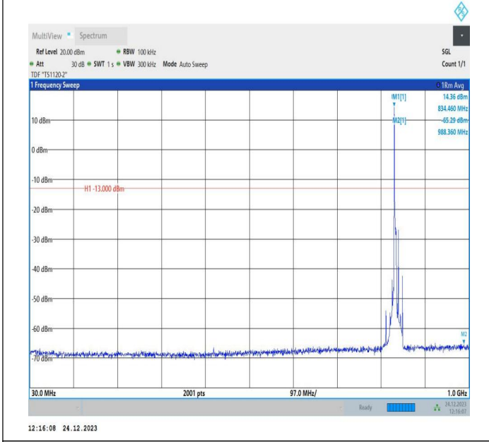
5-5-5MHz-10MHz-QPSK-QPSK-20528-20600-1RB#0-0RB#0-30~1000MHz-PASS
