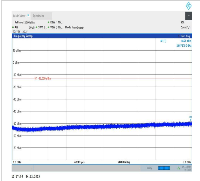
5-5-5MHz-10MHz-QPSK-QPSK-20528-20600-1RB#24-0RB#0 -1000~3000MHz-PASS
