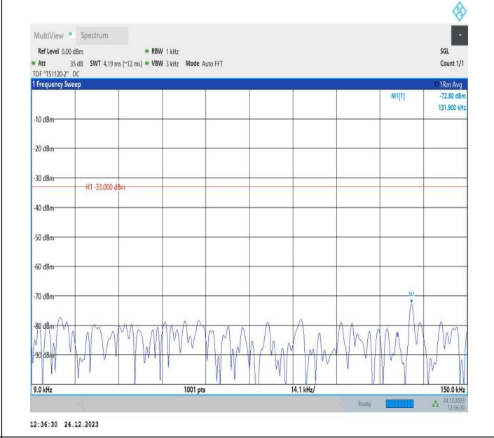
5-5-10MHz-10MHz-QPSK-QPSK-20450-20549-50RB#0-50RB #0-0.009~0.15MHz-PASS
