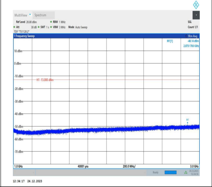
5-5-10MHz-10MHz-QPSK-QPSK-20450-20549-1RB#0-0RB#0 1000~3000MHz-PASS
