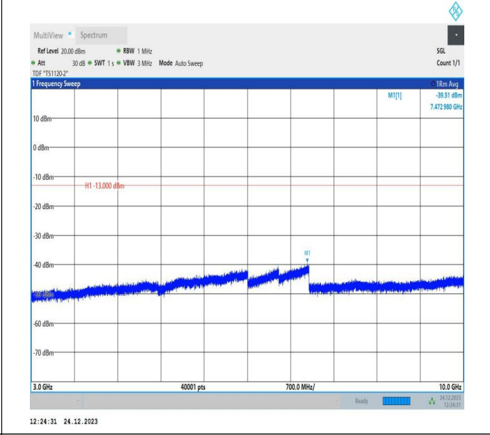
5-5-10MHz-5MHz-QPSK-QPSK-20450-20522-50RB#0-25RB# 0-3000~10000MHz-PASS
