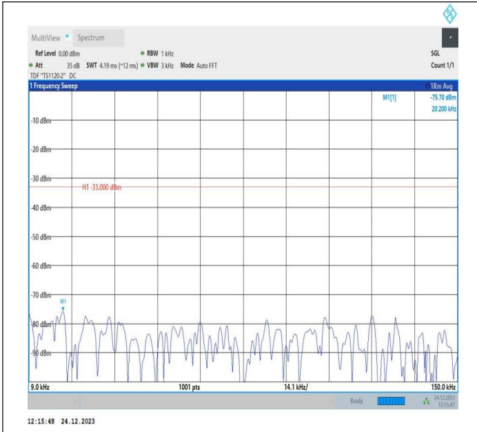
5-5-5MHz-10MHz-QPSK-QPSK-20528-20600-1RB#0-0RB#0-0.009~0.15MHz-PASS
