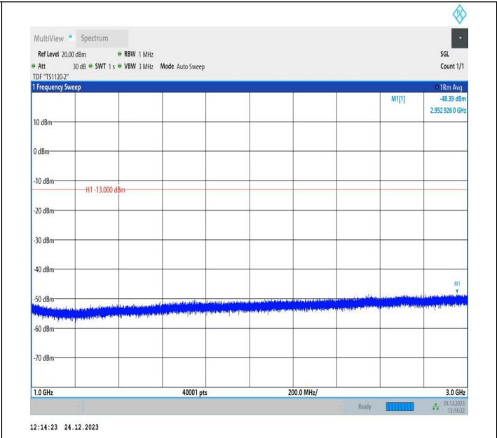
5-5-5MHz-10MHz-QPSK-QPSK-20478-20550-1RB#0-1RB#49- 1000~3000MHz-PASS
