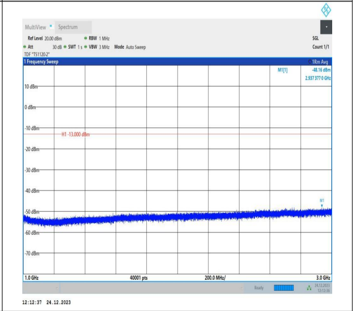
5-5-5MHz-10MHz-QPSK-QPSK-20478-20550-1RB#0-0RB#0-1000~3000MHz-PASS
