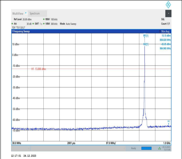
5-5-5MHz-10MHz-QPSK-QPSK-20528-20600-1RB#24-0RB#0-30~1000MHz-PASS
