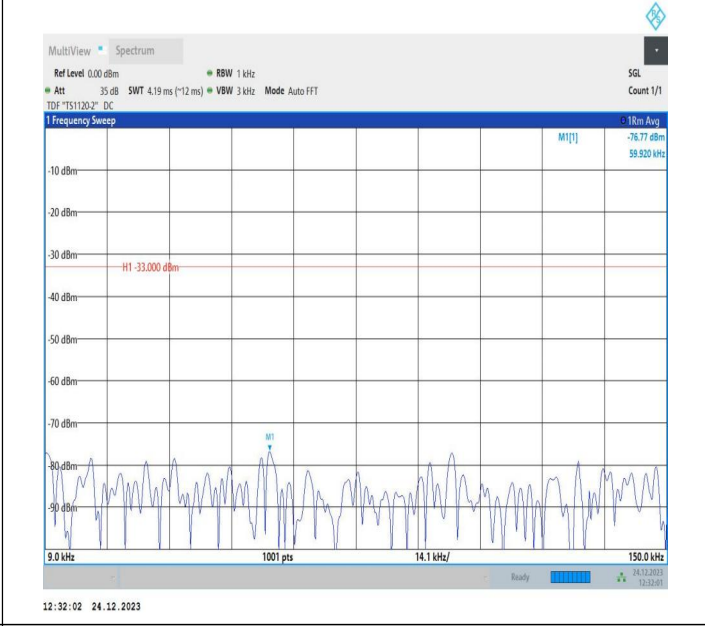
5-5-10MHz-5MHz-QPSK-QPSK-20550-20622-50RB#0-25RB# 0-0.009~0.15MHz-PASS
