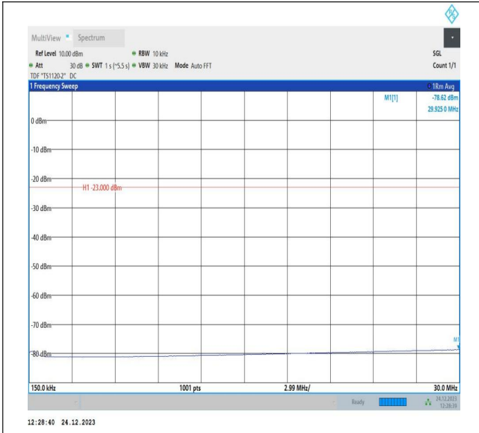
5-5-10MHz-5MHz-QPSK-QPSK-20500-20572-50RB#0-25RB# 0-0.15~30MHz-PASS
