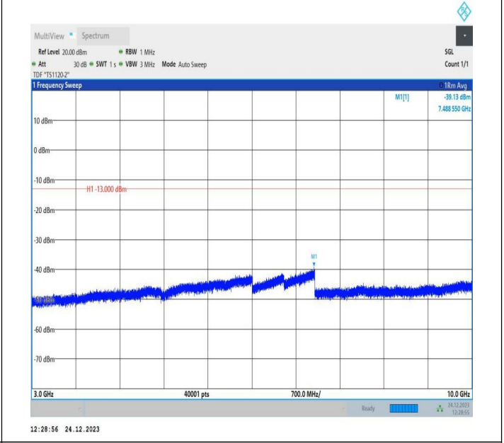
5-5-10MHz-5MHz-QPSK-QPSK-20500-20572-50RB#0-25RB# 0-3000~10000MHz-PASS
