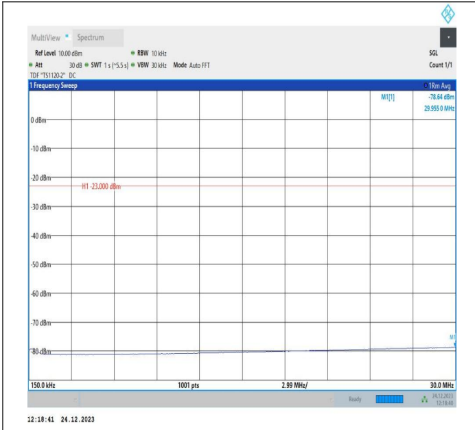
5-5-5MHz-10MHz-QPSK-QPSK-20528-20600-25RB#0-50RB# 0-0.15~30MHz-PASS
