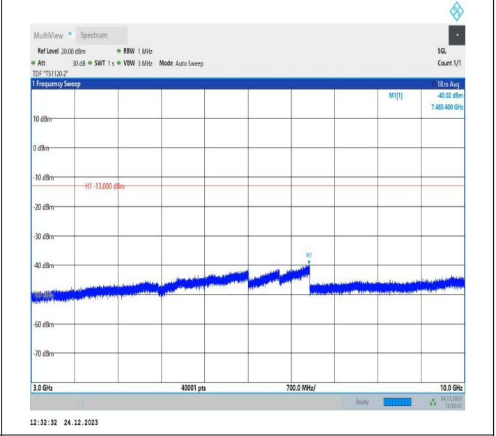
5-5-10MHz-5MHz-QPSK-QPSK-20550-20622-50RB#0-25RB# 0-3000~10000MHz-PASS
