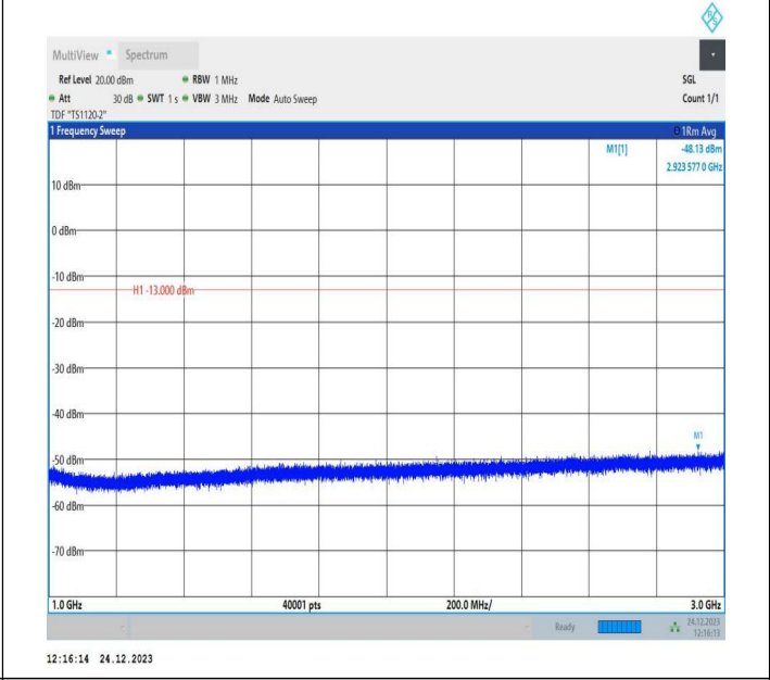
5-5-5MHz-10MHz-QPSK-QPSK-20528-20600-1RB#0-0RB#0-1000~3000MHz-PASS
