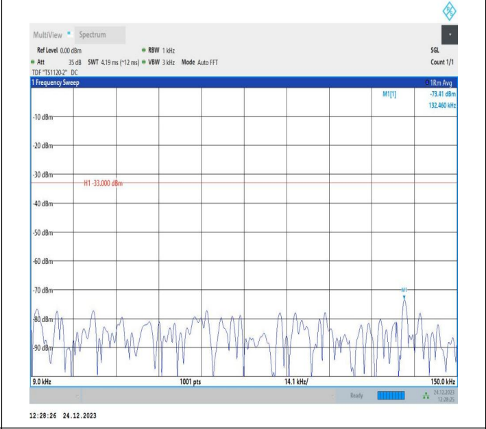
5-5-10MHz-5MHz-QPSK-QPSK-20500-20572-50RB#0-25RB# 0-0.009~0.15MHz-PASS
