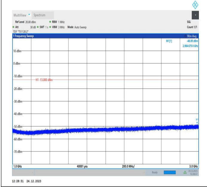
5-5-10MHz-5MHz-QPSK-QPSK-20500-20572-50RB#0-25RB# 0-1000~3000MHz-PASS
