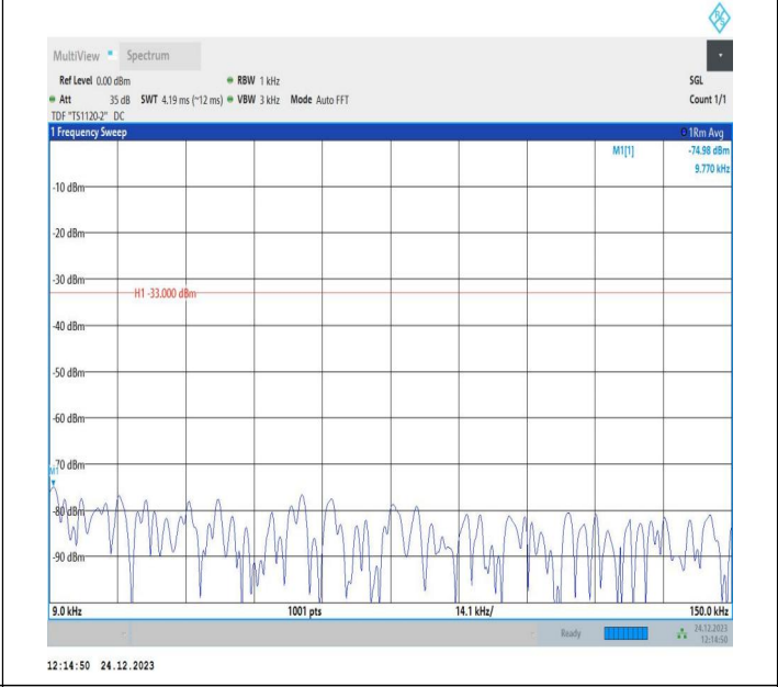
5-5-5MHz-10MHz-QPSK-QPSK-20478-20550-25RB#0-50RB# 0-0.009~0.15MHz-PASS
