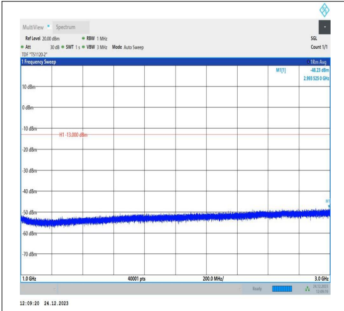
5-5-5MHz-10MHz-QPSK-QPSK-20428-20500-1RB#24-0RB#0 -1000~3000MHz-PASS
