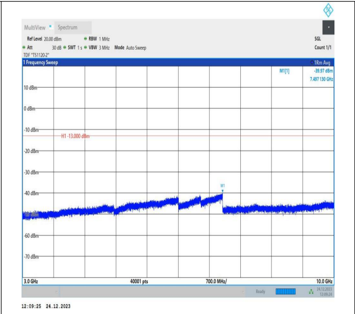
5-5-5MHz-10MHz-QPSK-QPSK-20428-20500-1RB#24-0RB#0- 3000~10000MHz-PASS
