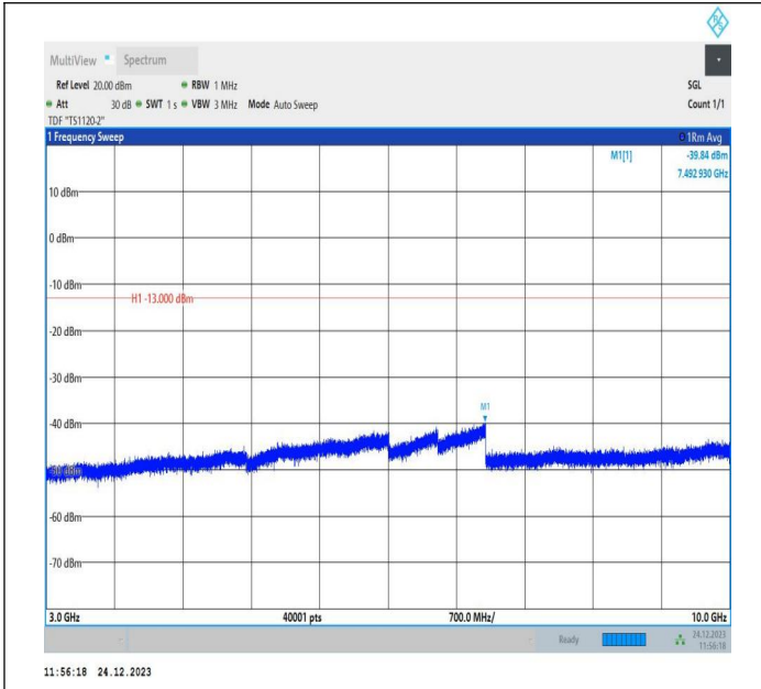
5-5-5MHz-3MHz-QPSK-QPSK-20425-20464-1RB#0-0RB#0-3 000~1000MHz-PASS
