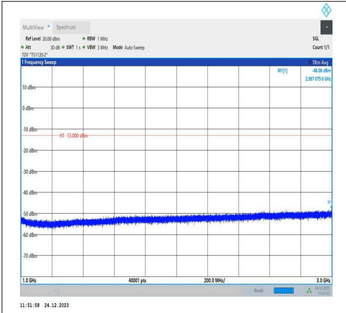
5-5-3MHz-5MHz-QPSK-QPSK-20586-20625-1RB#14-0RB#0-1000~3000MHz-PASS
