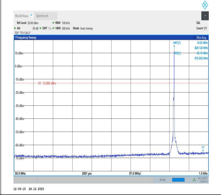
5-5-5MHz-10MHz-QPSK-QPSK-20428-20500-1RB#24-0RB#0-30~1000MHz-PASS
