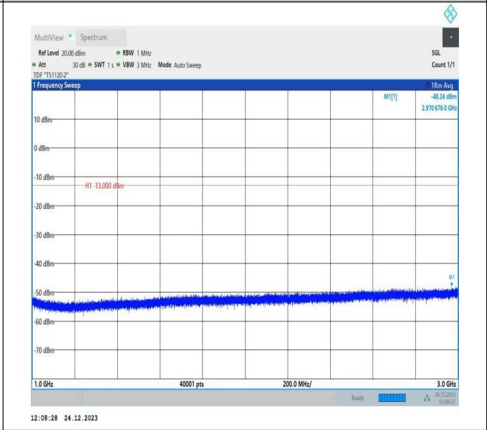
5-5-5MHz-10MHz-QPSK-QPSK-20428-20500-1RB#0-0RB#0-1000~3000MHz-PASS
