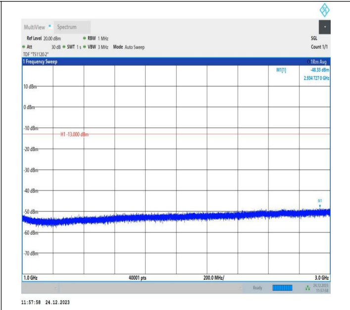
5-5-5MHz-3MHz-QPSK-QPSK-20425-20464-1RB#0-1RB#15-1000~3000MHz-PASS
