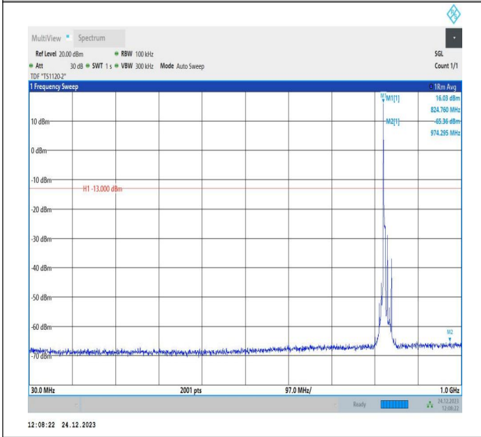
5-5-5MHz-10MHz-QPSK-QPSK-20428-20500-1RB#0-0RB#0-30~1000MHz-PASS
