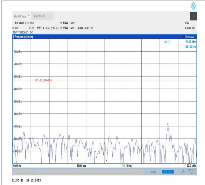
5-5-3MHz-5MHz-QPSK-QPSK-20586-20625-1RB#0-0RB#0-0. 009~0.15MHz-PASS
