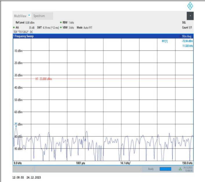
5-5-5MHz-10MHz-QPSK-QPSK-20428-20500-1RB#24-0RB#0-0.009~0.15MHz-PASS
