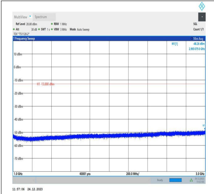
5-5-5MHz-3MHz-QPSK-QPSK-20425-20464-1RB#24-0RB#0-1000~3000MHz-PASS
