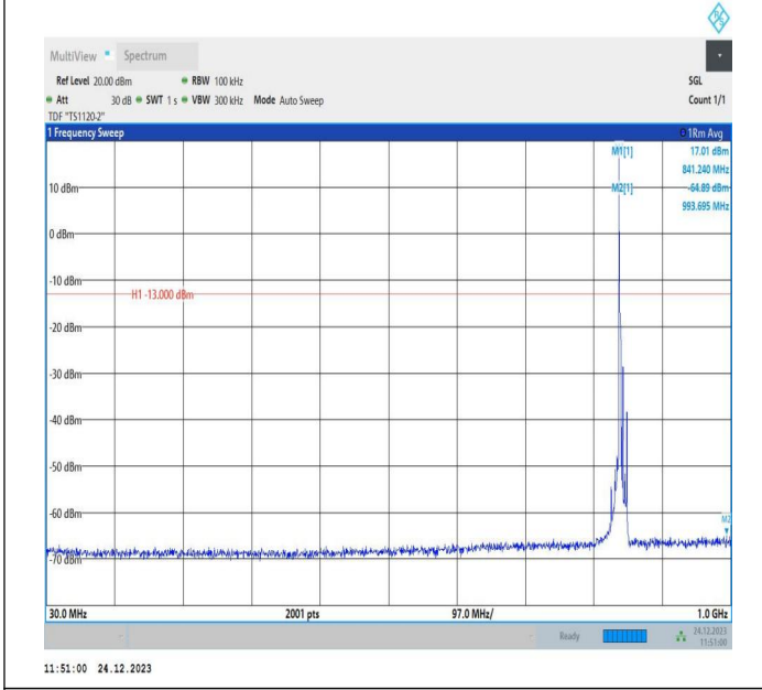
5-5-3MHz-5MHz-QPSK-QPSK-20586-20625-1RB#0-0RB#0-3 0~1000MHz-PASS
