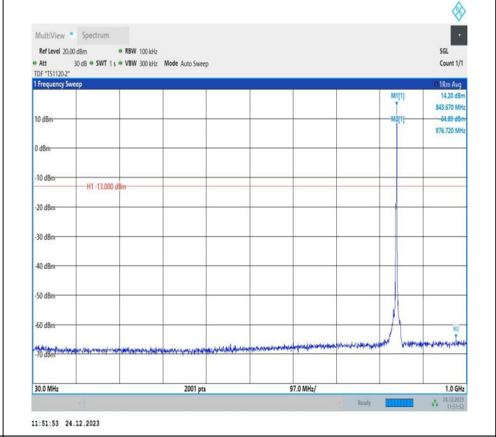
5-5-3MHz-5MHz-QPSK-QPSK-20586-20625-1RB#14-0RB#0-3 0~1000MHz-PASS
