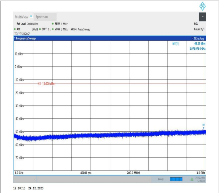
5-5-5MHz-10MHz-QPSK-QPSK-20428-20500-1RB#0-1RB#49- 1000~3000MHz-PASS
