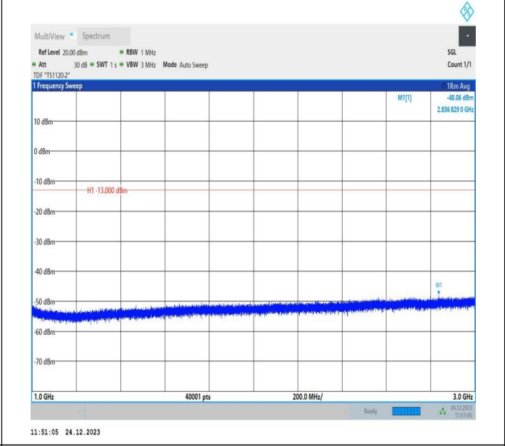
5-5-3MHz-5MHz-QPSK-QPSK-20586-20625-1RB#0-0RB#0-10 00~3000MHz-PASS
