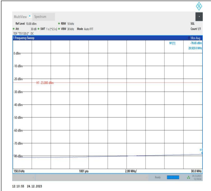
5-5-5MHz-10MHz-QPSK-QPSK-20428-20500-25RB#0-50RB# 0-0.15~30MHz-PASS
