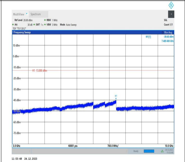
5-5-3MHz-5MHz-QPSK-QPSK-20586-20625-15RB#0-25RB#0- 3000~10000MHz-PASS
