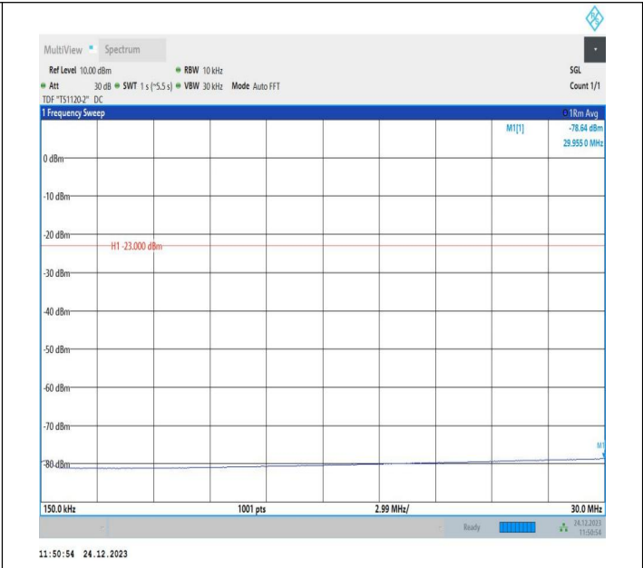
5-5-3MHz-5MHz-QPSK-QPSK-20586-20625-1RB#0-0RB#0-0. 15~30MHz-PASS
