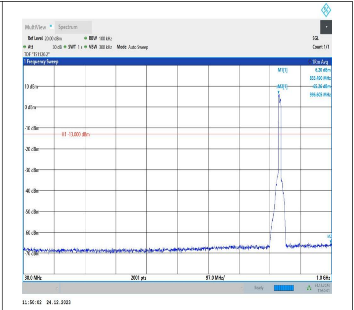
5-5-3MHz-5MHz-QPSK-QPSK-20501-20540-15RB#0-25RB#0- 30~1000MHz-PASS
