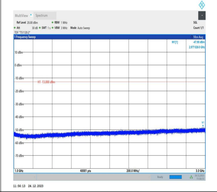
5-5-5MHz-3MHz-QPSK-QPSK-20425-20464-1RB#0-0RB#0-10 00~3000MHz-PASS
