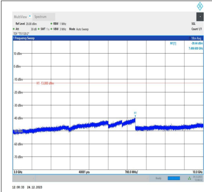
5-5-5MHz-10MHz-QPSK-QPSK-20428-20500-1RB#0-0RB#0-3000~10000MHz-PASS
