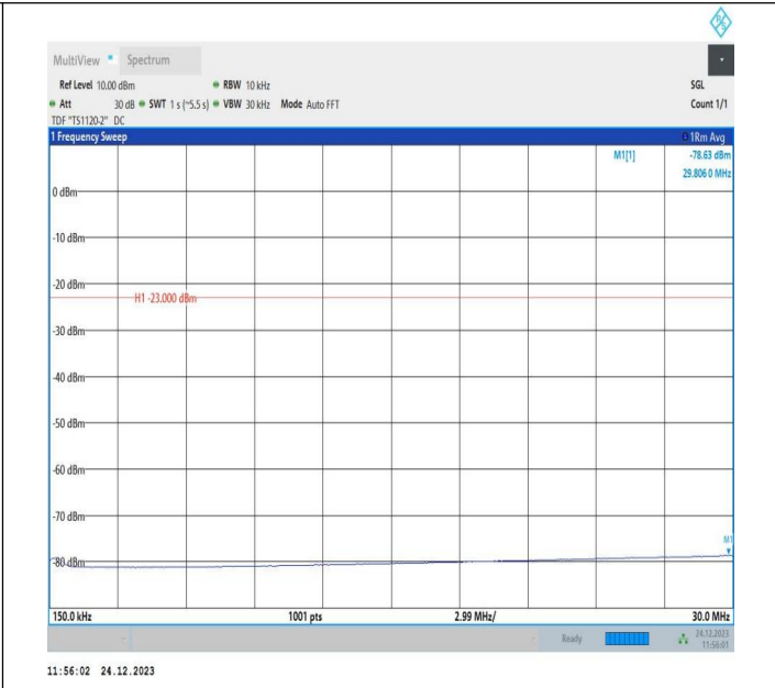
5-5-5MHz-3MHz-QPSK-QPSK-20425-20464-1RB#0-0RB#0-0. 15~30MHz-PASS
