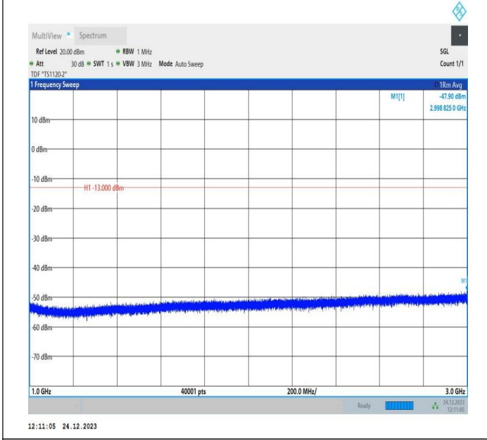
5-5-5MHz-10MHz-QPSK-QPSK-20428-20500-25RB#0-50RB# 0-1000~3000MHz-PASS
