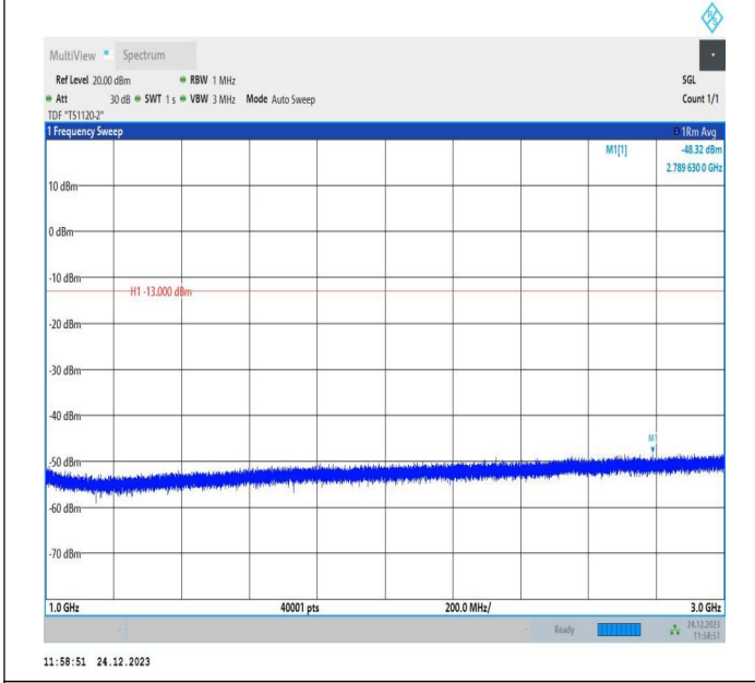
5-5-5MHz-3MHz-QPSK-QPSK-20425-20464-25RB#0-15RB#0 -1000~3000MHz-PASS
