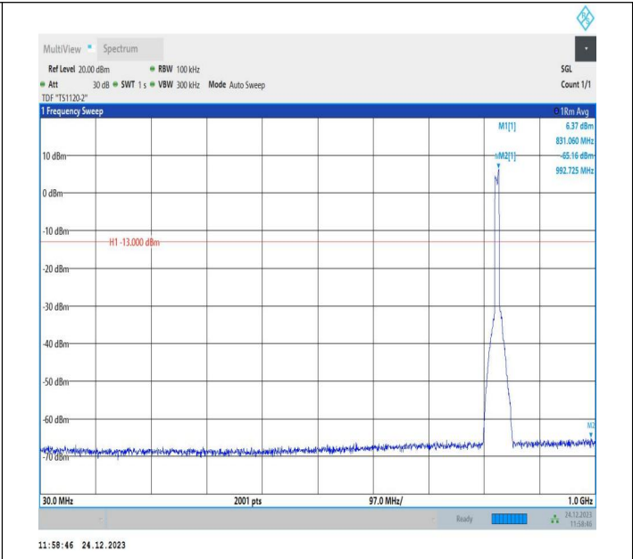
5-5-5MHz-3MHz-QPSK-QPSK-20425-20464-25RB#0-15RB#0- 30~1000MHz-PASS
