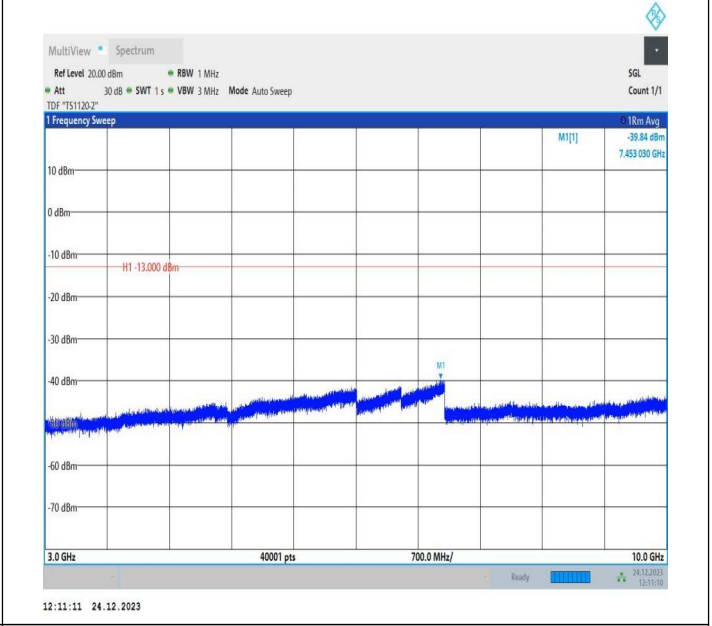
5-5-5MHz-10MHz-QPSK-QPSK-20428-20500-25RB#0-50RB# 0-3000~10000MHz-PASS
