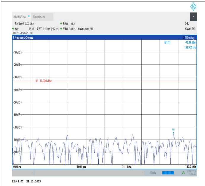
5-5-5MHz-10MHz-QPSK-QPSK-20428-20500-1RB#0-0RB#0-0.009~0.15MHz-PASS
