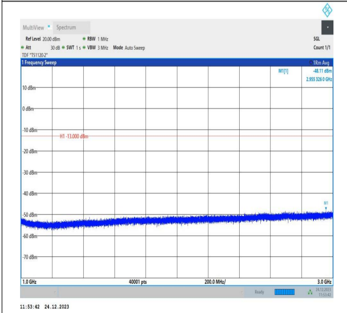
5-5-3MHz-5MHz-QPSK-QPSK-20586-20625-15RB#0-25RB#0 -1000~3000MHz-PASS
