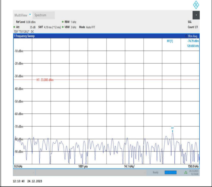
5-5-5MHz-10MHz-QPSK-QPSK-20428-20500-25RB#0-50RB# 0-0.009~0.15MHz-PASS
