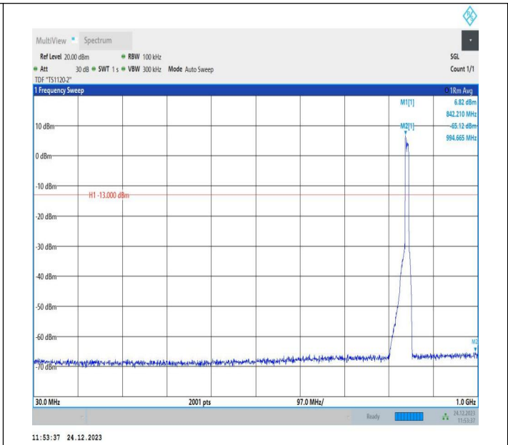
5-5-3MHz-5MHz-QPSK-QPSK-20586-20625-15RB#0-25RB#0- 30~1000MHz-PASS
