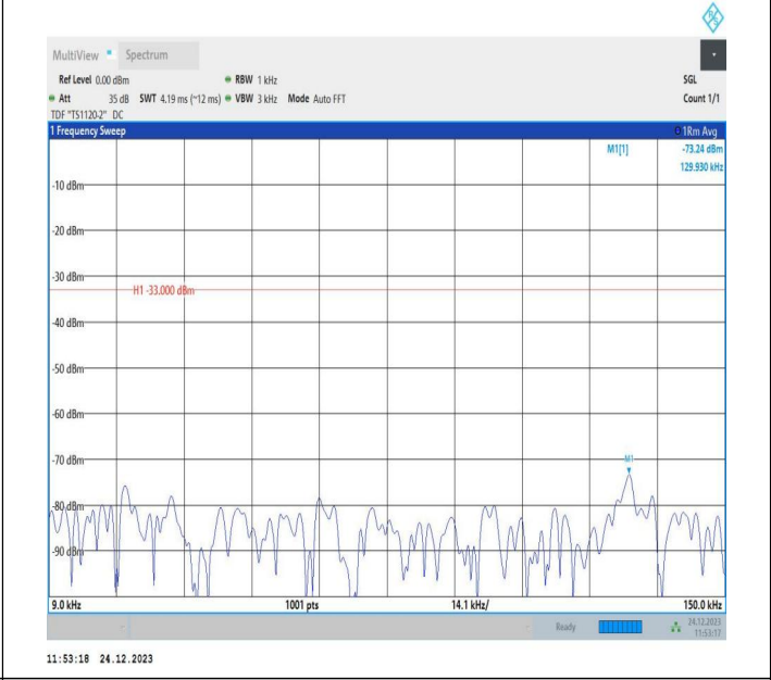
5-5-3MHz-5MHz-QPSK-QPSK-20586-20625-15RB#0-25RB#0-0.009~0.15MHz-PASS
