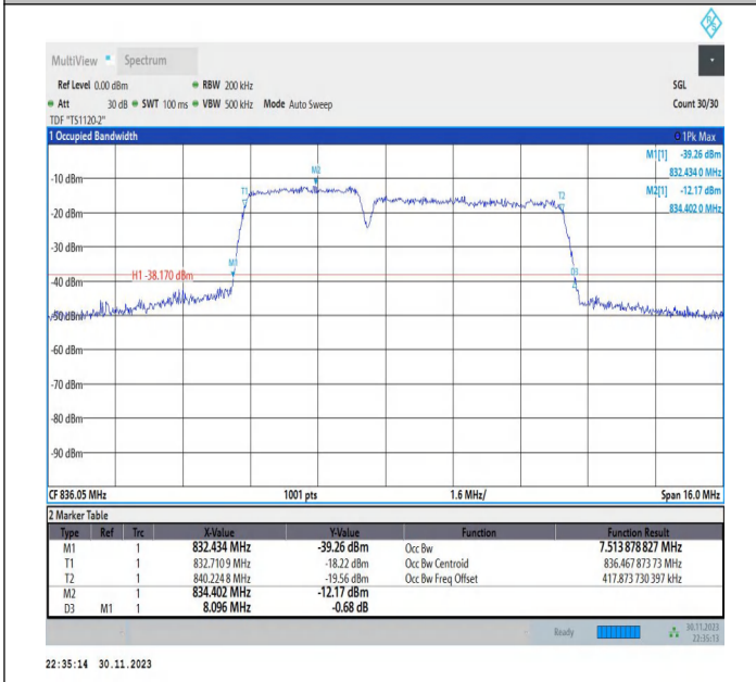
5-5-3MHz-5MHz-QPSK-QPSK-20501-20540-15RB#0-25RB#0 -PASS
