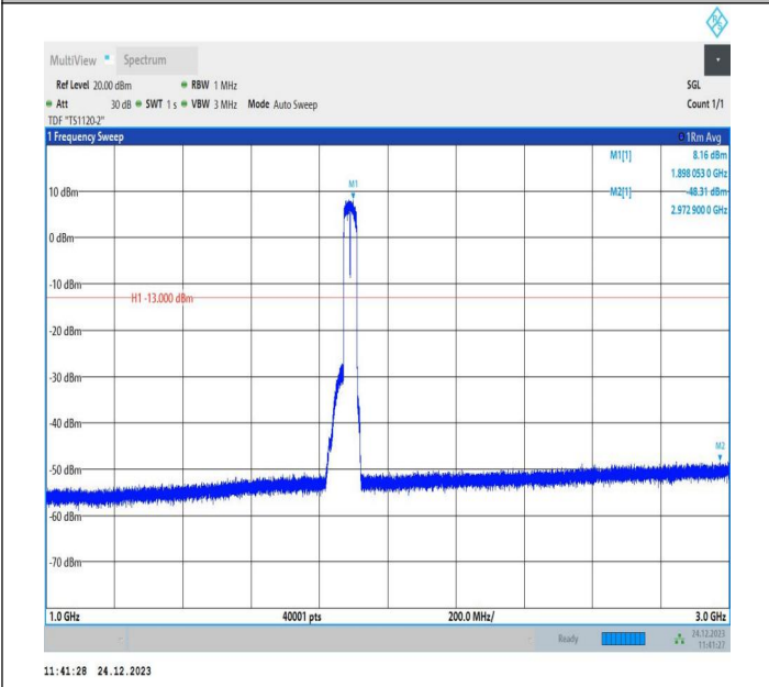
2-2-20MHz-20MHz-QPSK-QPSK-18902-19100-100RB#0-100 RB#0-1000~3000MHz-PASS
