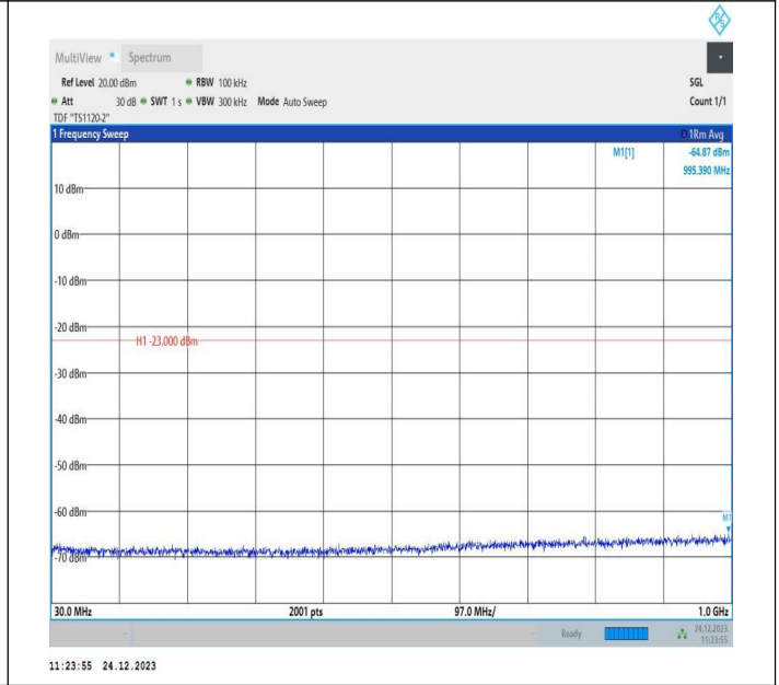
2-2-20MHz-15MHz-QPSK-QPSK-18826-18997-1RB#99-0RB#9 0-30~1000MHz-PASS
