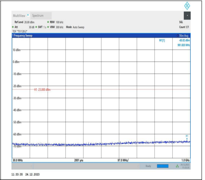
2-2-20MHz-20MHz-QPSK-QPSK-18700-18898-100RB#0-100 RB#0-30~1000MHz-PASS
