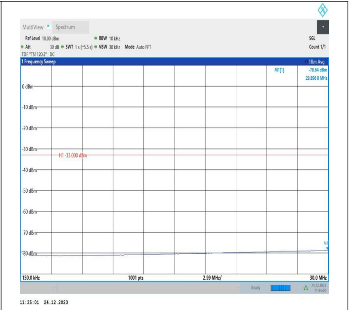
2-2-20MHz-20MHz-QPSK-QPSK-18801-18999-1RB#0-0RB#0 -0.15~30MHz-PASS
