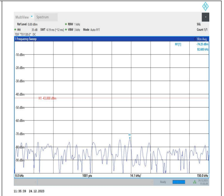
2-2-20MHz-20MHz-QPSK-QPSK-18801-18999-1RB#99-0RB#0 0-0.009~0.15MHz-PASS
