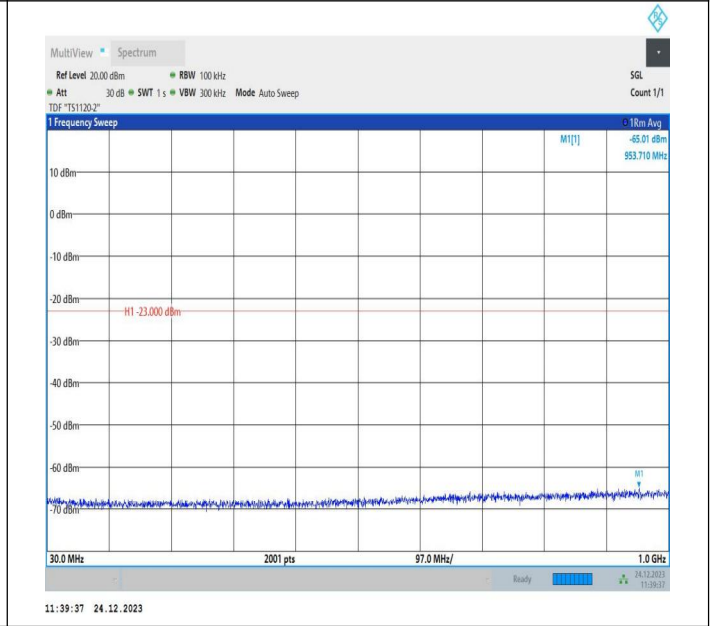
2-2-20MHz-20MHz-QPSK-QPSK-18902-19100-1RB#99-0RB#0 0-30~1000MHz-PASS
