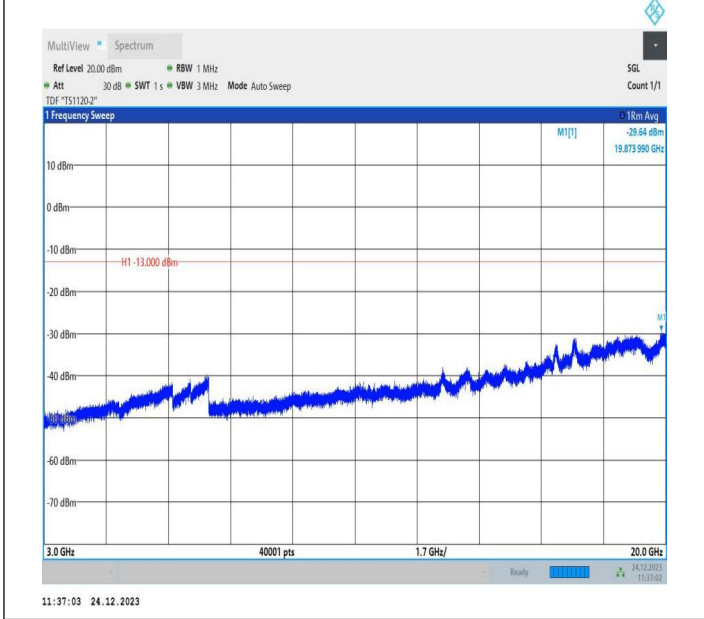
2-2-20MHz-20MHz-QPSK-QPSK-18801-18999-1RB#0-1RB#9 9-3000~20000MHz-PASS
