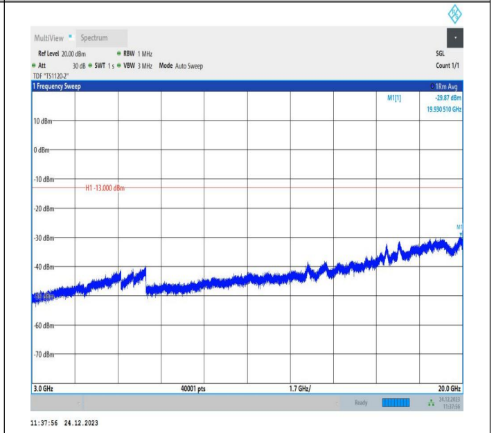
2-2-20MHz-20MHz-QPSK-QPSK-18801-18999-100RB#0-100 RB#0-3000~20000MHz-PASS
