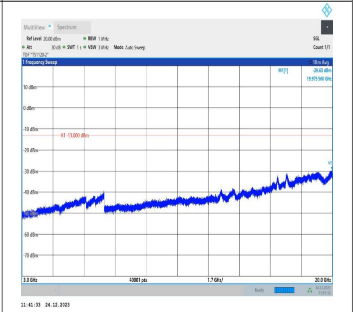
2-2-20MHz-20MHz-QPSK-QPSK-18902-19100-100RB#0-100 RB#0-3000~20000MHz-PASS
