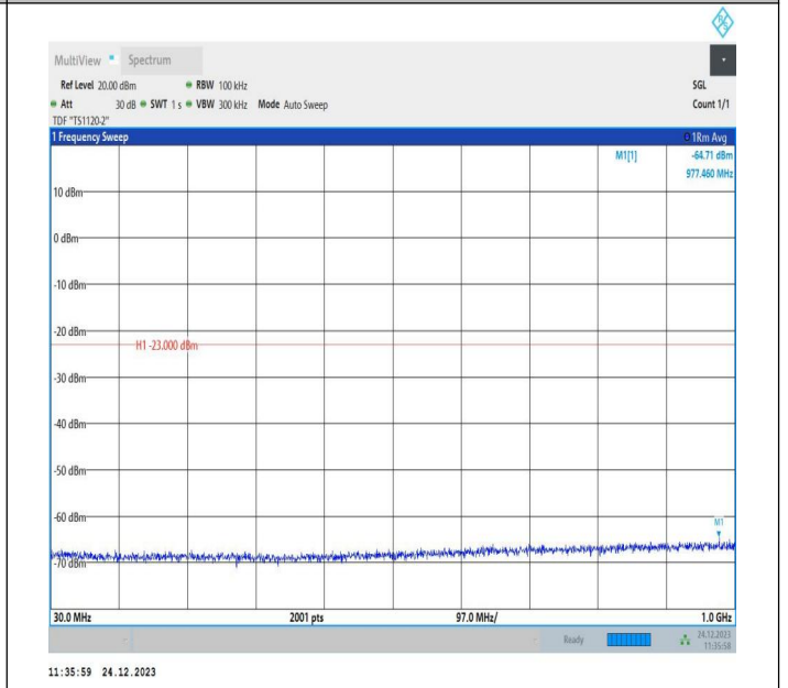
2-2-20MHz-20MHz-QPSK-QPSK-18801-18999-1RB#99-0RB#0 0-30~1000MHz-PASS
