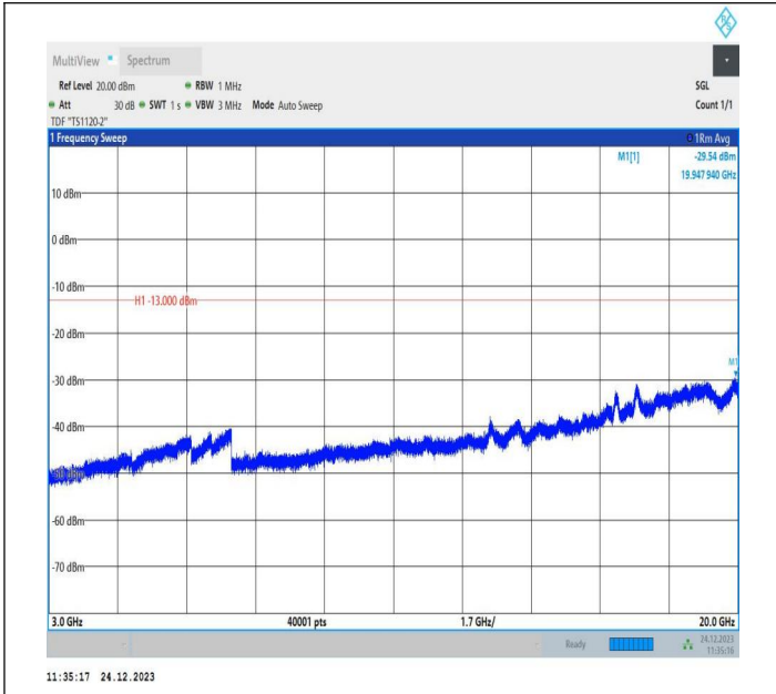
2-2-20MHz-20MHz-QPSK-QPSK-18801-18999-1RB#0-0RB#0 -3000~20000MHz-PASS
