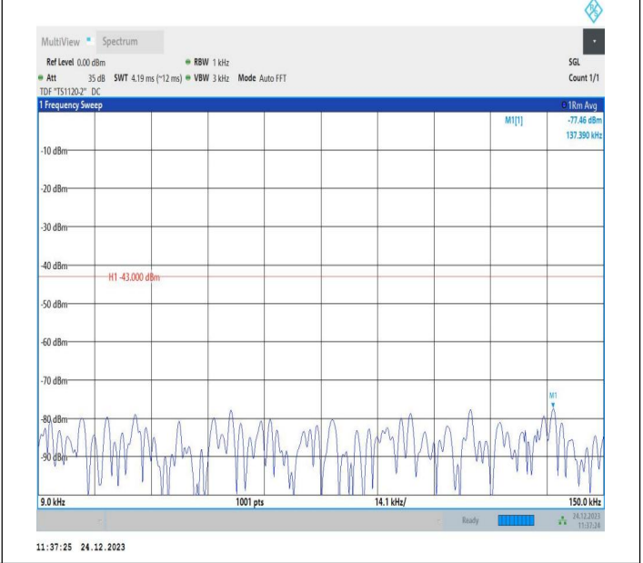
2-2-20MHz-20MHz-QPSK-QPSK-18801-18999-100RB#0-100 RB#0-0.009~0.15MHz-PASS
