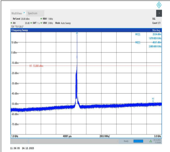
2-2-20MHz-20MHz-QPSK-QPSK-18801-18999-1RB#99-0RB# 0-1000~3000MHz-PASS
