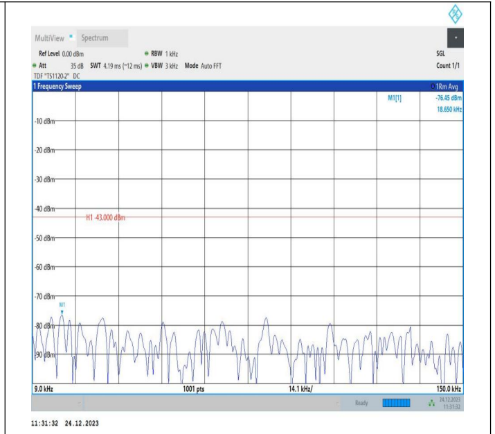
2-2-20MHz-20MHz-QPSK-QPSK-18700-18898-1RB#99-0RB#0 0-0.009~0.15MHz-PASS
