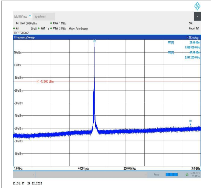
2-2-20MHz-20MHz-QPSK-QPSK-18700-18898-1RB#99-0RB# 0-1000~3000MHz-PASS
