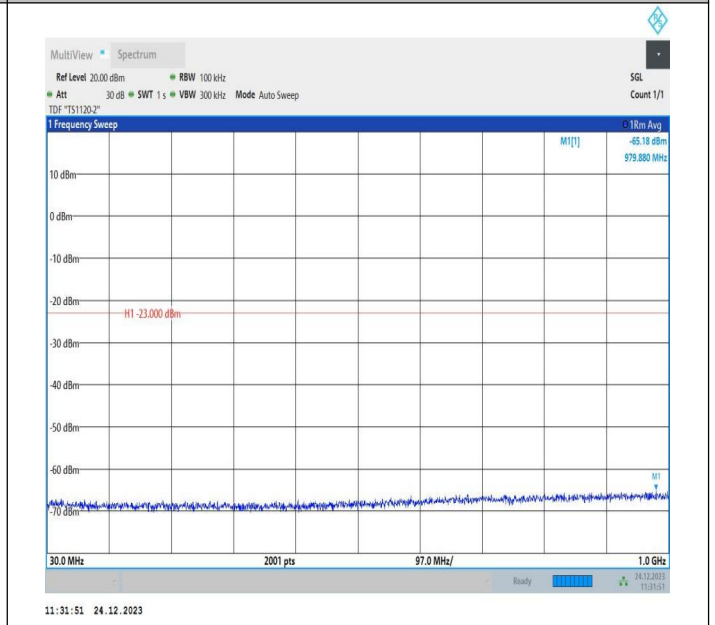
2-2-20MHz-20MHz-QPSK-QPSK-18700-18898-1RB#99-0RB#0 0-30~1000MHz-PASS
