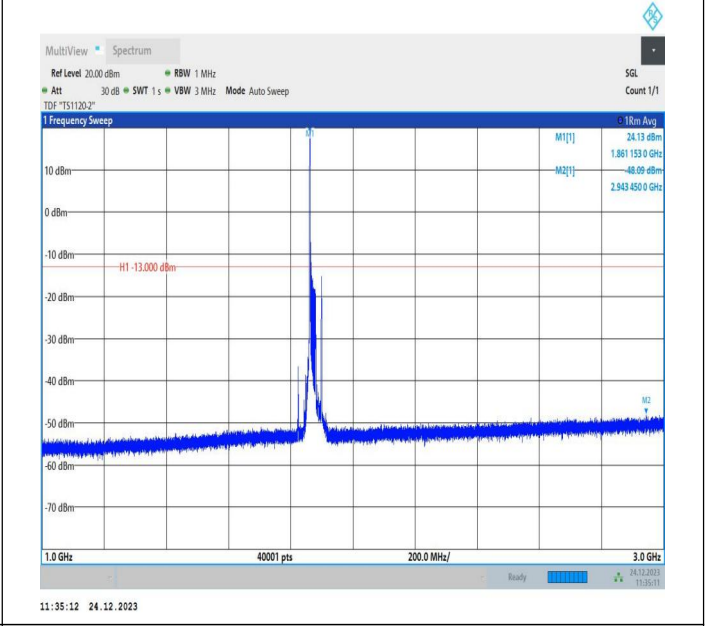
2-2-20MHz-20MHz-QPSK-QPSK-18801-18999-1RB#0-0RB#0 -1000~3000MHz-PASS
