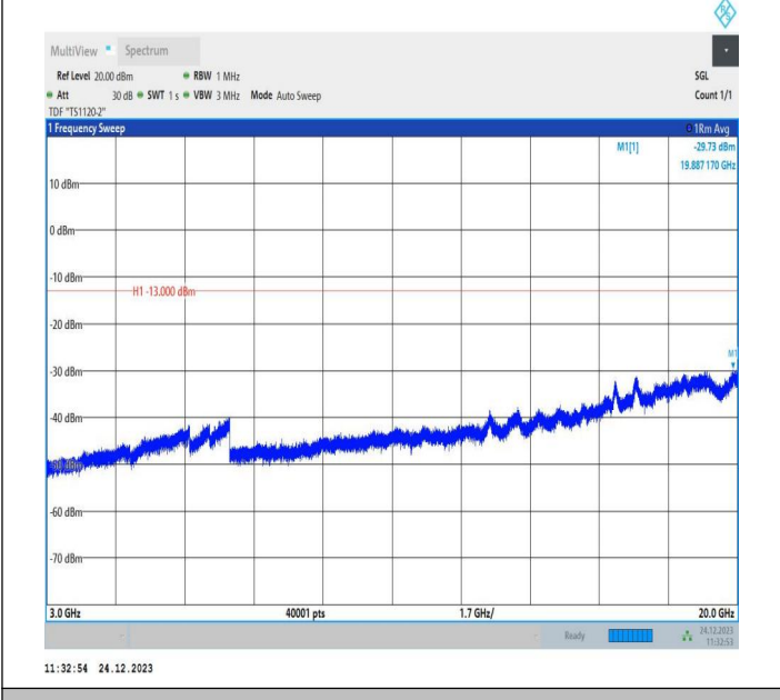
2-2-20MHz-20MHz-QPSK-QPSK-18700-18898-1RB#0-1RB#9 9-3000~20000MHz-PASS
