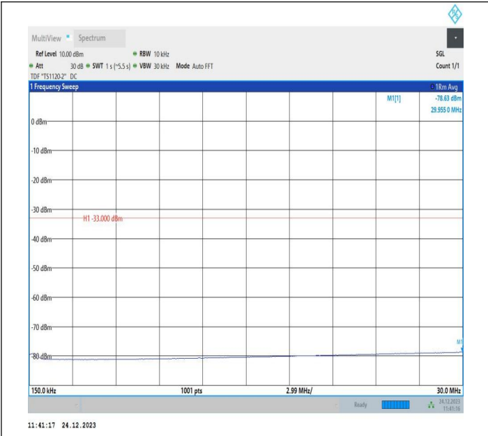
2-2-20MHz-20MHz-QPSK-QPSK-18902-19100-100RB#0-100 RB#0-0.15~30MHz-PASS
