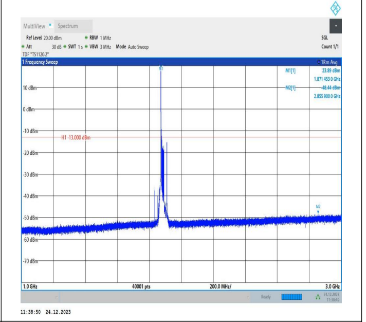
2-2-20MHz-20MHz-QPSK-QPSK-18902-19100-1RB#0-0RB#0 -1000~3000MHz-PASS
