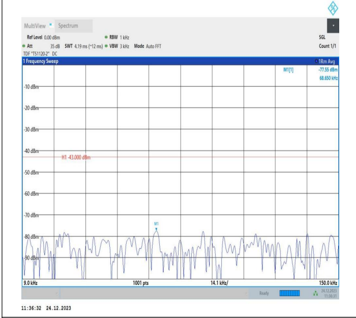
2-2-20MHz-20MHz-QPSK-QPSK-18801-18999-1RB#0-1RB#9 9-0.009~0.15MHz-PASS
