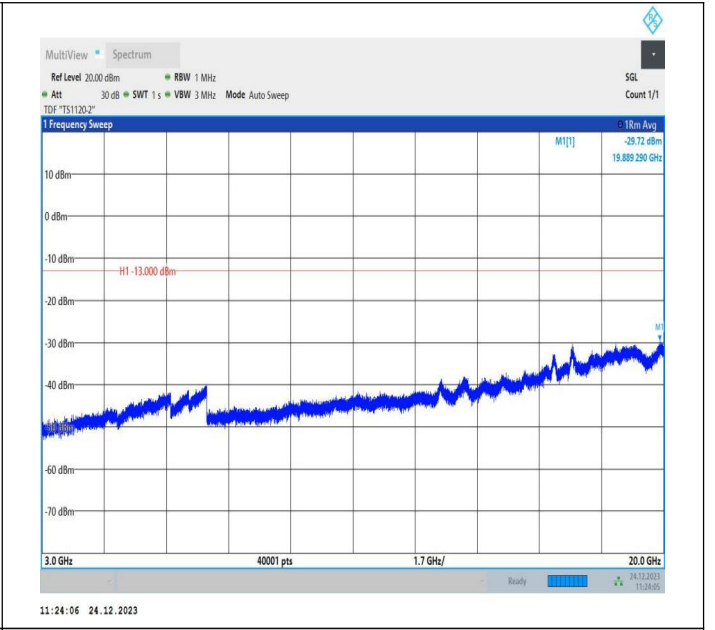
2-2-20MHz-15MHz-QPSK-QPSK-18826-18997-1RB#99-0RB# 0-3000~20000MHz-PASS
