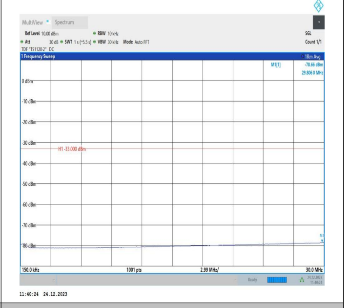
2-2-20MHz-20MHz-QPSK-QPSK-18902-19100-1RB#0-1RB#9 9-0.15~30MHz-PASS
