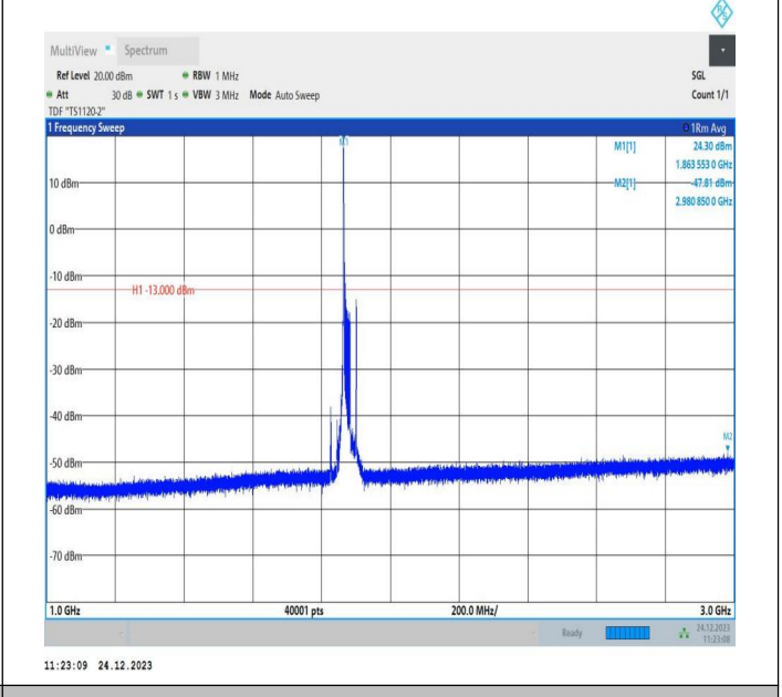
2-2-20MHz-15MHz-QPSK-QPSK-18826-18997-1RB#0-0RB#0 -1000~3000MHz-PASS
