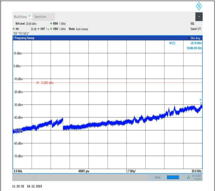
2-2-20MHz-20MHz-QPSK-QPSK-18700-18898-1RB#99-0RB# 0-3000~20000MHz-PASS
