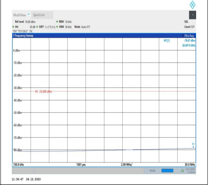
2-2-20MHz-20MHz-QPSK-QPSK-18801-18999-1RB#0-1RB#9 9-0.15~30MHz-PASS
