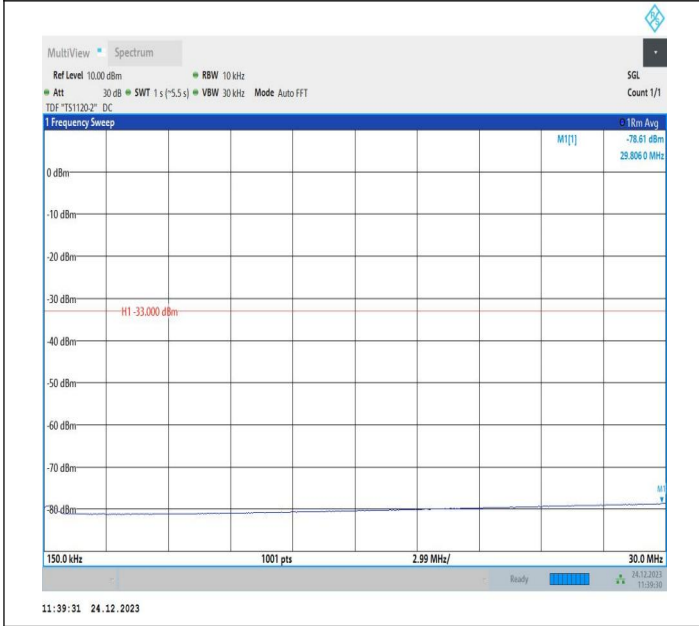
2-2-20MHz-20MHz-QPSK-QPSK-18902-19100-1RB#99-0RB#0 0-0.15~30MHz-PASS
