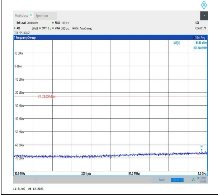
2-2-20MHz-20MHz-QPSK-QPSK-18700-18898-1RB#0-0RB#0 -30~1000MHz-PASS
