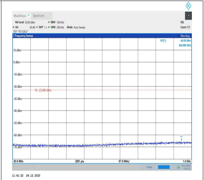
2-2-20MHz-20MHz-QPSK-QPSK-18902-19100-100RB#0-100 RB#0-30~1000MHz-PASS
