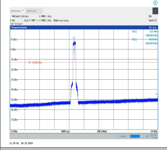
2-2-20MHz-20MHz-QPSK-QPSK-18700-18898-100RB#0-100 RB#0-1000~3000MHz-PASS
