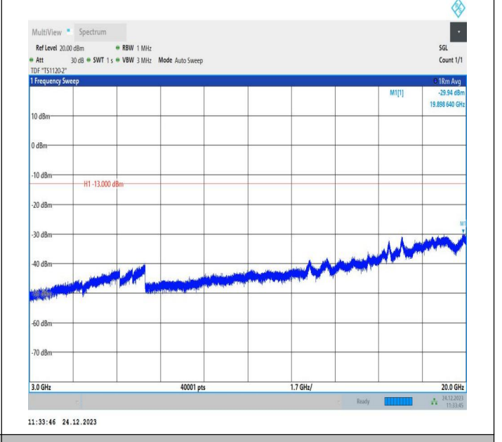
2-2-20MHz-20MHz-QPSK-QPSK-18700-18898-100RB#0-100 RB#0-3000~20000MHz-PASS
