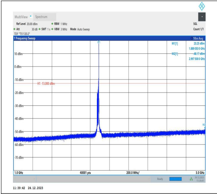
2-2-20MHz-20MHz-QPSK-QPSK-18902-19100-1RB#99-0RB# 0-1000~3000MHz-PASS
