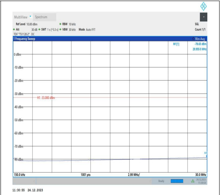
2-2-20MHz-20MHz-QPSK-QPSK-18700-18898-1RB#0-0RB#0 -0.15~30MHz-PASS
