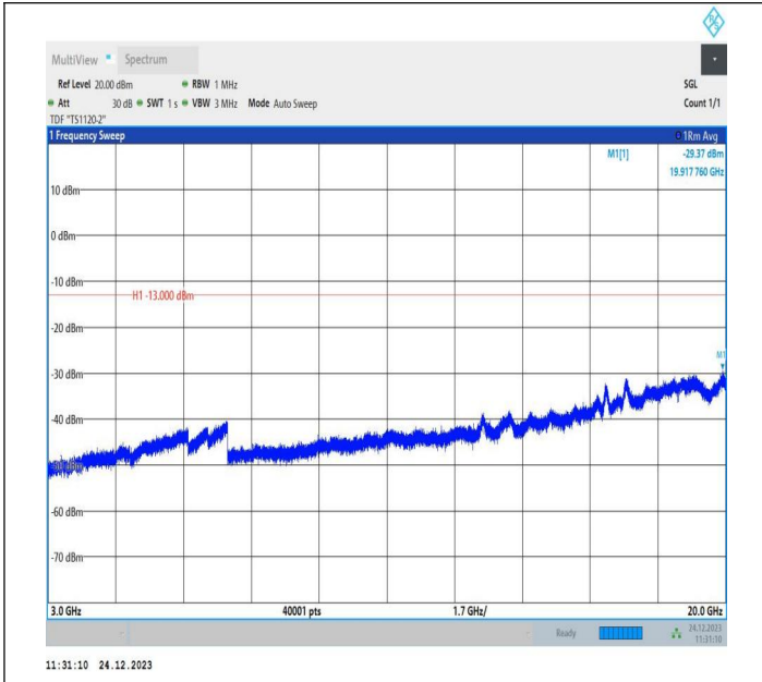
2-2-20MHz-20MHz-QPSK-QPSK-18700-18898-1RB#0-0RB#0 -3000~20000MHz-PASS
