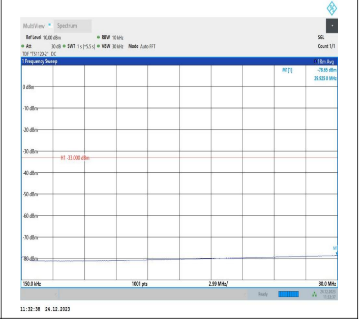
2-2-20MHz-20MHz-QPSK-QPSK-18700-18898-1RB#0-1RB#9 9-0.15~30MHz-PASS
