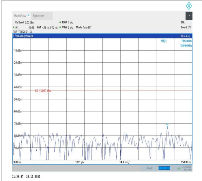
2-2-20MHz-20MHz-QPSK-QPSK-18801-18999-1RB#0-0RB#0 -0.009~0.15MHz-PASS
