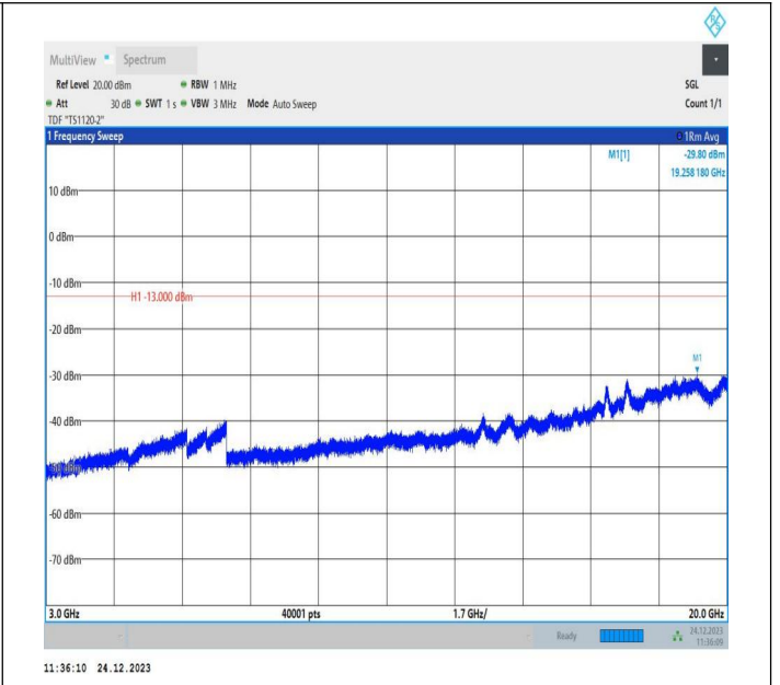
2-2-20MHz-20MHz-QPSK-QPSK-18801-18999-1RB#99-0RB# 0-3000~20000MHz-PASS
