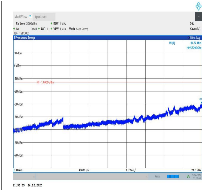
2-2-20MHz-20MHz-QPSK-QPSK-18902-19100-1RB#0-0RB#0 -3000~20000MHz-PASS
