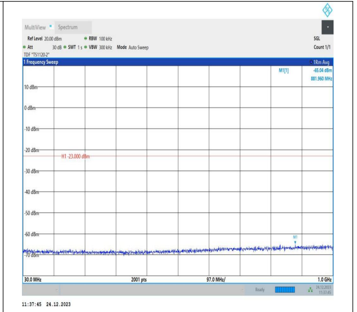
2-2-20MHz-20MHz-QPSK-QPSK-18801-18999-100RB#0-100 RB#0-30~1000MHz-PASS
