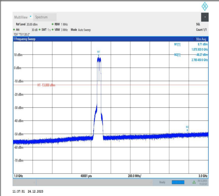
2-2-20MHz-20MHz-QPSK-QPSK-18801-18999-100RB#0-100 RB#0-1000~3000MHz-PASS
