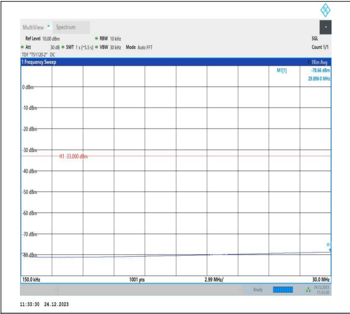
2-2-20MHz-20MHz-QPSK-QPSK-18700-18898-100RB#0-100 RB#0-0.15~30MHz-PASS
