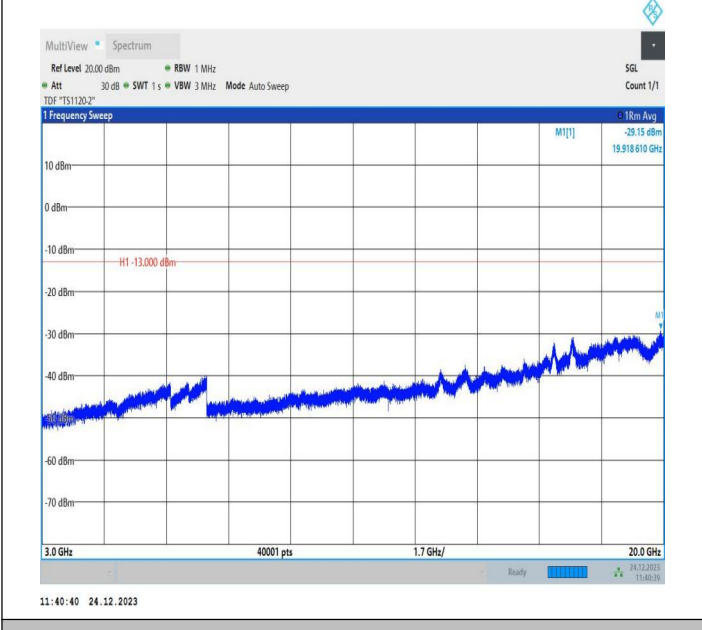
2-2-20MHz-20MHz-QPSK-QPSK-18902-19100-1RB#0-1RB#9 9-3000~20000MHz-PASS
