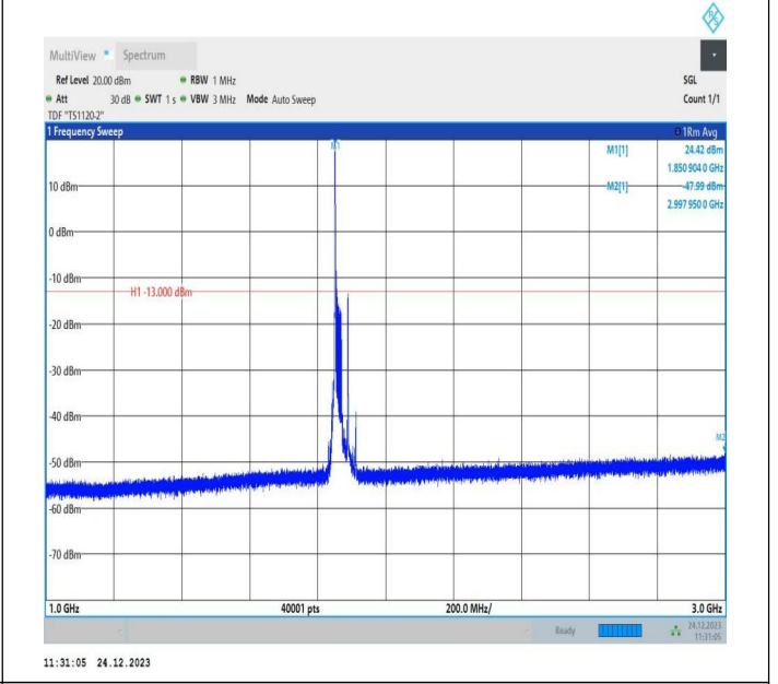
2-2-20MHz-20MHz-QPSK-QPSK-18700-18898-1RB#0-0RB#0 -1000~3000MHz-PASS
