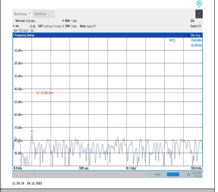
2-2-20MHz-20MHz-QPSK-QPSK-18700-18898-100RB#0-100 RB#0-0.009~0.15MHz-PASS
