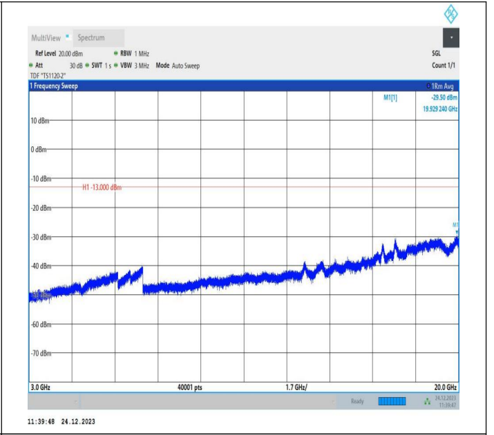
2-2-20MHz-20MHz-QPSK-QPSK-18902-19100-1RB#99-0RB# 0-3000~20000MHz-PASS
