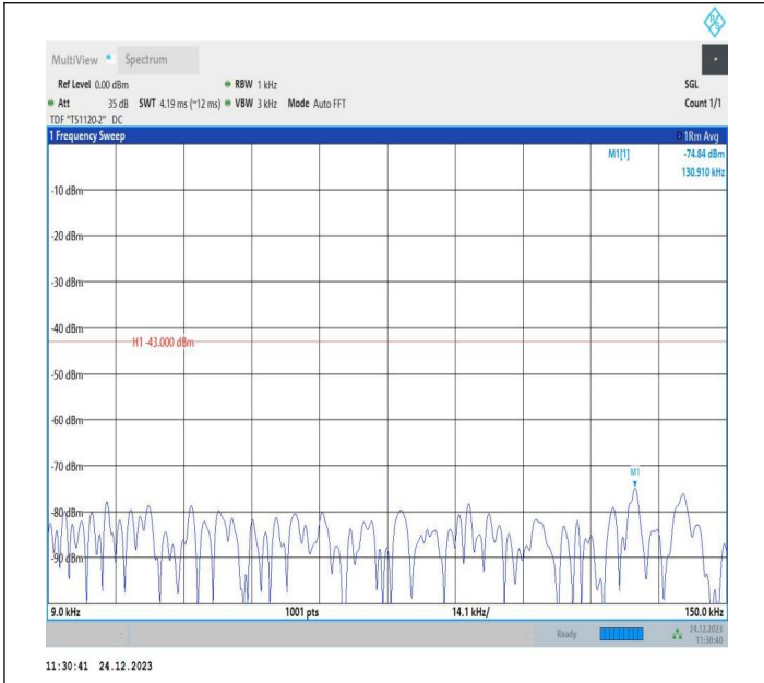
2-2-20MHz-20MHz-QPSK-QPSK-18700-18898-1RB#0-0RB#0 -0.009~0.15MHz-PASS
