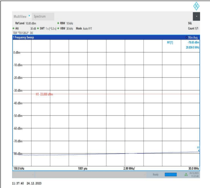
2-2-20MHz-20MHz-QPSK-QPSK-18801-18999-100RB#0-100 RB#0-0.15~30MHz-PASS
