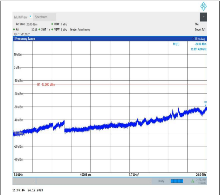
2-2-20MHz-5MHz-QPSK-QPSK-18700-18817-1RB#99-0RB#0 -3000~20000MHz-PASS
