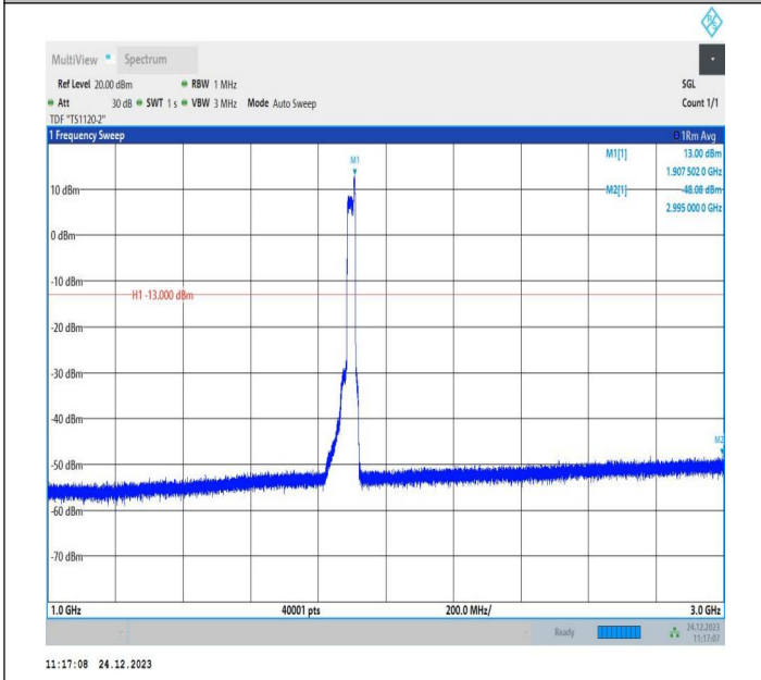
2-2-20MHz-5MHz-QPSK-QPSK-19050-19167-100RB#0-25RB #0-1000~3000MHz-PASS
