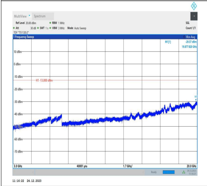
2-2-20MHz-5MHz-QPSK-QPSK-19050-19167-1RB#0-1RB#24 -3000~20000MHz-PASS
