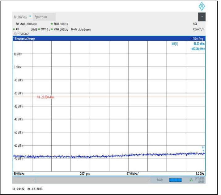
2-2-20MHz-5MHz-QPSK-QPSK-18700-18817-100RB#0-25RB #0-30~1000MHz-PASS
