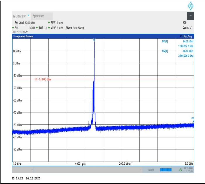
2-2-20MHz-5MHz-QPSK-QPSK-19050-19167-1RB#99-0RB#0 -1000~3000MHz-PASS
