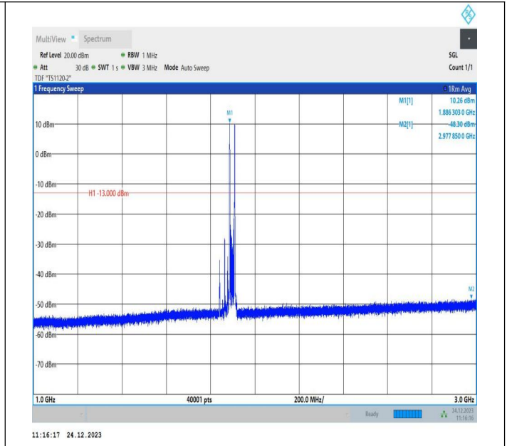
2-2-20MHz-5MHz-QPSK-QPSK-19050-19167-1RB#0-1RB#24 -1000~3000MHz-PASS
