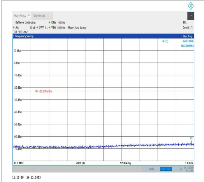
2-2-20MHz-5MHz-QPSK-QPSK-18875-18992-1RB#0-1RB#24 -30~1000MHz-PASS
