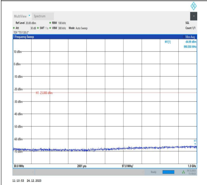
2-2-20MHz-5MHz-QPSK-QPSK-18875-18992-1RB#0-0RB#0-30~1000MHz-PASS
