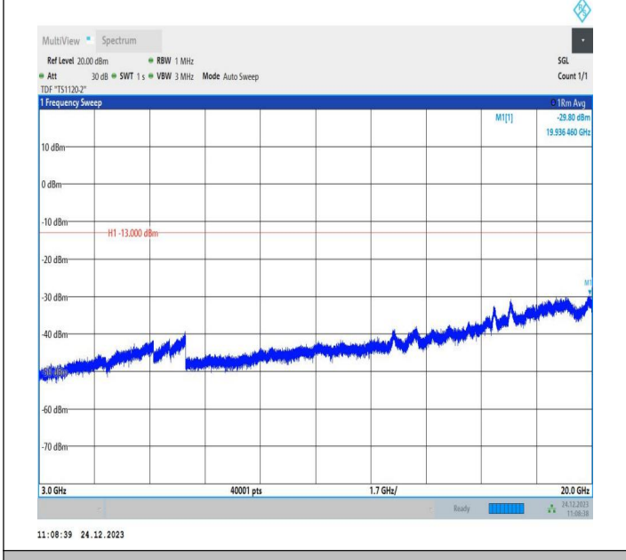
2-2-20MHz-5MHz-QPSK-QPSK-18700-18817-1RB#0-1RB#24 -3000~20000MHz-PASS
