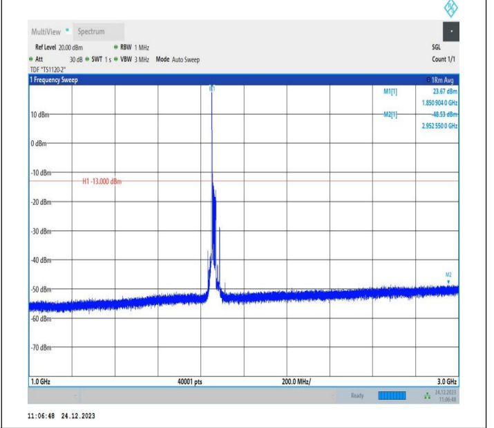
2-2-20MHz-5MHz-QPSK-QPSK-18700-18817-1RB#0-0RB#0-1000~3000MHz-PASS
