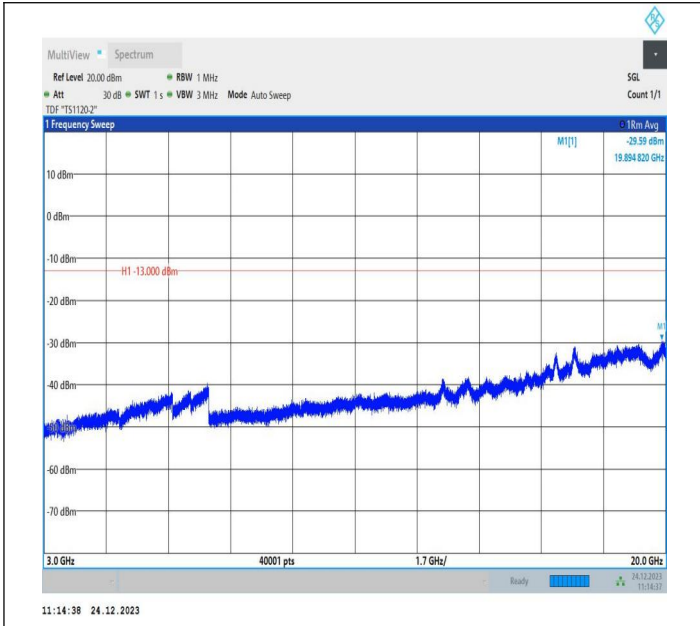
2-2-20MHz-5MHz-QPSK-QPSK-19050-19167-1RB#0-0RB#0-3000~20000MHz-PASS
