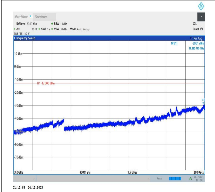
2-2-20MHz-5MHz-QPSK-QPSK-18875-18992-1RB#0-1RB#24 -3000~20000MHz-PASS
