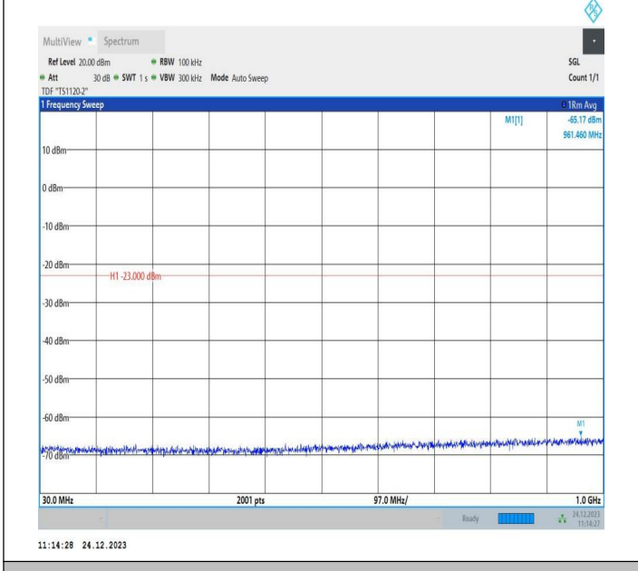
2-2-20MHz-5MHz-QPSK-QPSK-19050-19167-1RB#0-0RB#0-30~1000MHz-PASS
