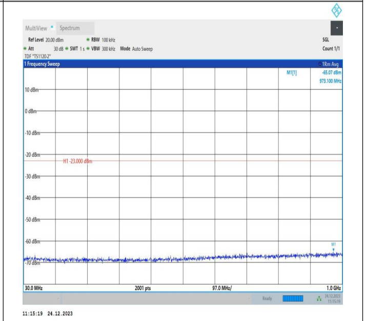
2-2-20MHz-5MHz-QPSK-QPSK-19050-19167-1RB#99-0RB#0-30~1000MHz-PASS
