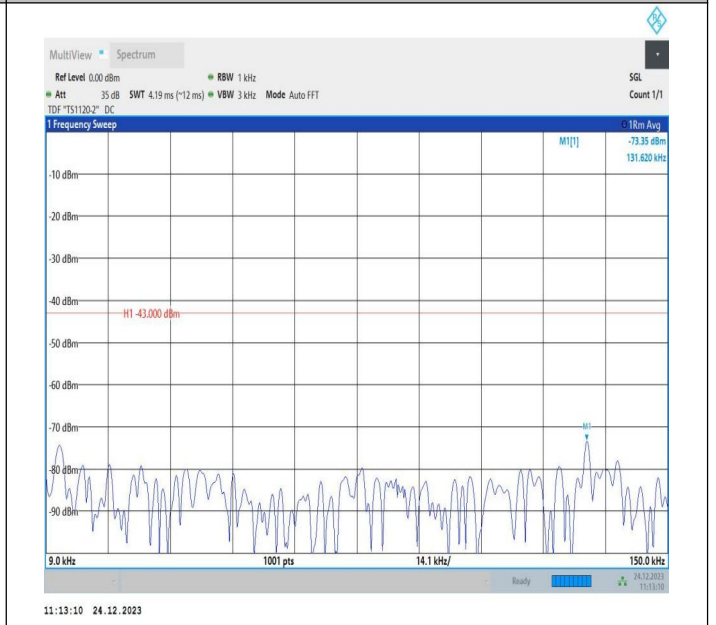
2-2-20MHz-5MHz-QPSK-QPSK-18875-18992-100RB#0-25RB #0-0.009~0.15MHz-PASS
