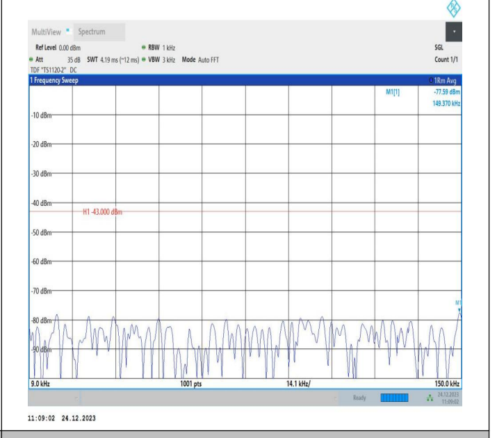
2-2-20MHz-5MHz-QPSK-QPSK-18700-18817-100RB#0-25RB #0-0.009~0.15MHz-PASS
