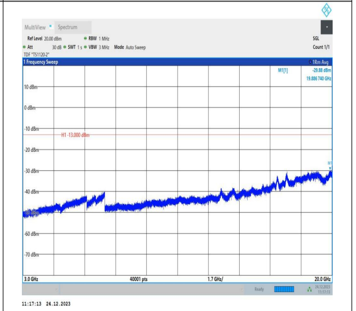
2-2-20MHz-5MHz-QPSK-QPSK-19050-19167-100RB#0-25RB #0-3000~20000MHz-PASS
