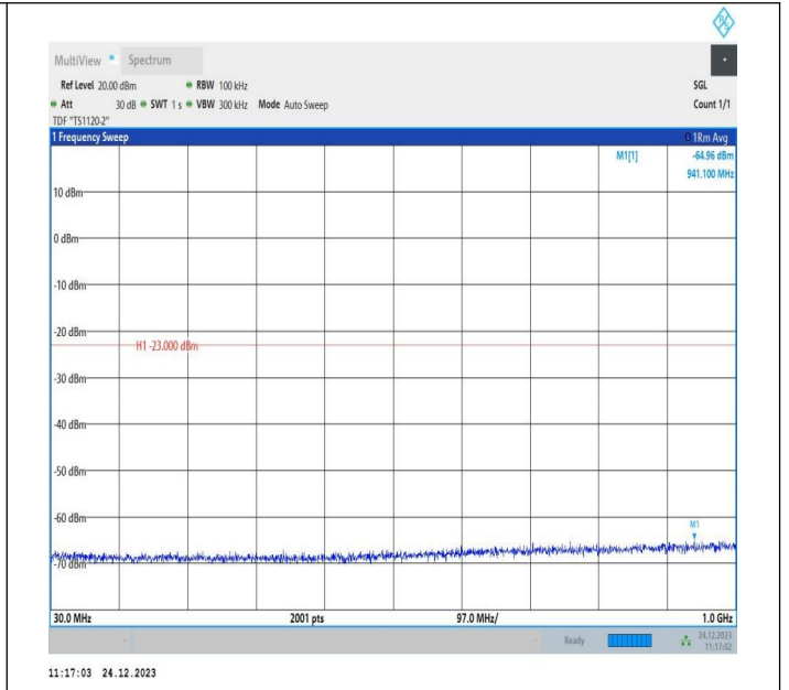
2-2-20MHz-5MHz-QPSK-QPSK-19050-19167-100RB#0-25RB #0-30~1000MHz-PASS
