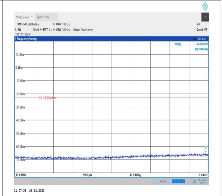
2-2-20MHz-5MHz-QPSK-QPSK-18700-18817-1RB#99-0RB#0-30~1000MHz-PASS
