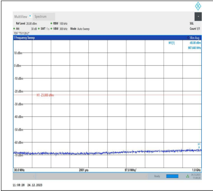
2-2-20MHz-5MHz-QPSK-QPSK-18700-18817-1RB#0-1RB#24 -30~1000MHz-PASS
