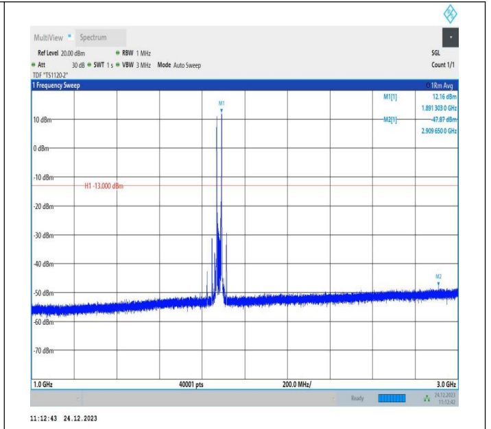
2-2-20MHz-5MHz-QPSK-QPSK-18875-18992-1RB#0-1RB#24 -1000~3000MHz-PASS
