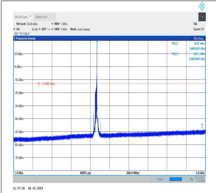
2-2-20MHz-5MHz-QPSK-QPSK-18700-18817-1RB#99-0RB#0 -1000~3000MHz-PASS
