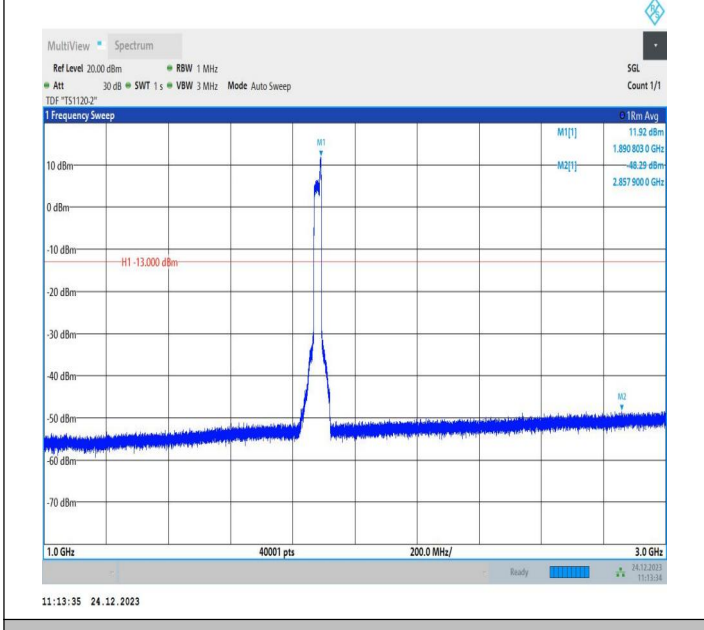
2-2-20MHz-5MHz-QPSK-QPSK-18875-18992-100RB#0-25RB #0-1000~3000MHz-PASS
