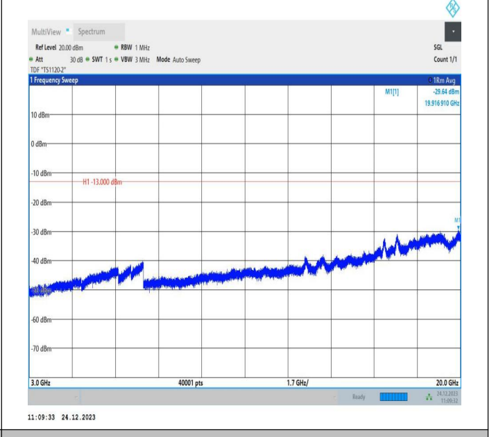
2-2-20MHz-5MHz-QPSK-QPSK-18700-18817-100RB#0-25RB #0-3000~20000MHz-PASS
