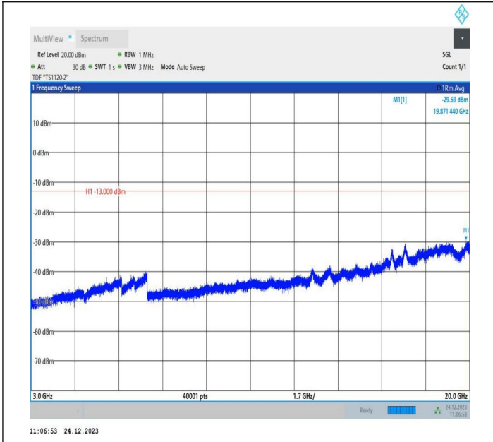
2-2-20MHz-5MHz-QPSK-QPSK-18700-18817-1RB#0-0RB#0-3000~20000MHz-PASS
