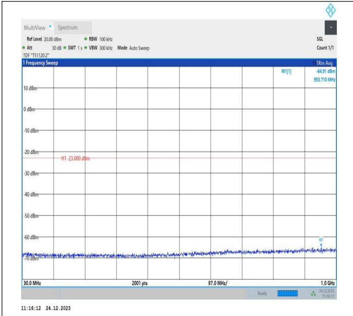
2-2-20MHz-5MHz-QPSK-QPSK-19050-19167-1RB#0-1RB#24 -30~1000MHz-PASS
