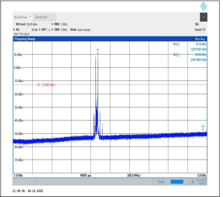
2-2-20MHz-5MHz-QPSK-QPSK-18700-18817-1RB#0-1RB#24 -1000~3000MHz-PASS
