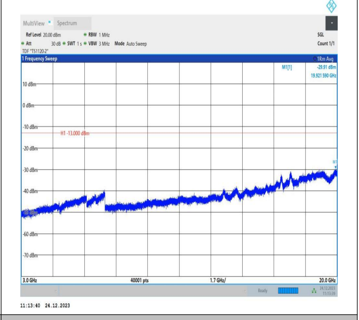
2-2-20MHz-5MHz-QPSK-QPSK-18875-18992-100RB#0-25RB #0-3000~20000MHz-PASS
