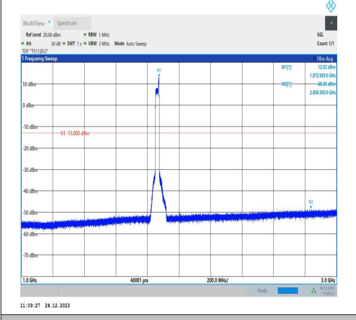
2-2-20MHz-5MHz-QPSK-QPSK-18700-18817-100RB#0-25RB #0-1000~3000MHz-PASS
