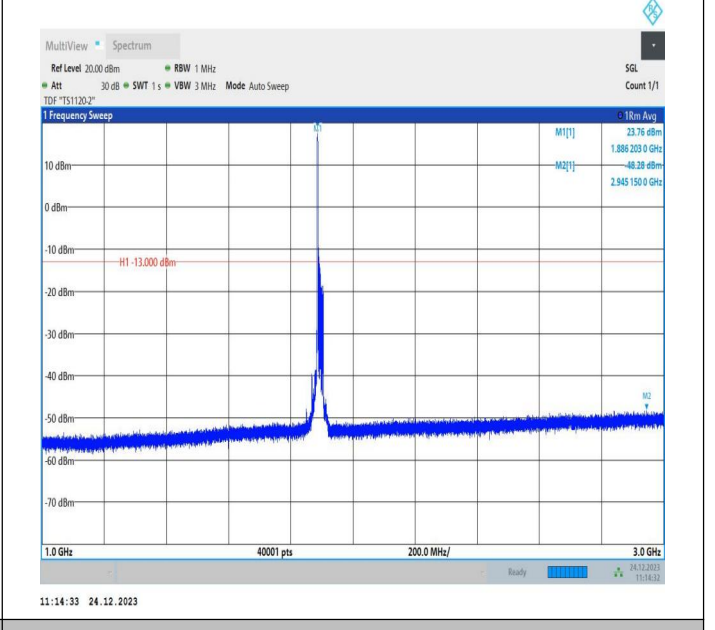
2-2-20MHz-5MHz-QPSK-QPSK-19050-19167-1RB#0-0RB#0-1000~3000MHz-PASS
