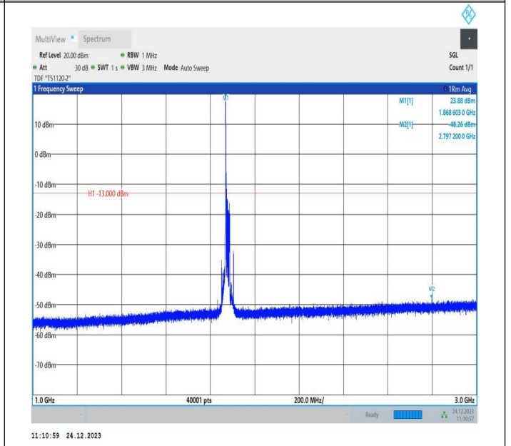
2-2-20MHz-5MHz-QPSK-QPSK-18875-18992-1RB#0-0RB#0-1000~3000MHz-PASS
