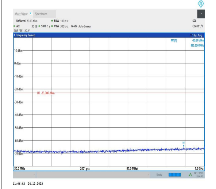
2-2-20MHz-5MHz-QPSK-QPSK-18700-18817-1RB#0-0RB#0-30~1000MHz-PASS
