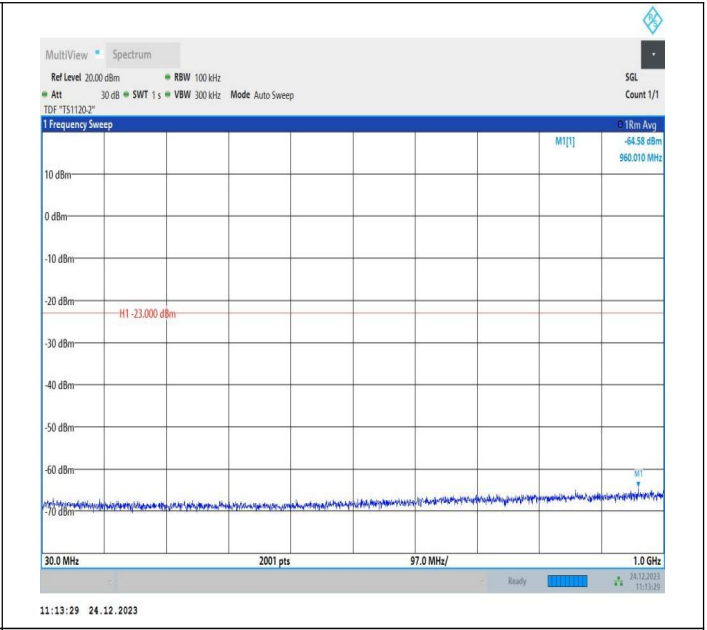
2-2-20MHz-5MHz-QPSK-QPSK-18875-18992-100RB#0-25RB #0-30~1000MHz-PASS
