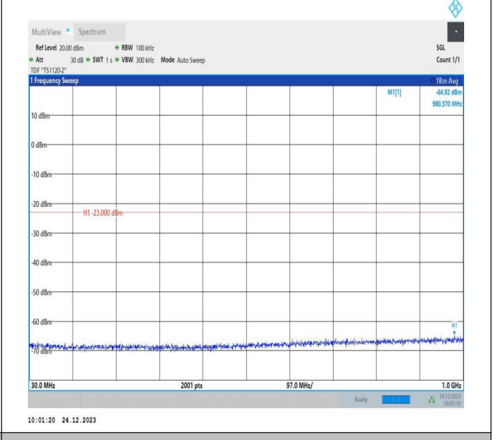
2-2-15MHz-10MHz-QPSK-QPSK-18851-18971-1RB#74-0RB# 0-30~1000MHz-PASS
