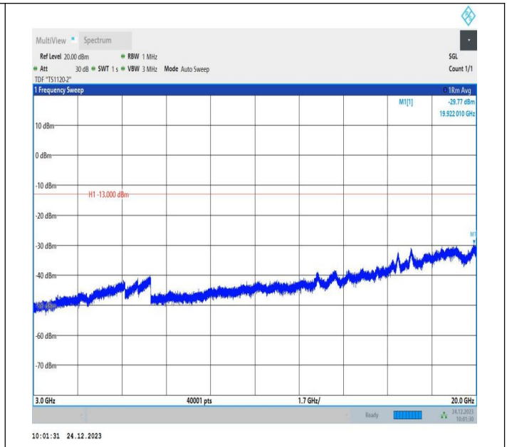
2-2-15MHz-10MHz-QPSK-QPSK-18851-18971-1RB#74-0RB# 0-3000~20000MHz-PASS
