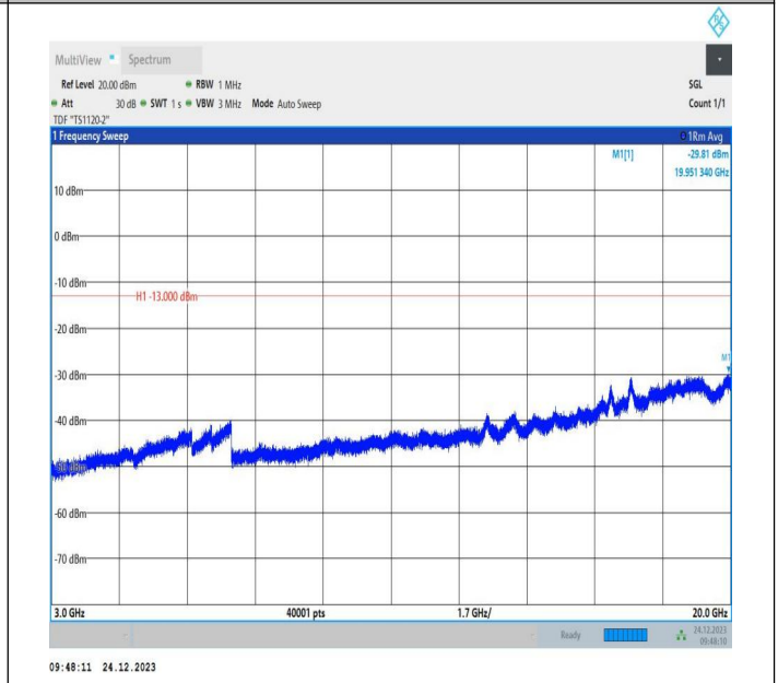
2-2-20MHz-10MHz-QPSK-QPSK-18851-18995-1RB#0-ORB#0 -3000~20000MHz-PASS
