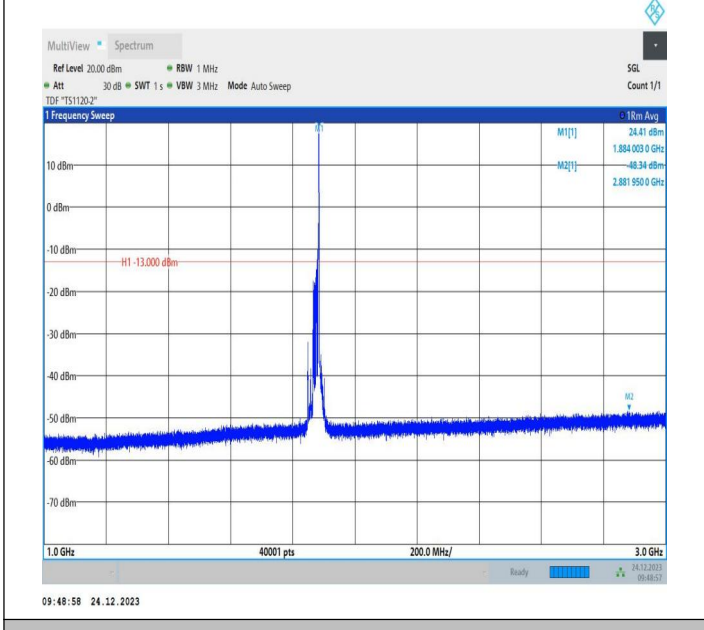
2-2-20MHz-10MHz-QPSK-QPSK-18851-18995-1RB#99-0RB# 0-1000~3000MHz-PASS
