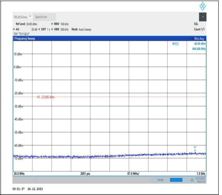
2-2-20MHz-10MHz-QPSK-QPSK-19001-19145-1RB#0-0RB#0 -30~1000MHz-PASS
