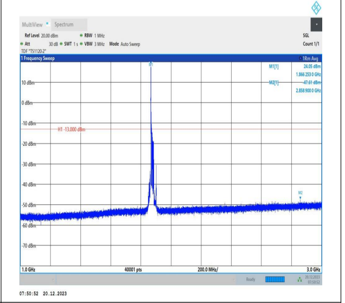
2-2-20MHz-10MHz-16QAM-16QAM-18851-18995-1RB#0-ORB #0-1000~3000MHz-PASS
