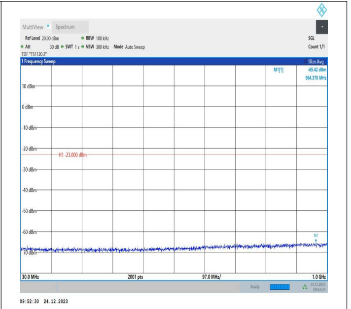
2-2-20MHz-10MHz-QPSK-QPSK-19001-19145-1RB#99-0RB# 0-30~1000MHz-PASS
