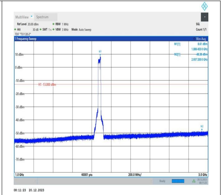
2-2-20MHz-10MHz-16QAM-16QAM-18851-18995-100RB#0-4 ORB#0-1000~3000MHz-PASS
