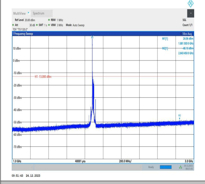
2-2-20MHz-10MHz-QPSK-QPSK-19001-19145-1RB#0-0RB#0 -1000~3000MHz-PASS
