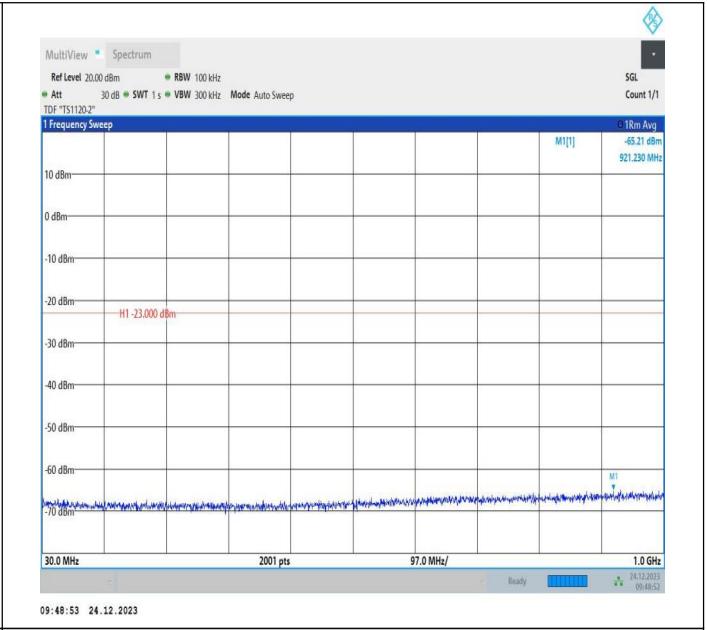
2-2-20MHz-10MHz-QPSK-QPSK-18851-18995-1RB#99-0RB# 0-30~1000MHz-PASS
