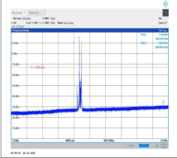
2-2-20MHz-10MHz-QPSK-QPSK-18851-18995-1RB#0-1RB#4 9-1000~3000MHz-PASS
