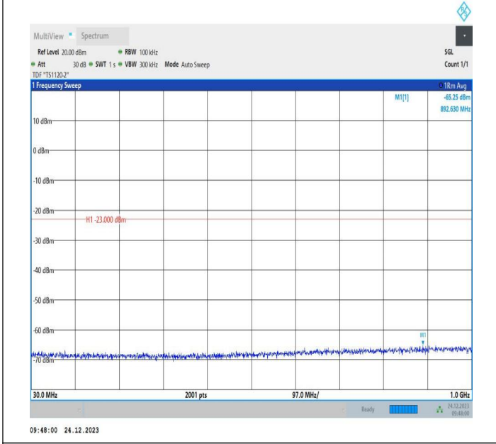
2-2-20MHz-10MHz-QPSK-QPSK-18851-18995-1RB#0-0RB#0 -30~1000MHz-PASS
