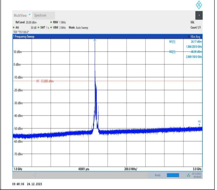
2-2-20MHz-10MHz-QPSK-QPSK-18851-18995-1RB#0-0RB#0 -1000~3000MHz-PASS
