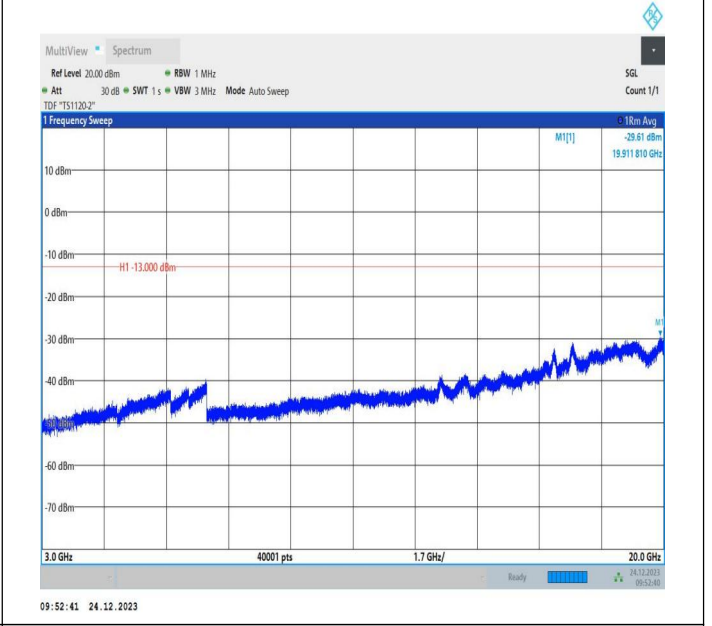
2-2-20MHz-10MHz-QPSK-QPSK-19001-19145-1RB#99-0RB# 0-3000~20000MHz-PASS
