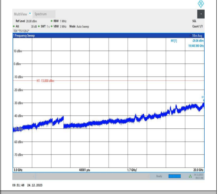
2-2-20MHz-10MHz-QPSK-QPSK-19001-19145-1RB#0-0RB#0 -3000~20000MHz-PASS
