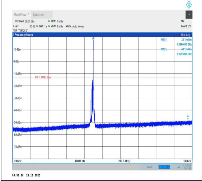
2-2-20MHz-10MHz-QPSK-QPSK-19001-19145-1RB#99-0RB# 0-1000~3000MHz-PASS
