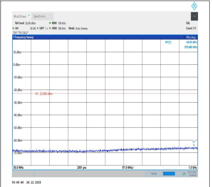
2-2-20MHz-10MHz-QPSK-QPSK-18851-18995-1RB#0-1RB#4 9-30~1000MHz-PASS
