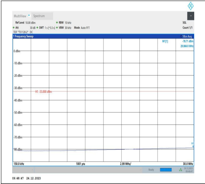
2-2-20MHz-10MHz-QPSK-QPSK-18851-18995-1RB#99-0RB# 0-0.15~30MHz-PASS
