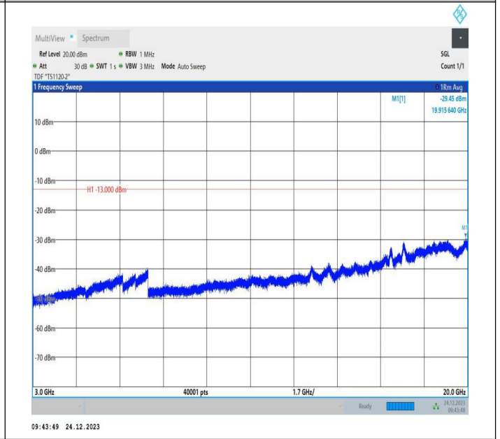
2-2-20MHz-10MHz-QPSK-QPSK-18700-18844-1RB#0-0RB#0 -3000~20000MHz-PASS
