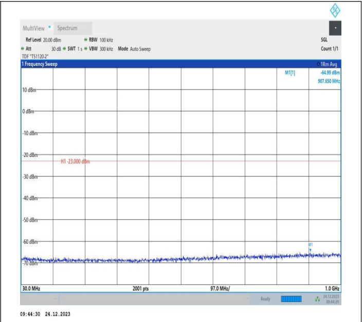
2-2-20MHz-10MHz-QPSK-QPSK-18700-18844-1RB#99-0RB# 0-30~1000MHz-PASS
