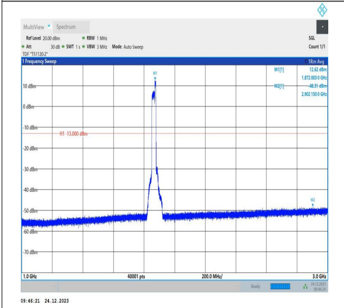
2-2-20MHz-10MHz-QPSK-QPSK-18700-18844-100RB#0-40R B#0-1000~3000MHz-PASS
