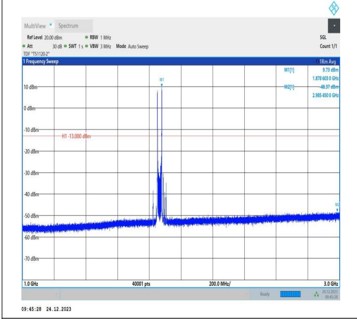
2-2-20MHz-10MHz-QPSK-QPSK-18700-18844-1RB#0-1RB#49-1000~3000MHz-PASS
