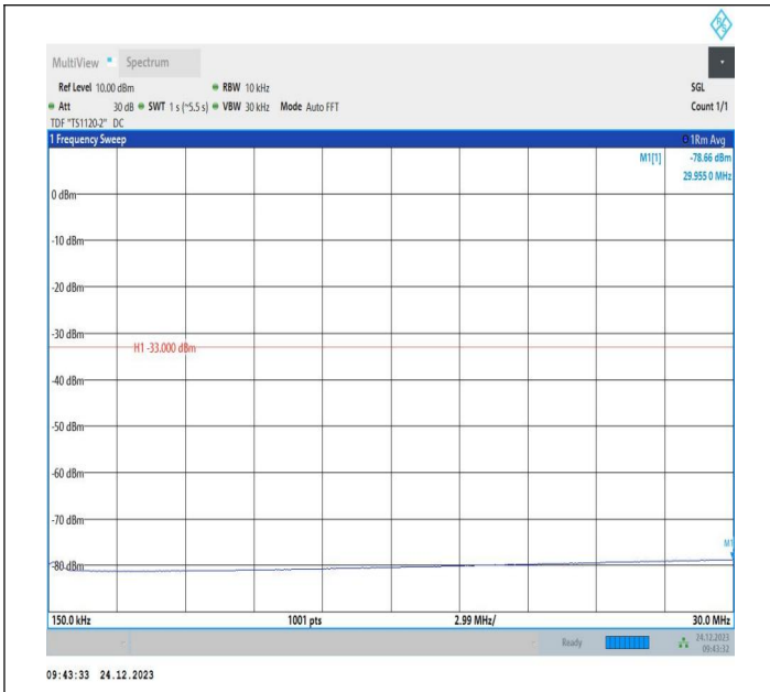
2-2-20MHz-10MHz-QPSK-QPSK-18700-18844-1RB#0-0RB#0 -0.15~30MHz-PASS
