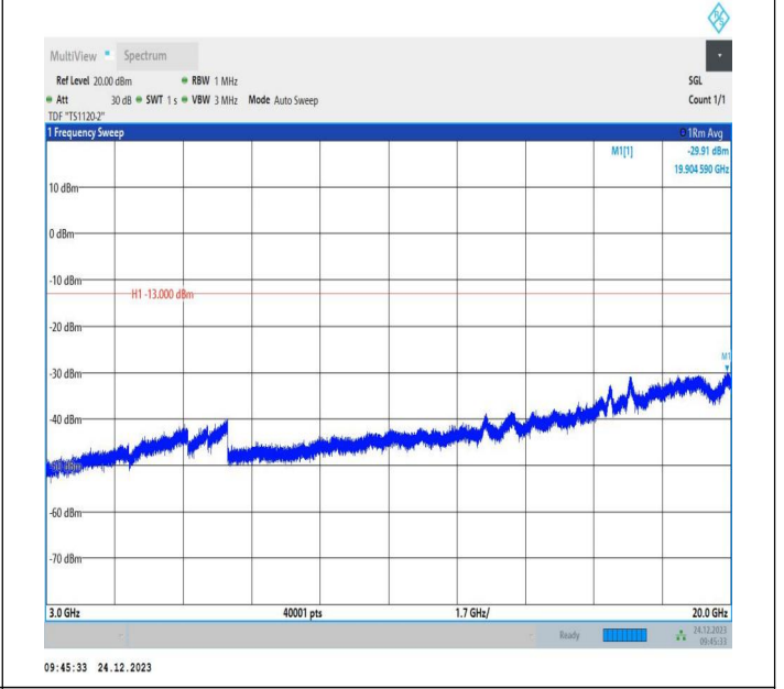
2-2-20MHz-10MHz-QPSK-QPSK-18700-18844-1RB#0-1RB#49-3000~20000MHz-PASS
