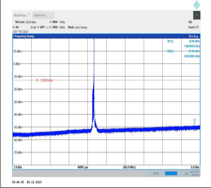
2-2-20MHz-10MHz-QPSK-QPSK-18700-18844-1RB#99-0RB# 0-1000~3000MHz-PASS
