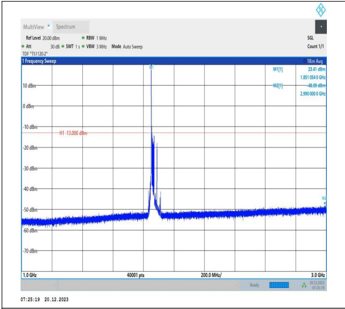
2-2-20MHz-10MHz-16QAM-16QAM-18700-18844-1RB#0-ORB #0-1000~3000MHz-PASS
