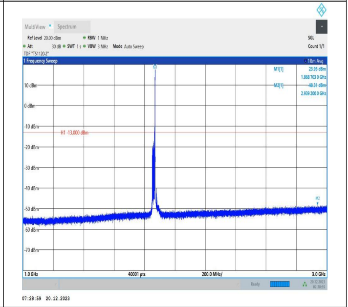
2-2-20MHz-10MHz-16QAM-16QAM-18700-18844-1RB#99-0R B#0-1000~3000MHz-PASS
