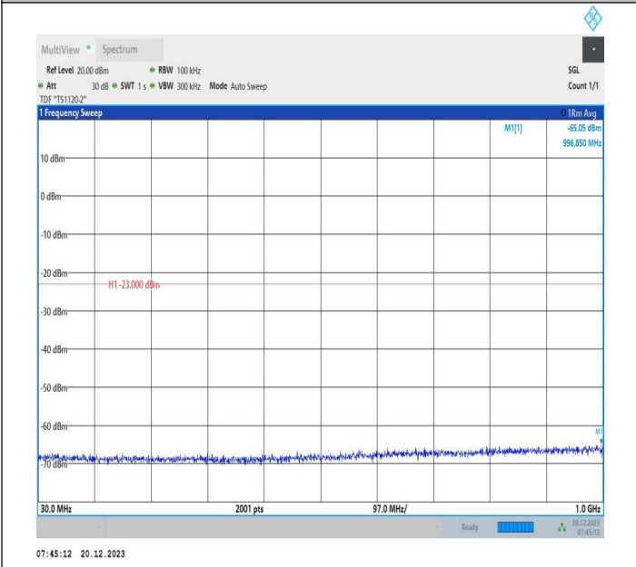
2-2-20MHz-10MHz-16QAM-16QAM-18700-18844-100RB#0-4 ORB#0-30~1000MHz-PASS
