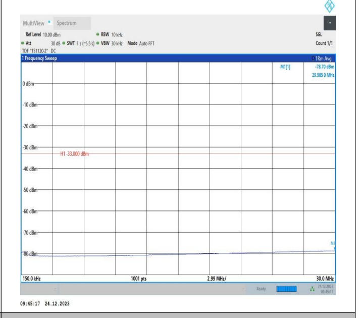
2-2-20MHz-10MHz-QPSK-QPSK-18700-18844-1RB#0-1RB#4 9-0.15~30MHz-PASS
