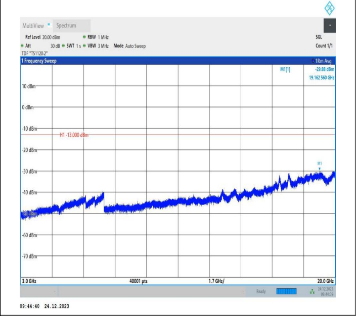
2-2-20MHz-10MHz-QPSK-QPSK-18700-18844-1RB#99-0RB# 0-3000~20000MHz-PASS
