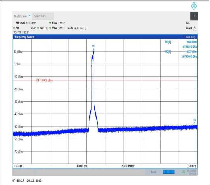
2-2-20MHz-10MHz-16QAM-16QAM-18700-18844-100RB#0-4 ORB#0-1000~3000MHz-PASS
