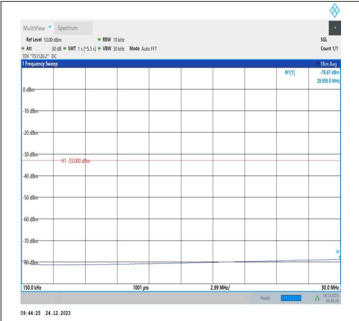
2-2-20MHz-10MHz-QPSK-QPSK-18700-18844-1RB#99-0RB# 0-0.15~30MHz-PASS
