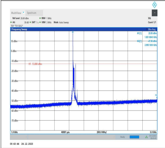
2-2-20MHz-10MHz-QPSK-QPSK-18700-18844-1RB#0-0RB#0 -1000~3000MHz-PASS
