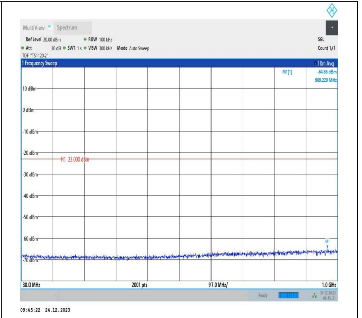
2-2-20MHz-10MHz-QPSK-QPSK-18700-18844-1RB#0-1RB#49-30~1000MHz-PASS
