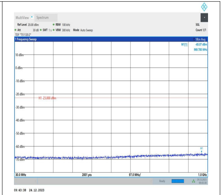
2-2-20MHz-10MHz-QPSK-QPSK-18700-18844-1RB#0-0RB#0 -30~1000MHz-PASS
