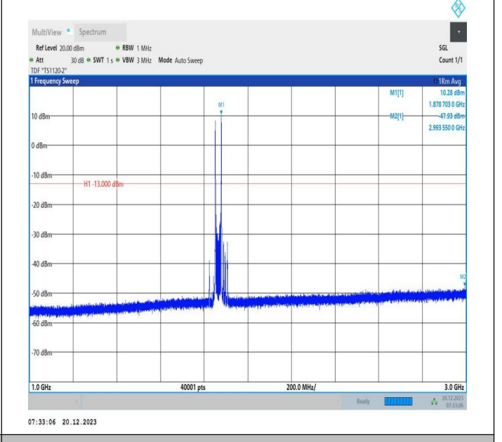
2-2-20MHz-10MHz-16QAM-16QAM-18700-18844-1RB#0-1RB #49-1000~3000MHz-PASS
