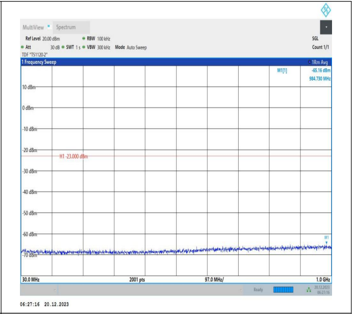
2-2-10MHz-20MHz-QPSK-QPSK-18806-18950-1RB#49-0RB# 0-30~1000MHz-PASS
