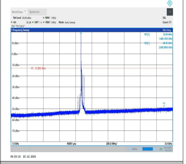
2-2-10MHz-20MHz-QPSK-QPSK-18806-18950-1RB#0-0RB#0 -1000~3000MHz-PASS
