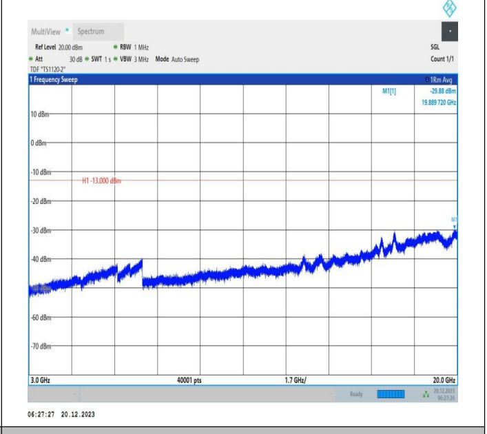
2-2-10MHz-20MHz-QPSK-QPSK-18806-18950-1RB#49-0RB# 0-3000~20000MHz-PASS
