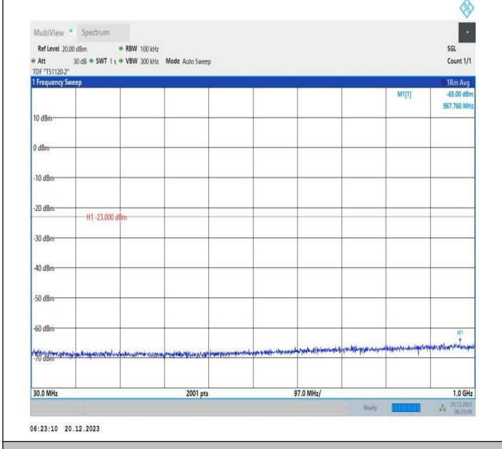
2-2-10MHz-20MHz-QPSK-QPSK-18806-18950-1RB#0-0RB#0 -30~1000MHz-PASS
