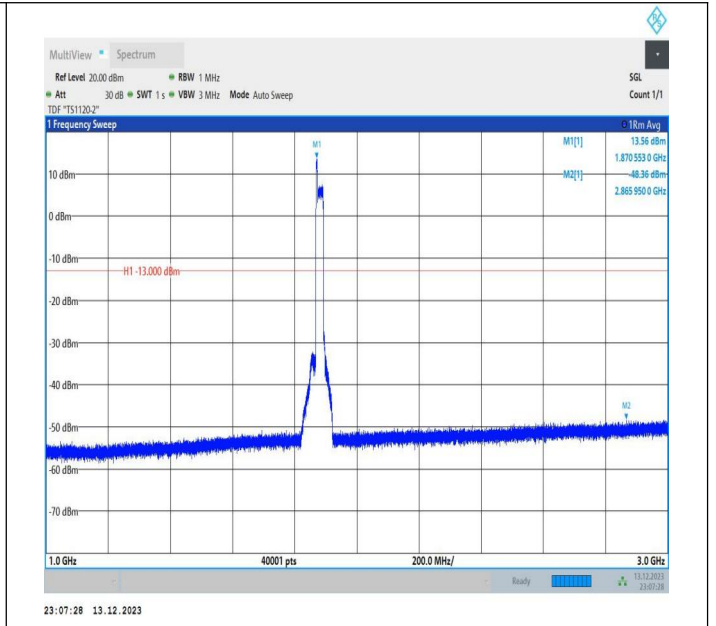
2-2-5MHz-20MHz-QPSK-QPSK-18808-18925-25RB#0-100RB #0-1000~3000MHz-PASS
