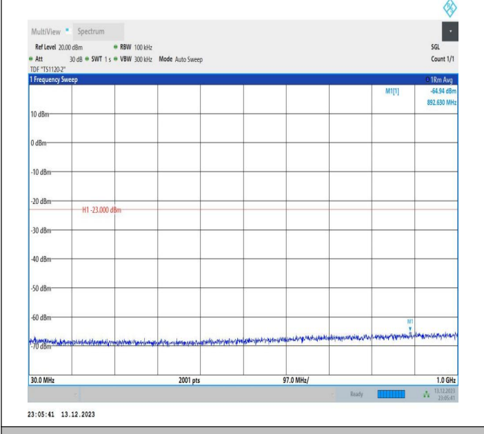
2-2-5MHz-20MHz-QPSK-QPSK-18808-18925-1RB#0-1RB#99 -30~1000MHz-PASS
