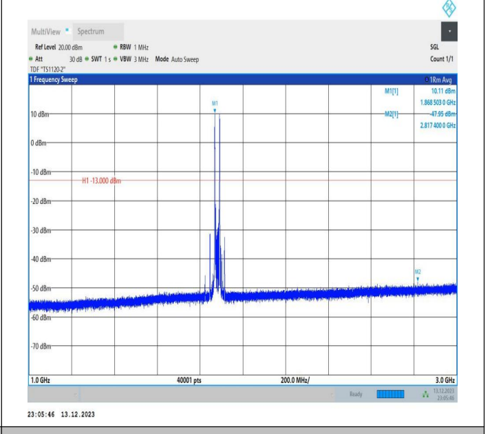
2-2-5MHz-20MHz-QPSK-QPSK-18808-18925-1RB#0-1RB#99 -1000~3000MHz-PASS
