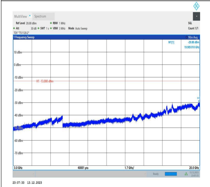
2-2-5MHz-20MHz-QPSK-QPSK-18808-18925-25RB#0-100RB #0-3000~20000MHz-PASS
