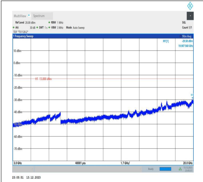
2-2-5MHz-20MHz-QPSK-QPSK-18808-18925-1RB#0-1RB#99 -3000~20000MHz-PASS
