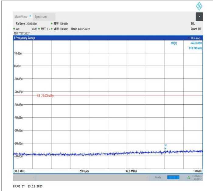
2-2-5MHz-20MHz-QPSK-QPSK-18808-18925-1RB#24-0RB#0 -30~1000MHz-PASS
