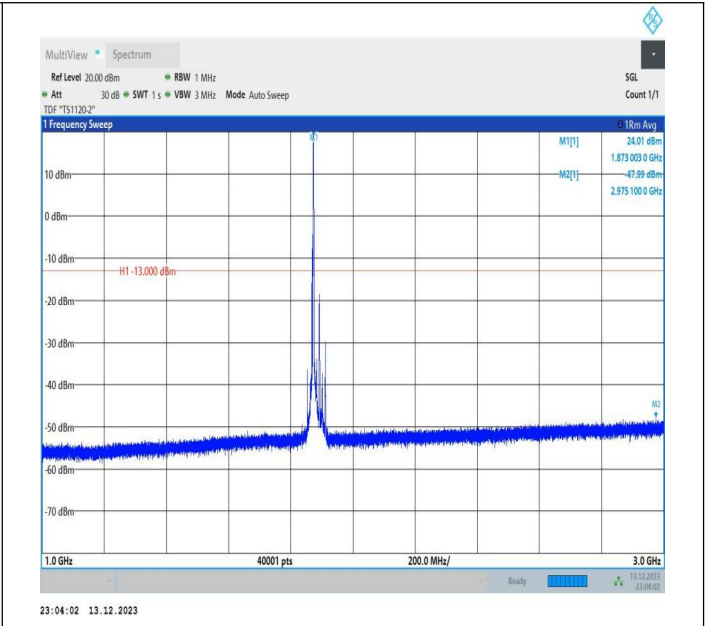
2-2-5MHz-20MHz-QPSK-QPSK-18808-18925-1RB#24-0RB#0 -1000~3000MHz-PASS
