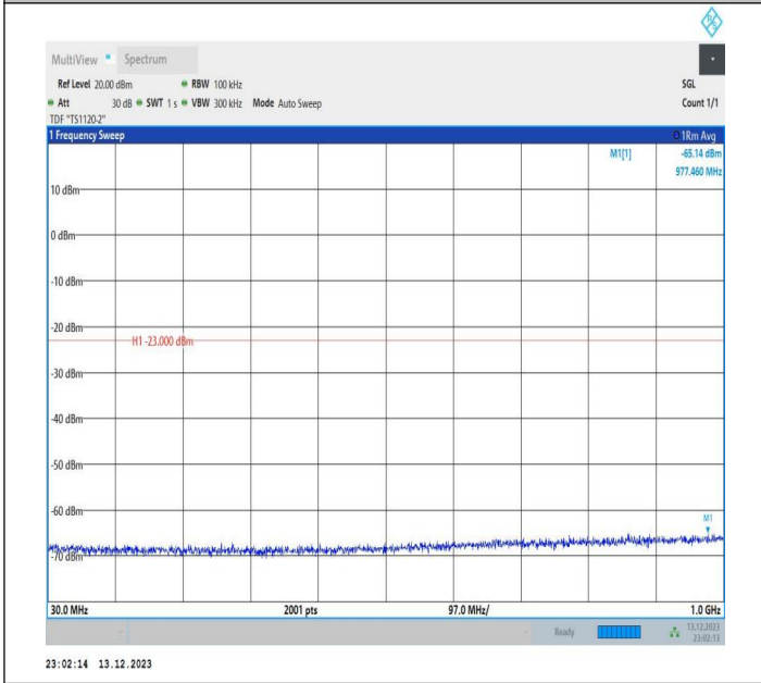
2-2-5MHz-20MHz-QPSK-QPSK-18808-18925-1RB#0-0RB#0-30~1000MHz-PASS
