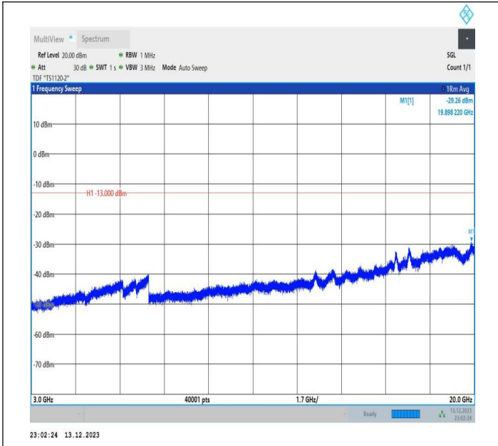
2-2-5MHz-20MHz-QPSK-QPSK-18808-18925-1RB#0-0RB#0-3000~20000MHz-PASS
