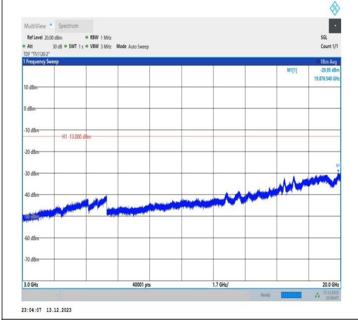
2-2-5MHz-20MHz-QPSK-QPSK-18808-18925-1RB#24-0RB#0 -3000~20000MHz-PASS
