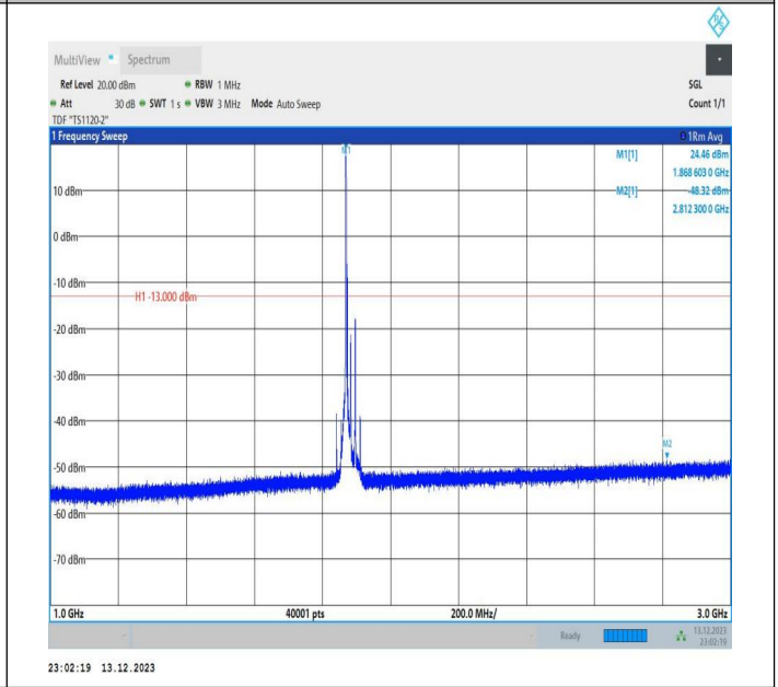
2-2-5MHz-20MHz-QPSK-QPSK-18808-18925-1RB#0-0RB#0-1000~3000MHz-PASS
