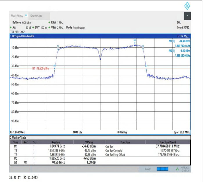
2-2-20MHz-20MHz-16QAM-16QAM-18700-18898-100RB#0-100 RB#0-PASS
