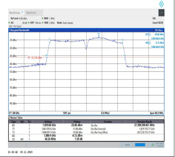
2-2-20MHz-20MHz-16QAM-16QAM-18801-18999-100RB#0-100 RB#0-PASS
