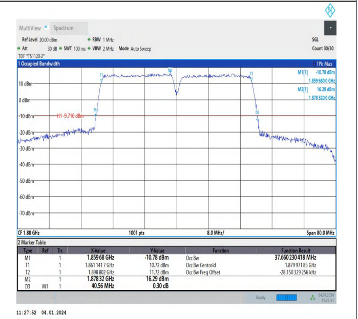
2-2-20MHz-20MHz-64QAM-64QAM-18801-18999-100RB#0-1 00RB#0-PASS
