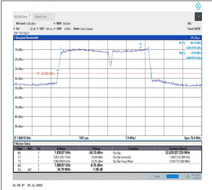
2-2-20MHz-15MHz-QPSK-QPSK-18700-18871-100RB#0-75R B#0-PASS
