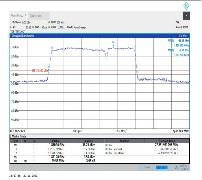
2-2-20MHz-10MHz-16QAM-16QAM-18700-18844-100RB#0-50 ORB#0-PASS
