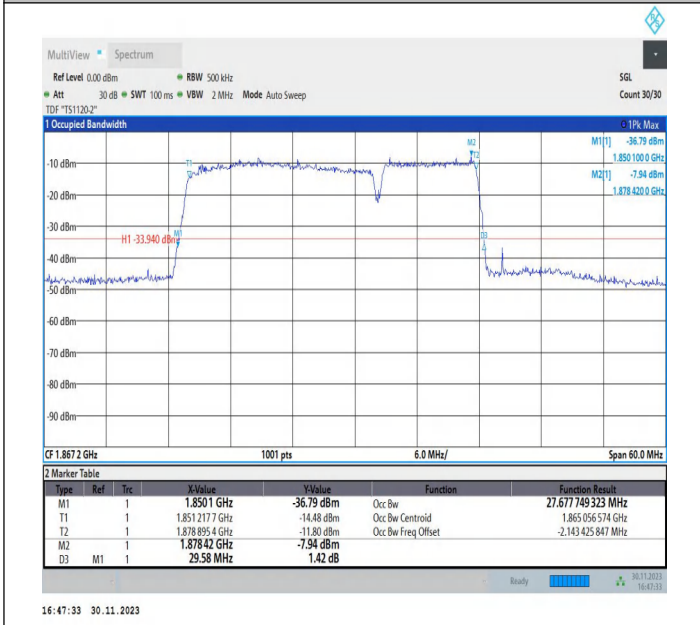
2-2-20MHz-10MHz-QPSK-QPSK-18700-18844-100RB#0-50R B#0-PASS
