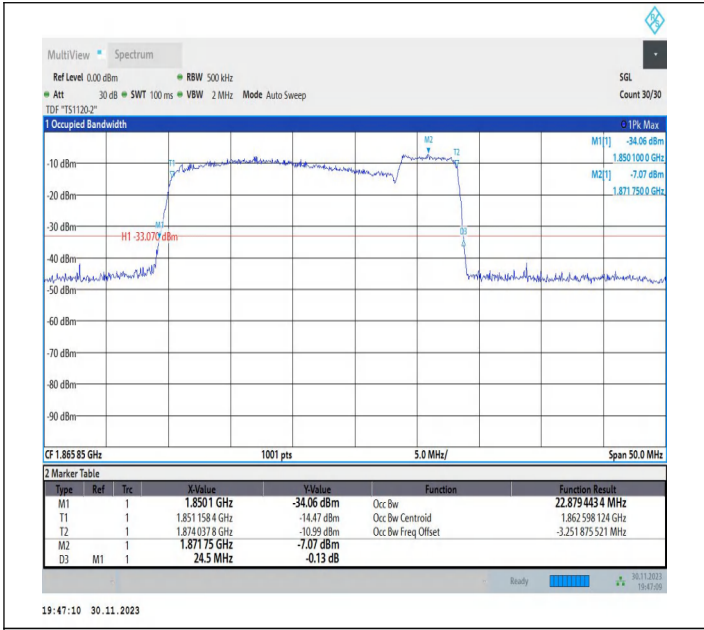
2-2-20MHz-5MHz-QPSK-QPSK-18700-18817-100RB#0-25RB #0-PASS
