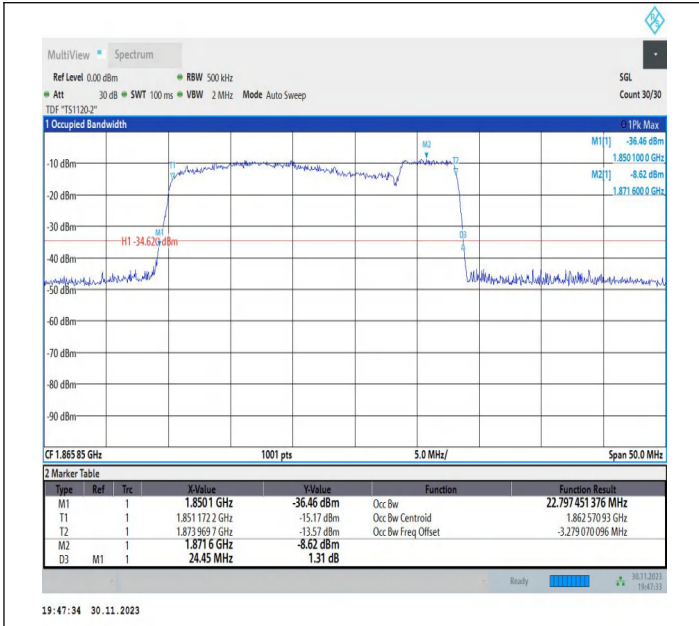
2-2-20MHz-5MHz-16QAM-16QAM-18700-18817-100RB#0-25 RB#0-PASS
