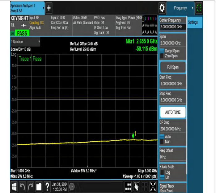
NTNV_N78-3450-3550_PC2_30_100_M_TID2_NS_01_1000_3000_#1
