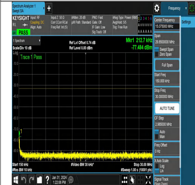
NTNV_N78-3450-3550_PC2_30_100_L_TID6_NS_01_0.15_30_#1
