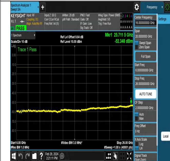
NTNV_N78-3450-3550_PC2_30_100_L_TID2_NS_01_6000_2 6000_#1
