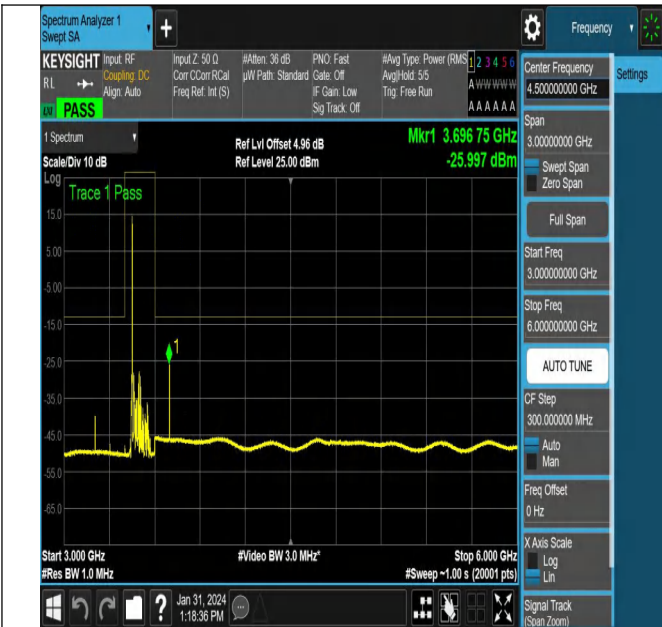
NTNV_N78-3450-3550_PC2_30_100_L_TID2_NS_01_3000_6000_#1
