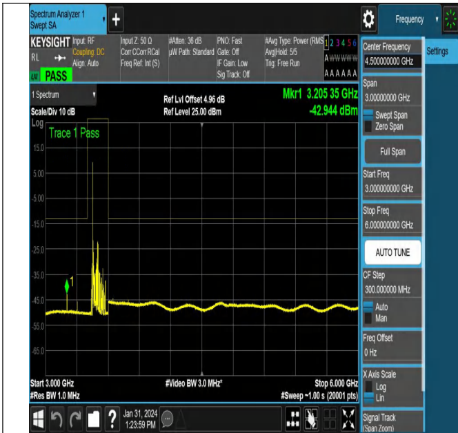
NTNV_N78-3450-3550_PC2_30_100_L_TID17_NS_01_3000_6000_#1
