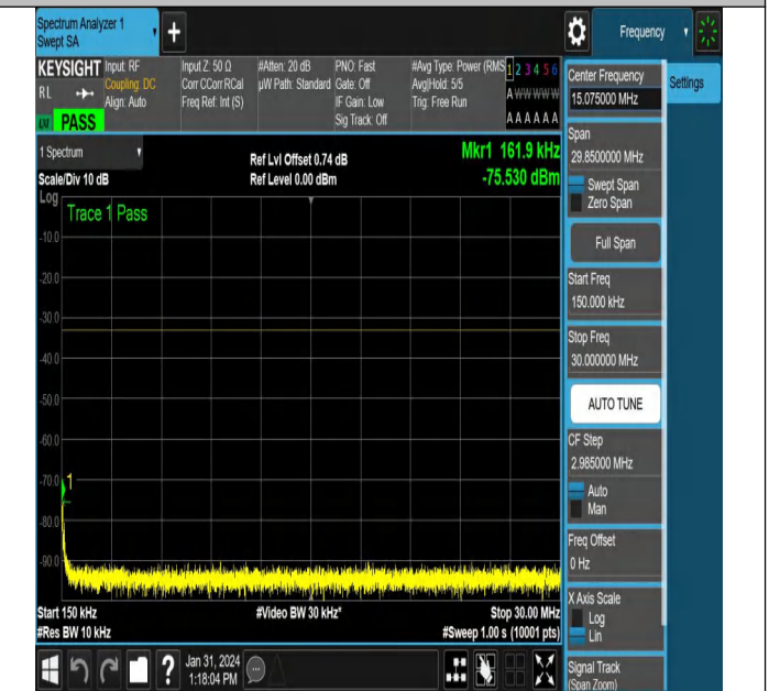
NTNV_N78-3450-3550_PC2_30_100_L_TID2_NS_01_0.15_30_#1
