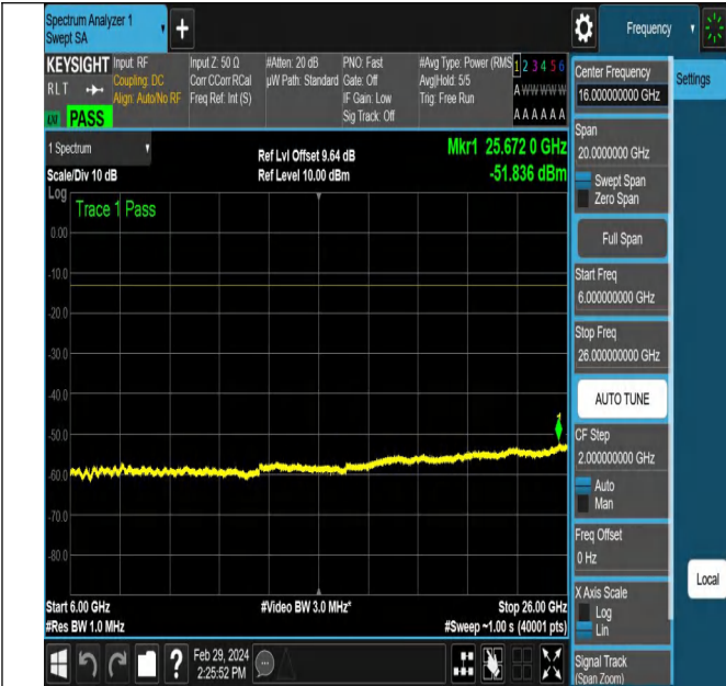
NTNV_N78-3450-3550_PC2_30_100_M_TID6_NS_01_6000_26000_#1
