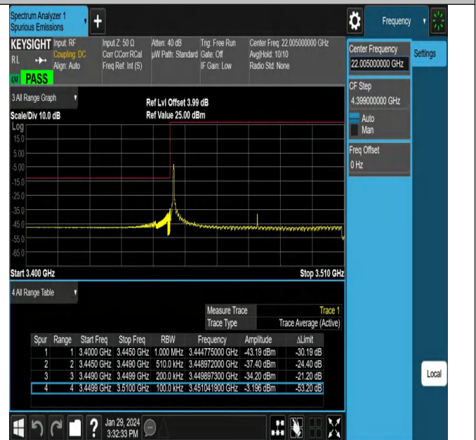
NTNV_N78-3450-3550_PC2_30_60_L_TID23_#1
