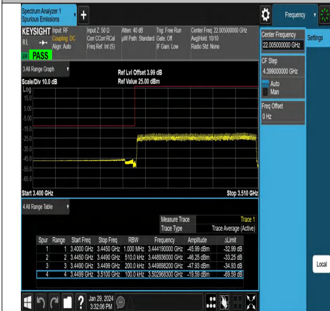
NTNV_N78-3450-3550_PC2_30_60_L_TID22_#1
