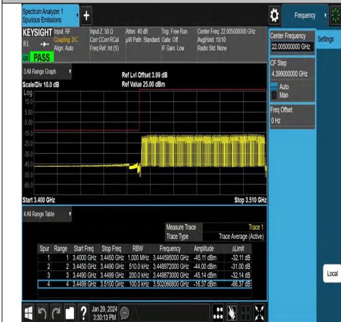
NTNV_N78-3450-3550_PC2_30_60_L_TID16_#1
