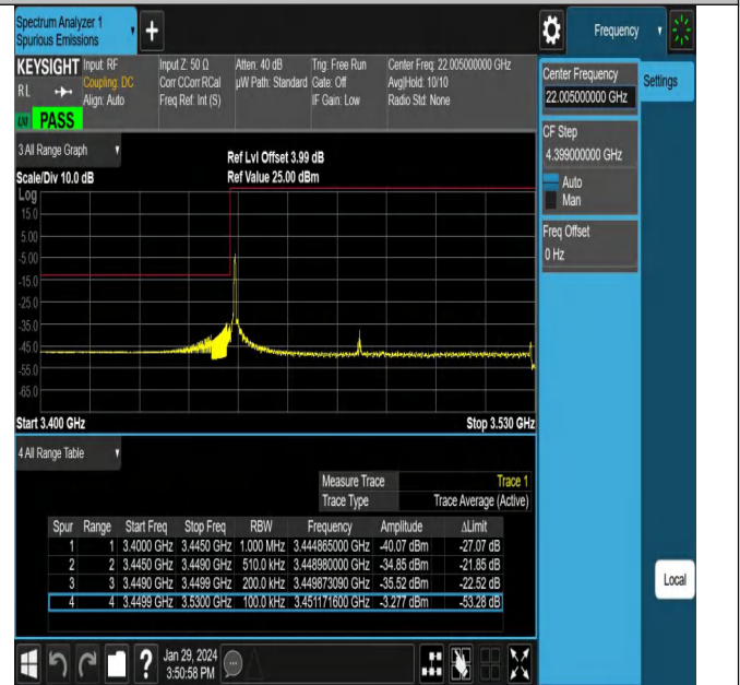
NTNV_N78-3450-3550_PC2_30_80_L_TID23_#1
