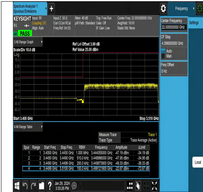
NTNV_N78-3450-3550_PC2_30_60_L_TID25_#1
