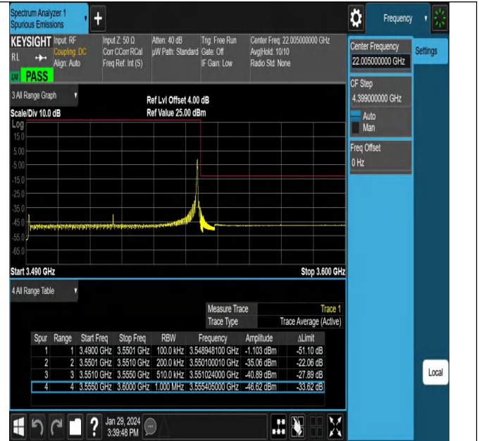
NTNV_N78-3450-3550_PC2_30_60_H_TID18_#1
