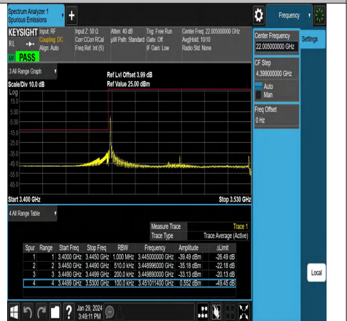
NTNV_N78-3450-3550_PC2_30_80_L_TID17_#1
