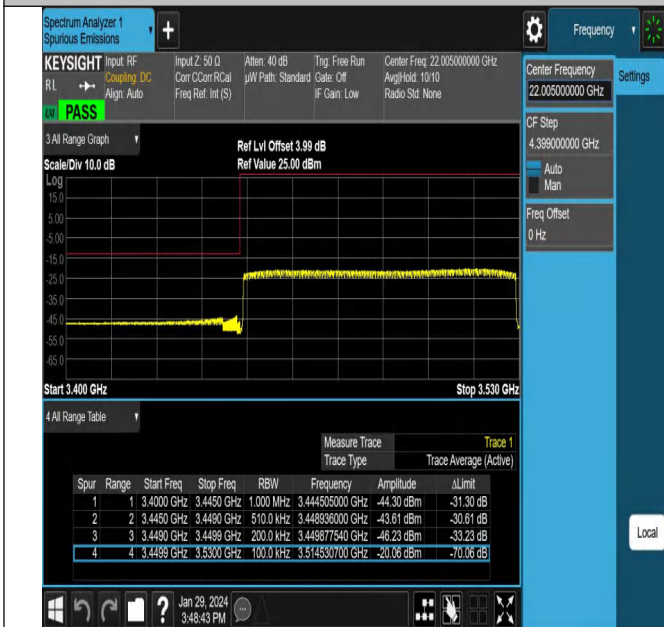
NTNV_N78-3450-3550_PC2_30_80_L_TID16_#1
