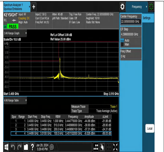
NTNV_N78-3450-3550_PC2_30_60_L_TID14_#1
