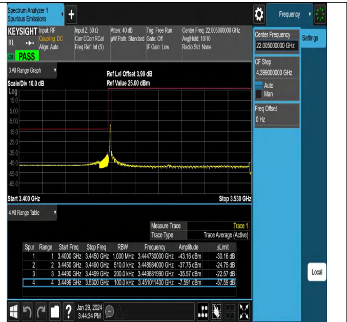
NTNV_N78-3450-3550_PC2_30_80_L_TID2_#1
