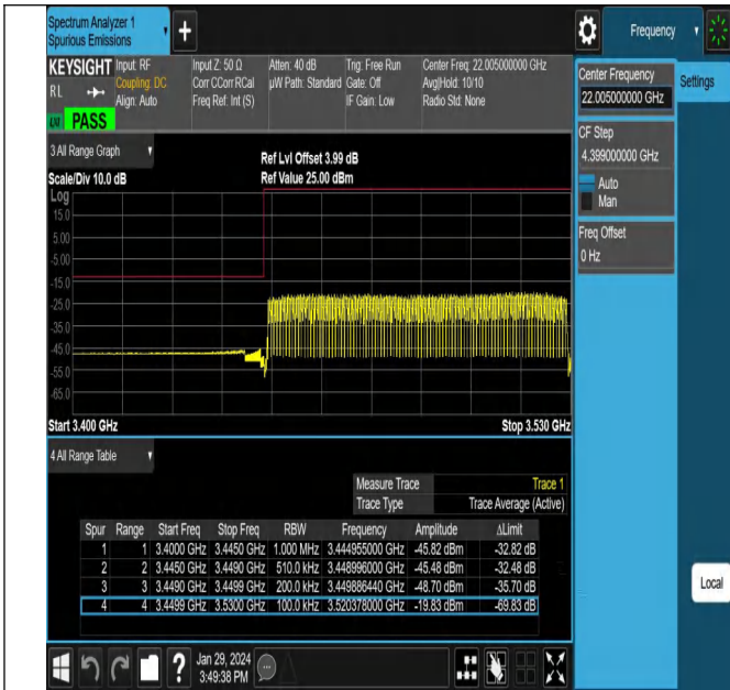
NTNV_N78-3450-3550_PC2_30_80_L_TID19_#1
