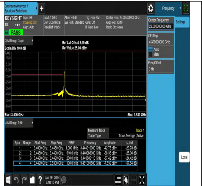
NTNV_N78-3450-3550_PC2_30_80_L_TID14_#1
