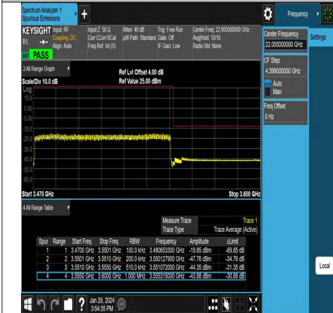
NTNV_N78-3450-3550_PC2_30_80_H_TID7_#1
