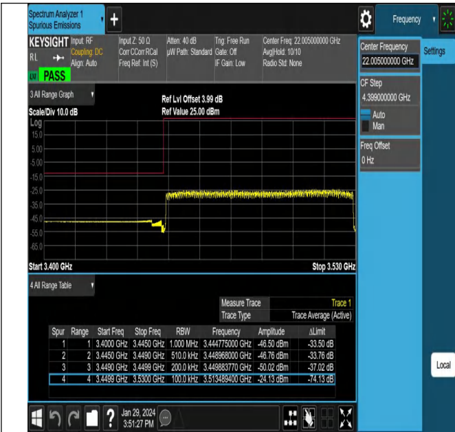
NTNV_N78-3450-3550_PC2_30_80_L_TID25_#1
