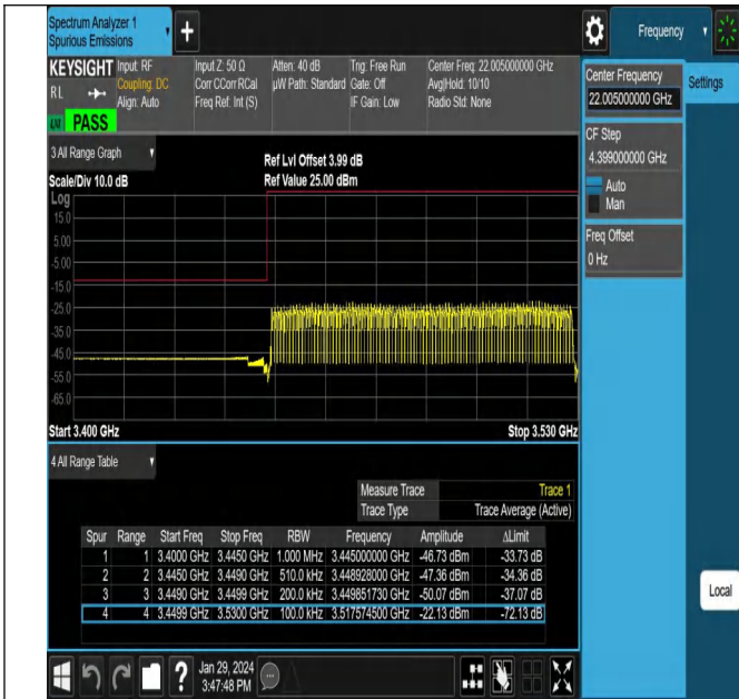
NTNV_N78-3450-3550_PC2_30_80_L_TID13_#1
