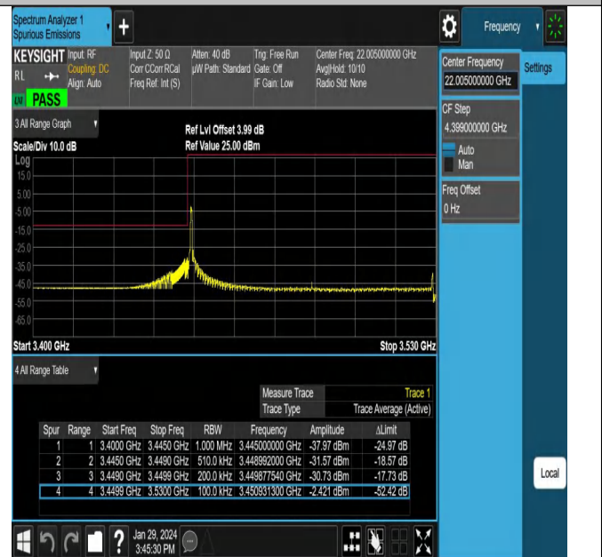
NTNV_N78-3450-3550_PC2_30_80_L_TID5_#1
