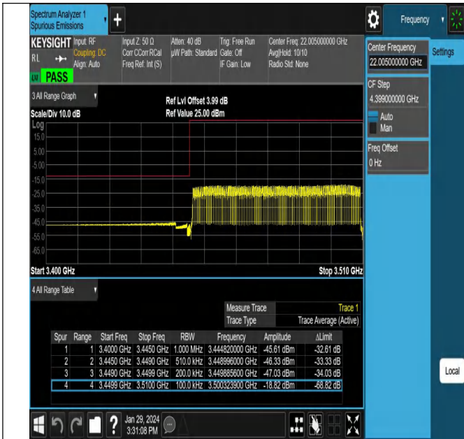
NTNV_N78-3450-3550_PC2_30_60_L_TID19_#1
