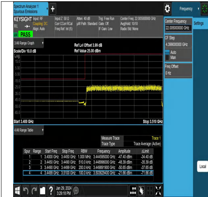
NTNV_N78-3450-3550_PC2_30_60_L_TID13_#1
