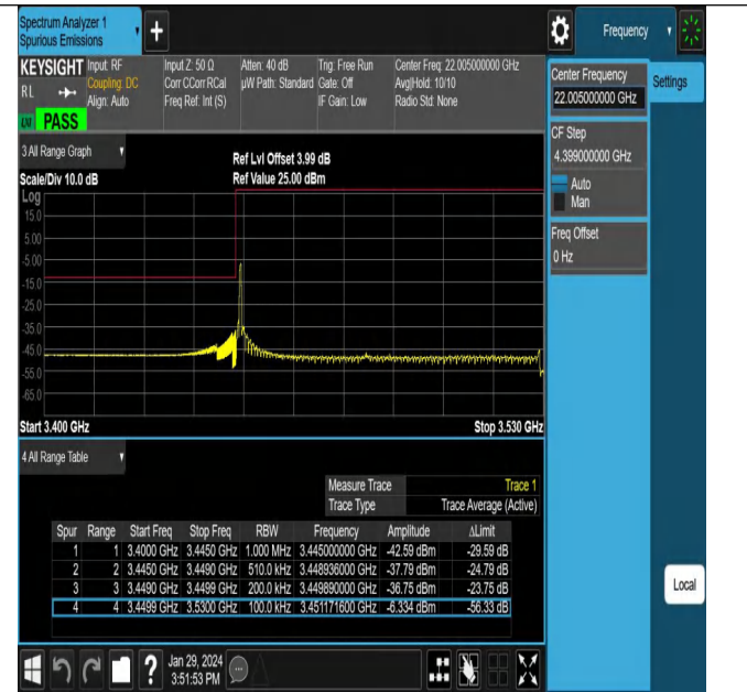
NTNV_N78-3450-3550_PC2_30_80_L_TID26_#1
