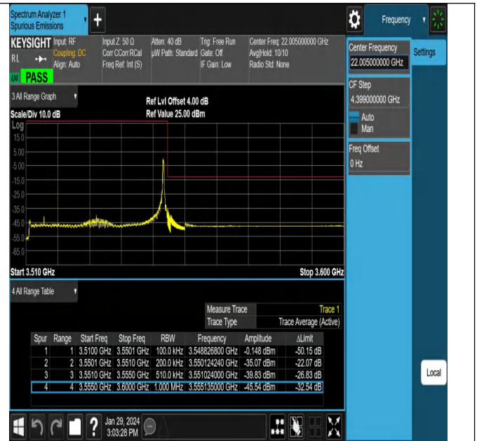
NTNV_N78-3450-3550_PC2_30_40_H_TID18_#1
