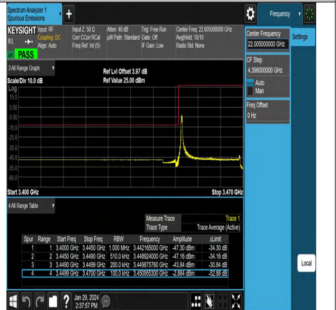
NTNV_N78-3450-3550_PC2_30_20_L_TID23_#1
