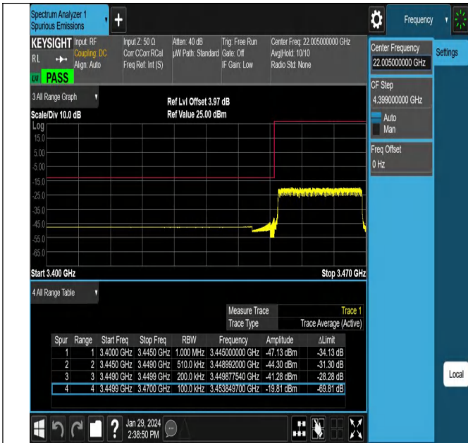
NTNV_N78-3450-3550_PC2_30_20_L_TID25_#1
