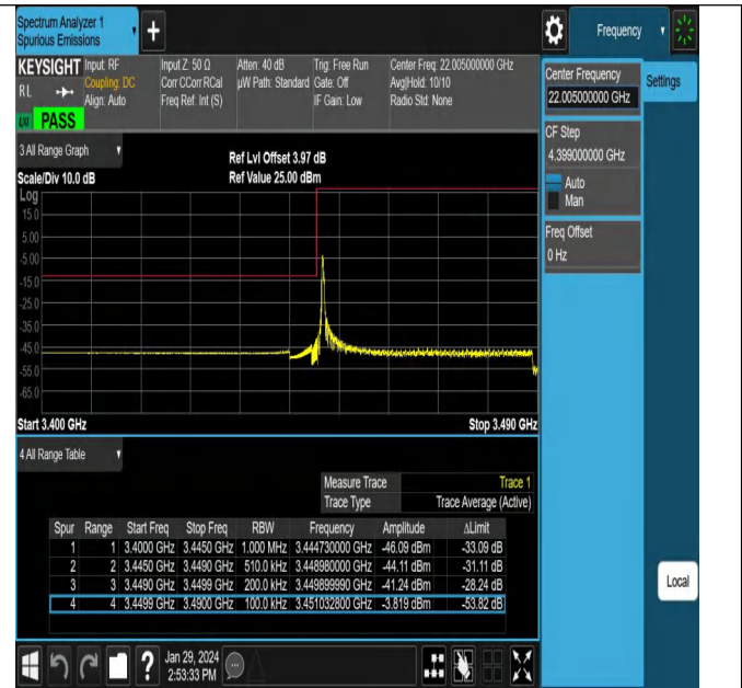
NTNV_N78-3450-3550_PC2_30_40_L_TID14_#1
