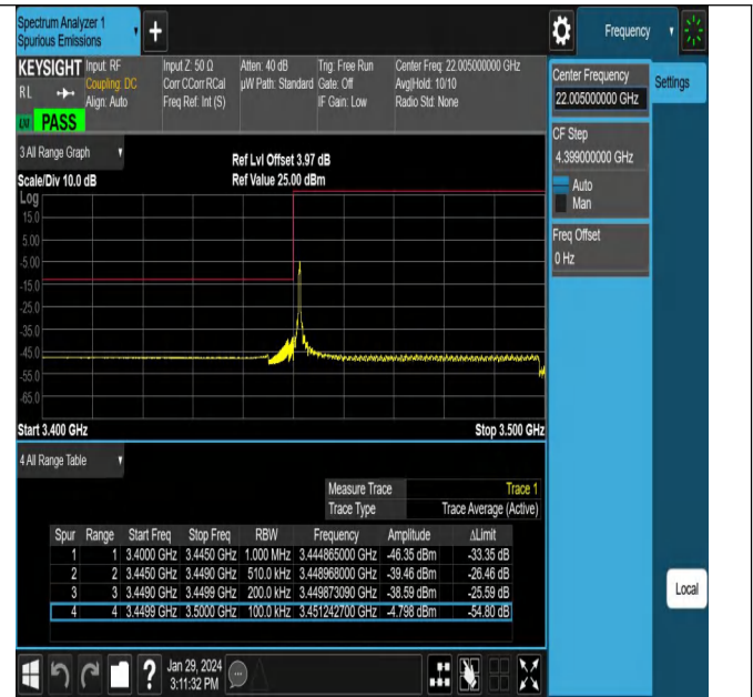
NTNV_N78-3450-3550_PC2_30_50_L_TID14_#1
