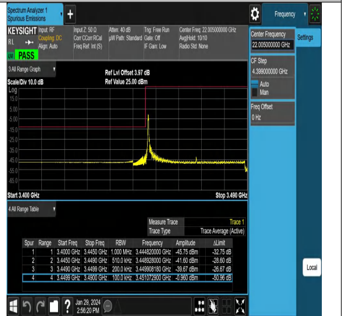
NTNV_N78-3450-3550_PC2_30_40_L_TID23_#1
