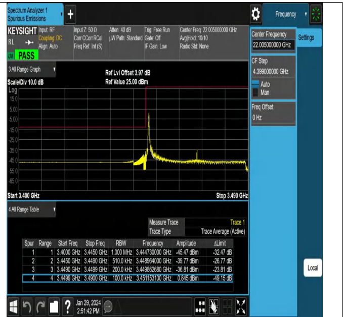
NTNV_N78-3450-3550_PC2_30_40_L_TID8_#1
