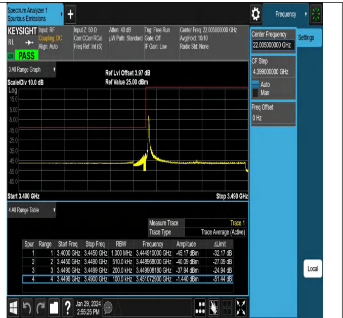
NTNV_N78-3450-3550_PC2_30_40_L_TID20_#1
