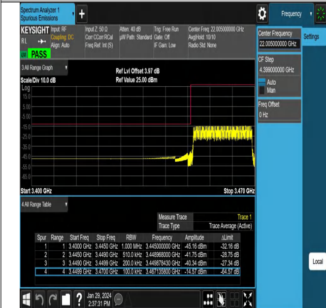
NTNV_N78-3450-3550_PC2_30_20_L_TID22_#1
