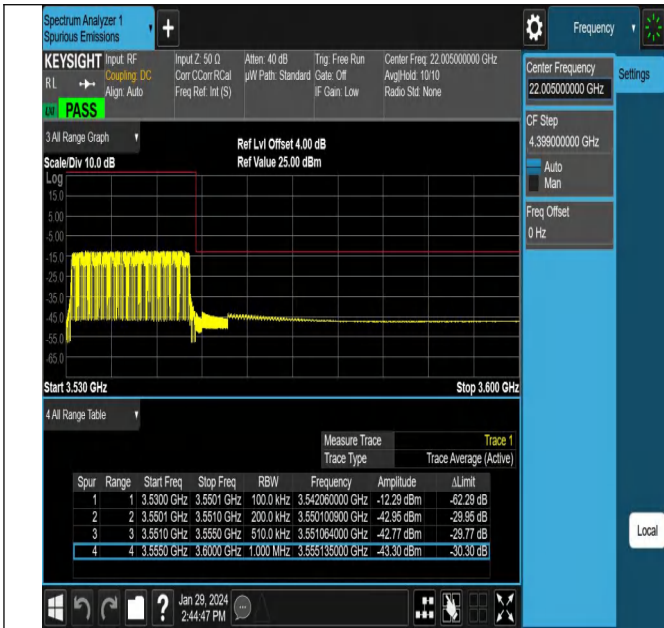
NTNV_N78-3450-3550_PC2_30_20_H_TID16_#1
