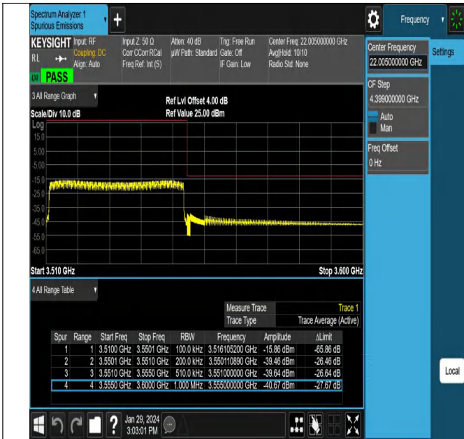
NTNV_N78-3450-3550_PC2_30_40_H_TID16_#1
