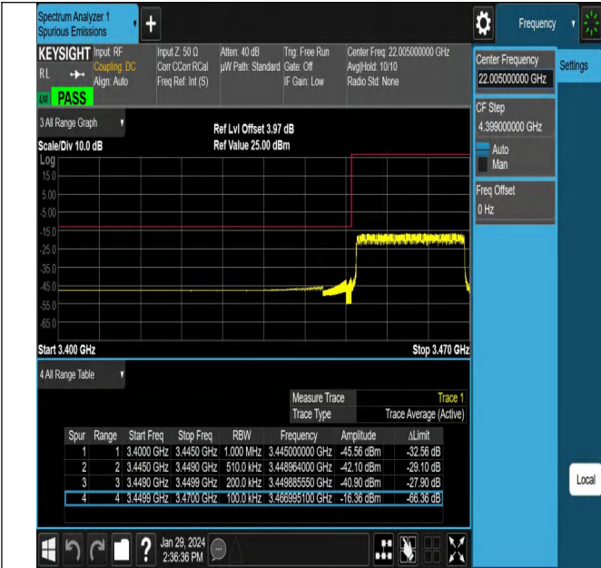
NTNV_N78-3450-3550_PC2_30_20_L_TID19_#1
