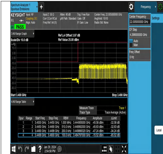
NTNV_N78-3450-3550_PC2_30_40_L_TID19_#1
