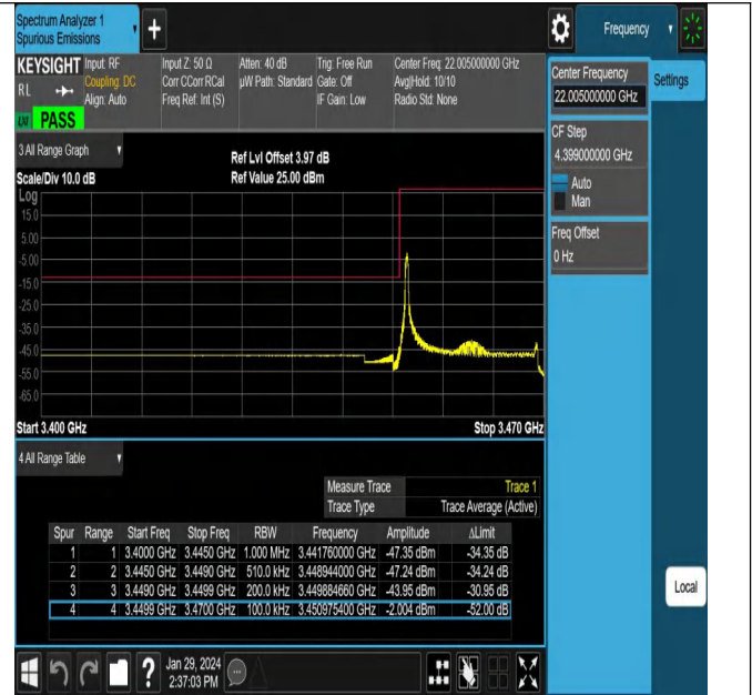
NTNV_N78-3450-3550_PC2_30_20_L_TID20_#1
