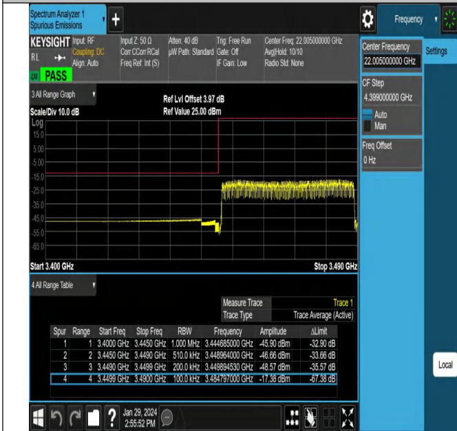
NTNV_N78-3450-3550_PC2_30_40_L_TID22_#1
