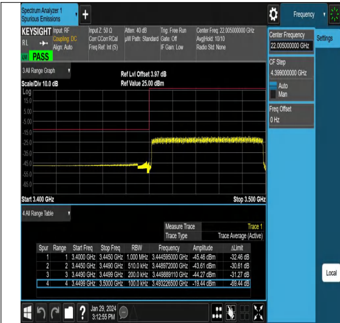
NTNV_N78-3450-3550_PC2_30_50_L_TID19_#1
