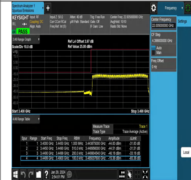
NTNV_N78-3450-3550_PC2_30_40_L_TID16_#1
