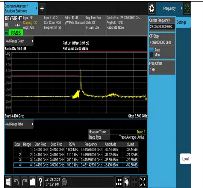
NTNV_N78-3450-3550_PC2_30_50_L_TID20_#1
