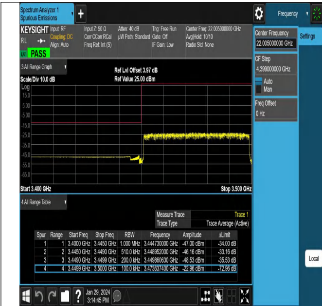
NTNV_N78-3450-3550_PC2_30_50_L_TID25_#1
