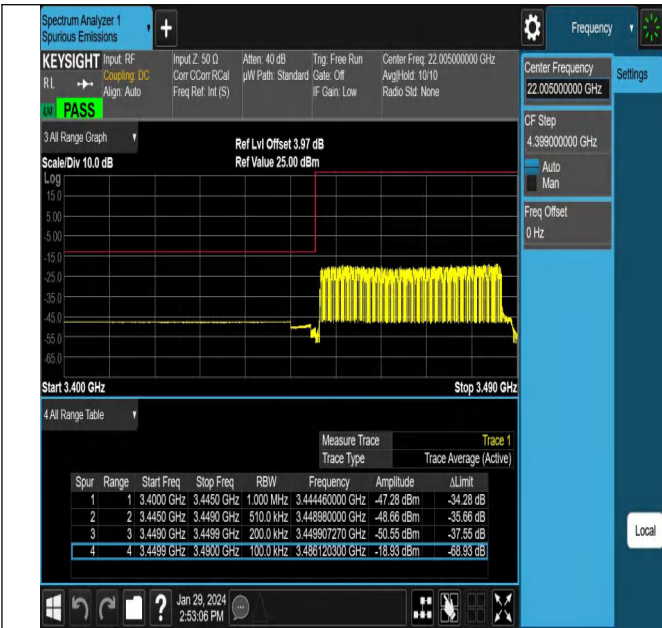
NTNV_N78-3450-3550_PC2_30_40_L_TID13_#1
