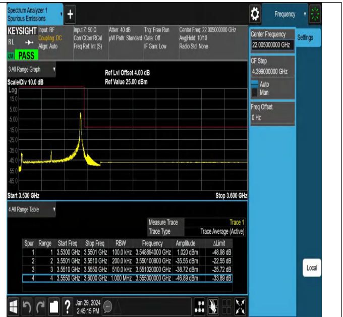
NTNV_N78-3450-3550_PC2_30_20_H_TID18_#1
