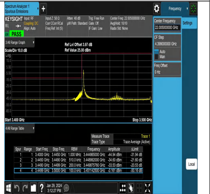
NTNV_N78-3450-3550_PC2_30_50_L_TID17_#1
