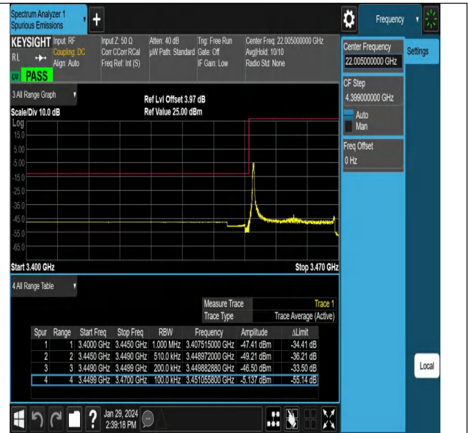
NTNV_N78-3450-3550_PC2_30_20_L_TID26_#1
