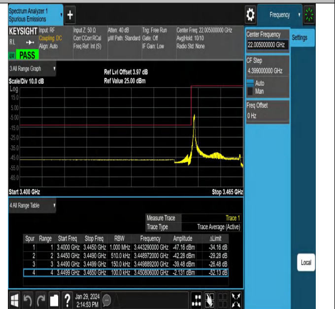
NTNV_N78-3450-3550_PC2_30_15_L_TID11_#1
