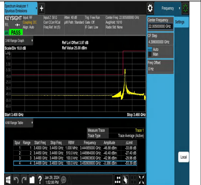
NTNV_N78-3450-3550_PC2_30_10_L_TID23_#1
