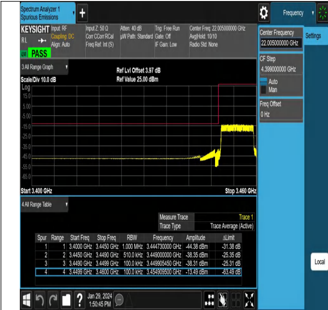
NTNV_N78-3450-3550_PC2_30_10_L_TID19_#1
