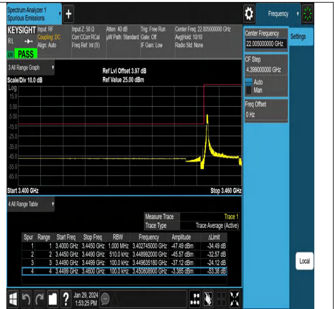
NTNV_N78-3450-3550_PC2_30_10_L_TID26_#1
