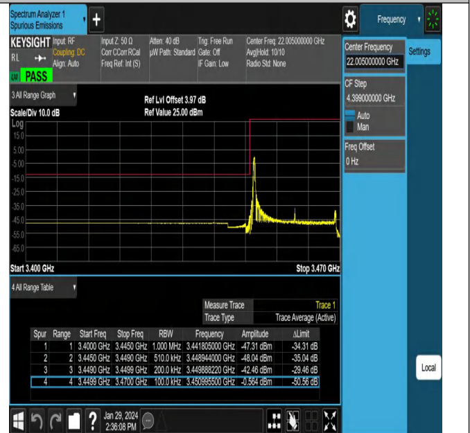
NTNV_N78-3450-3550_PC2_30_20_L_TID17_#1
