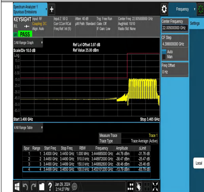
NTNV_N78-3450-3550_PC2_30_15_L_TID10_#1
