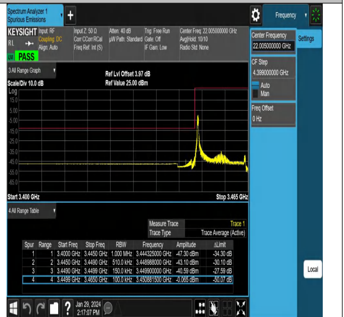
NTNV_N78-3450-3550_PC2_30_15_L_TID17_#1
