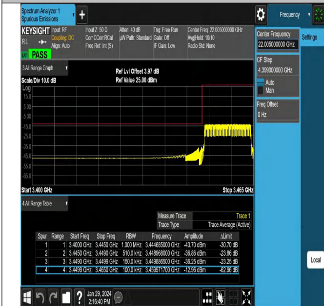
NTNV_N78-3450-3550_PC2_30_15_L_TID16_#1
