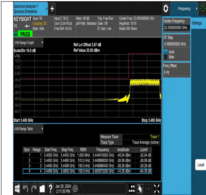
NTNV_N78-3450-3550_PC2_30_15_L_TID19_#1
