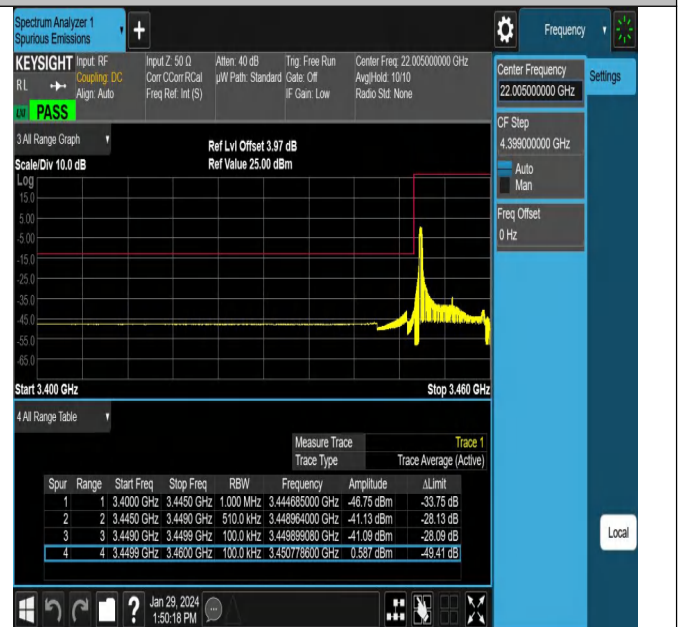
NTNV_N78-3450-3550_PC2_30_10_L_TID17_#1
