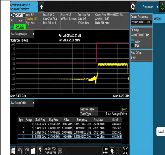
NTNV_N78-3450-3550_PC2_30_20_L_TID16_#1
