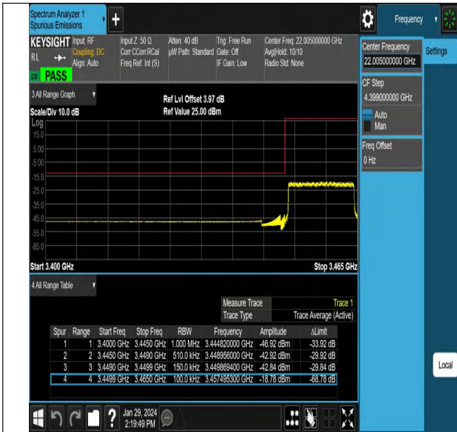
NTNV_N78-3450-3550_PC2_30_15_L_TID25_#1
