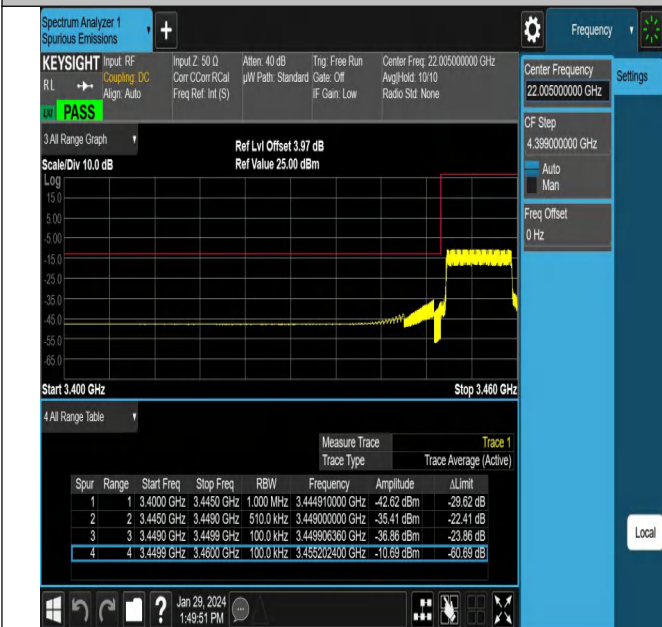
NTNV_N78-3450-3550_PC2_30_10_L_TID16_#1
