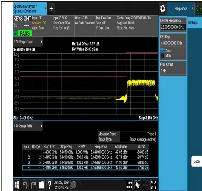
NTNV_N78-3450-3550_PC2_30_15_L_TID13_#1
