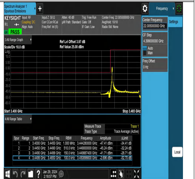
NTNV_N78-3450-3550_PC2_30_15_L_TID23_#1
