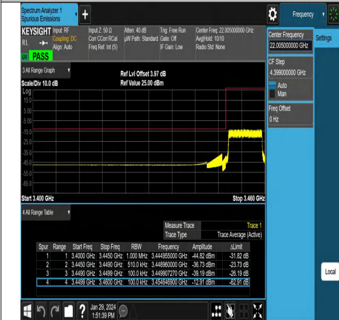
NTNV_N78-3450-3550_PC2_30_10_L_TID22_#1
