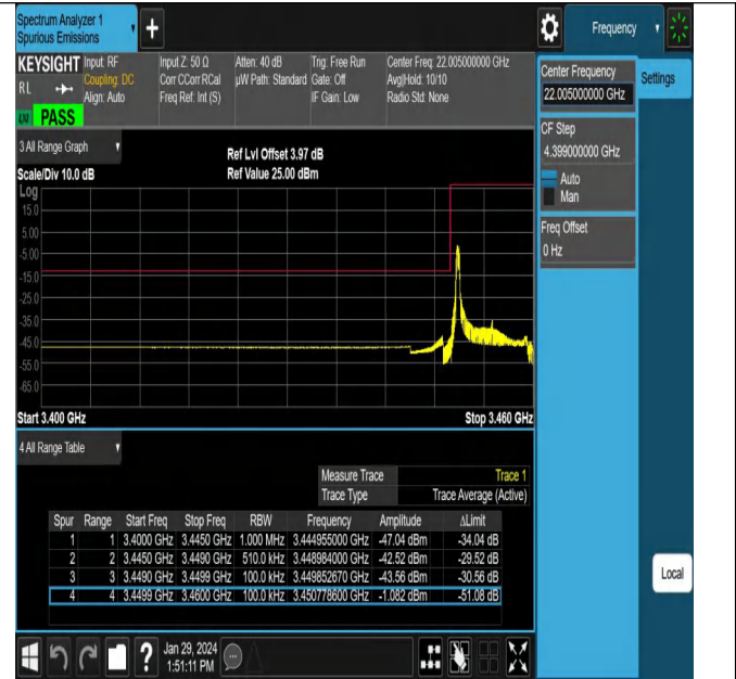
NTNV_N78-3450-3550_PC2_30_10_L_TID20_#1
