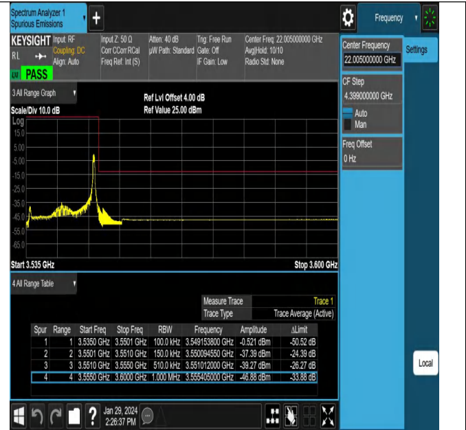
NTNV_N78-3450-3550_PC2_30_15_H_TID18_#1
