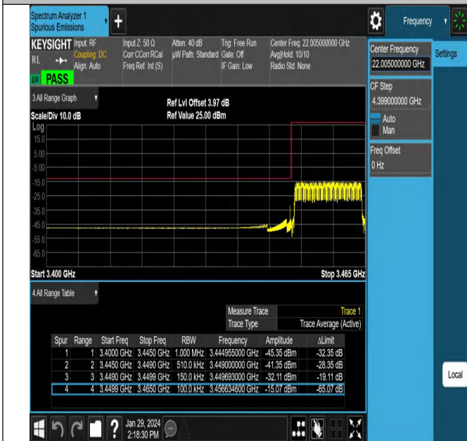
NTNV_N78-3450-3550_PC2_30_15_L_TID22_#1
