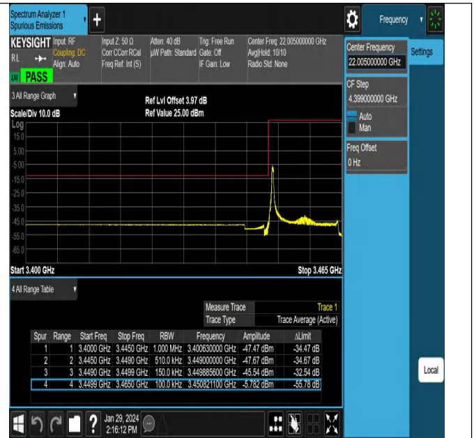
NTNV_N78-3450-3550_PC2_30_15_L_TID14_#1
