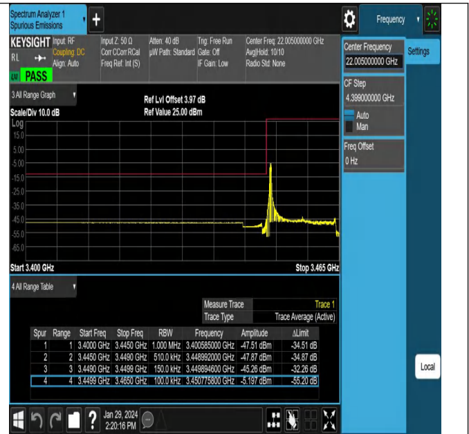
NTNV_N78-3450-3550_PC2_30_15_L_TID26_#1
