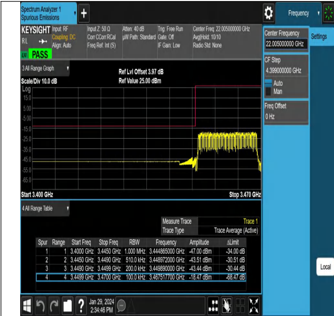
NTNV_N78-3450-3550_PC2_30_20_L_TID13_#1
