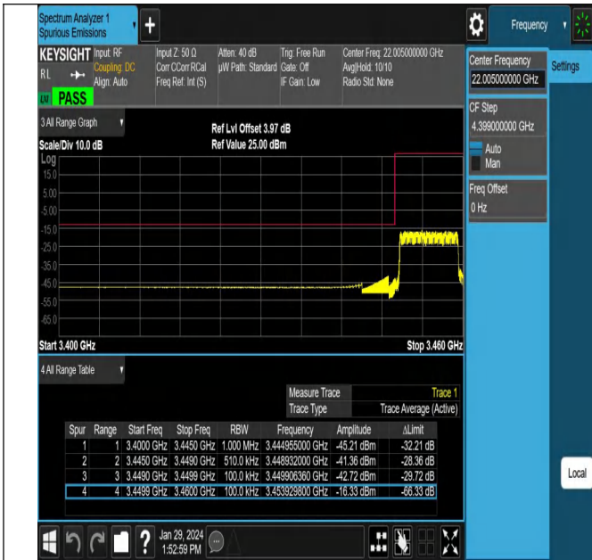
NTNV_N78-3450-3550_PC2_30_10_L_TID25_#1
