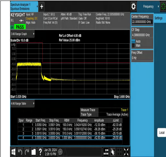
NTNV_N78-3450-3550_PC2_30_15_H_TID16_#1
