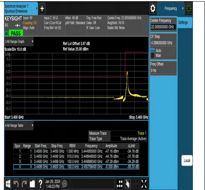
NTNV_N78-3450-3550_PC2_30_10_L_TID14_#1
