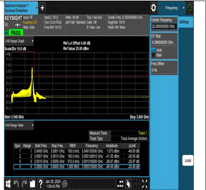
NTNV_N78-3450-3550_PC2_30_10_H_TID18_#1
