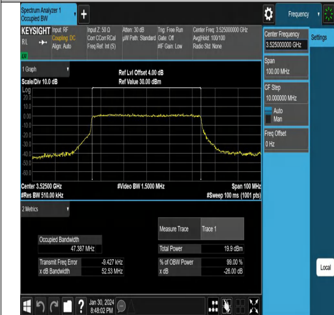
NTV_N78-3450-3550_PC2_30_50_H_TID7_Ant1#1
