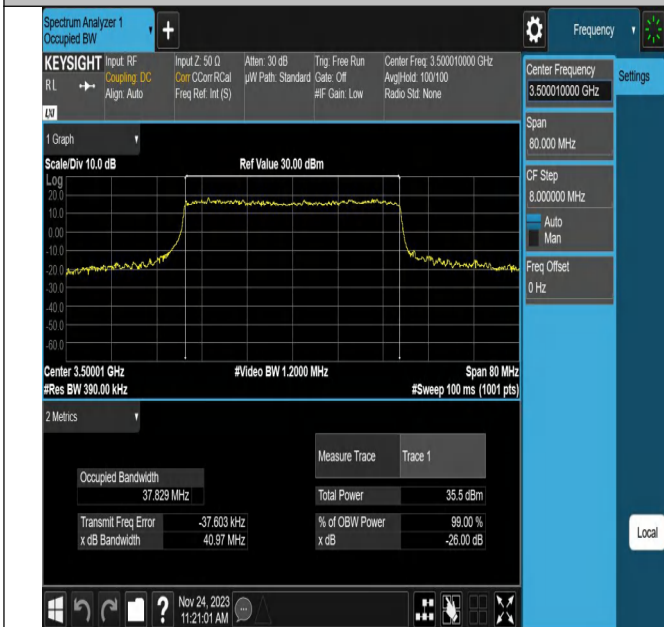
NTV_N78-3450-3550_PC2_30_40_M_TID7_Ant1#1
