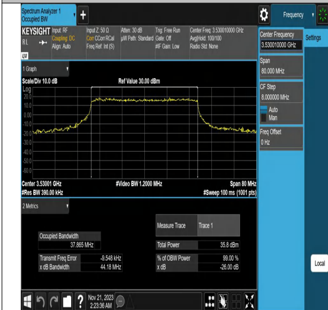
NTV_N78-3450-3550_PC_30_40_H_TID6_Ant1#1
