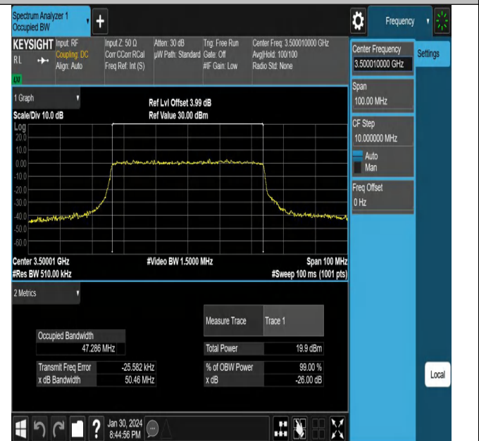
NTV_N78-3450-3550_PC2_30_50_M_TID7_Ant1#1
