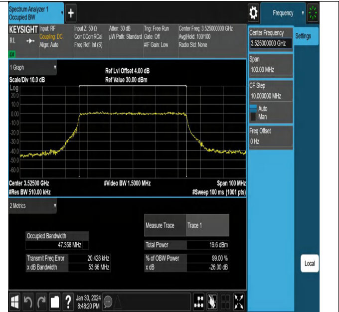
NTV_N78-3450-3550_PC2_30_50_H_TID8_Ant1#1
