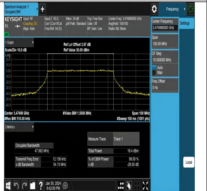
NTV_N78-3450-3550_PC2_30_50_L_TID8_Ant1#1
