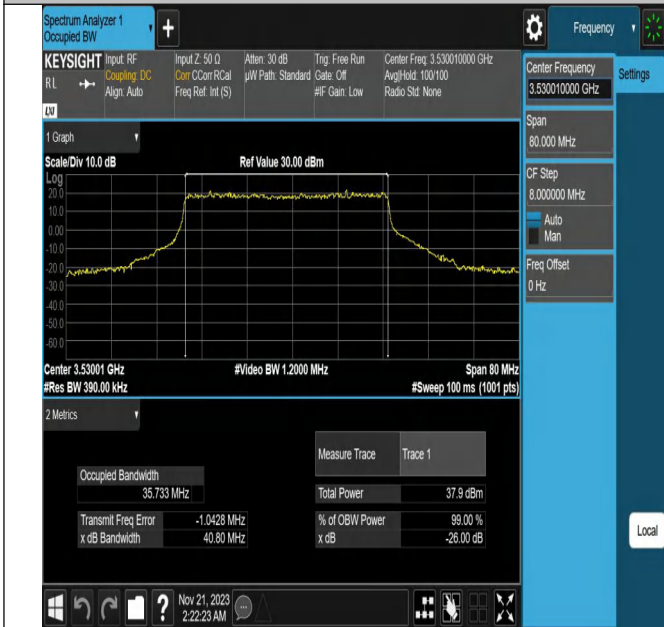
NTV_N78-3450-3550_PC2_30_40_H_TID2_Ant1#1
