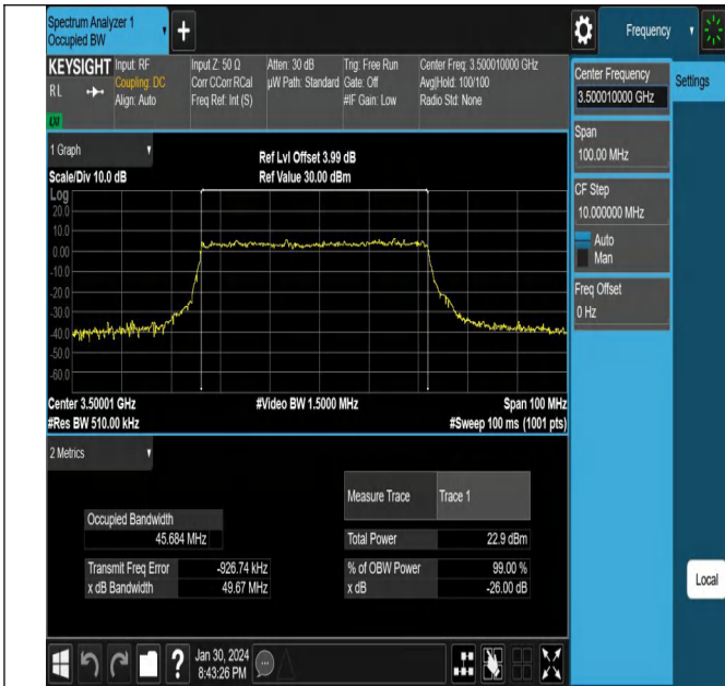
NTV_N78-3450-3550_PC2_30_50_M_TID2_Ant1#1
