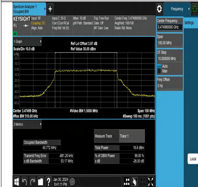
NTV_N78-3450-3550_PC2_30_50_L_TID5_Ant1#1
