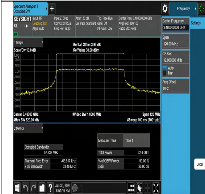
NTV_N78-3450-3550_PC2_30_60_L_TID6_Ant1#1
