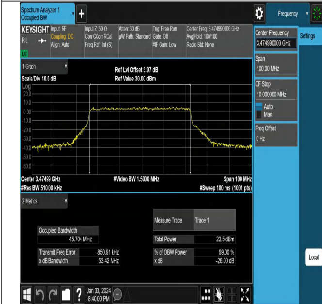
NTV_N78-3450-3550_PC2_30_50_L_TID1_Ant1#1
