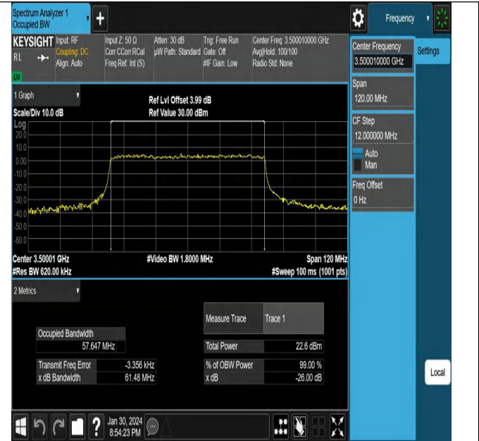
NTV_N78-3450-3550_PC2_30_60_M_TID6_Ant1#1
