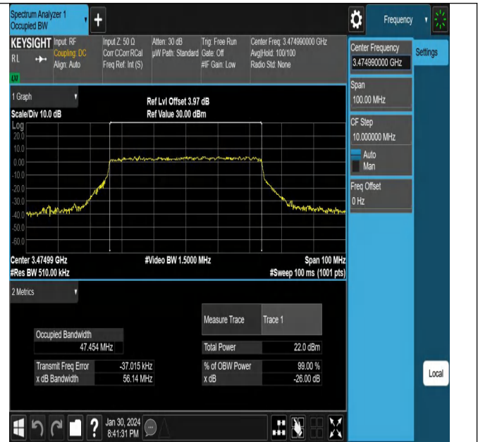
NTV_N78-3450-3550_PC2_30_50_L_TID6_Ant1#1
