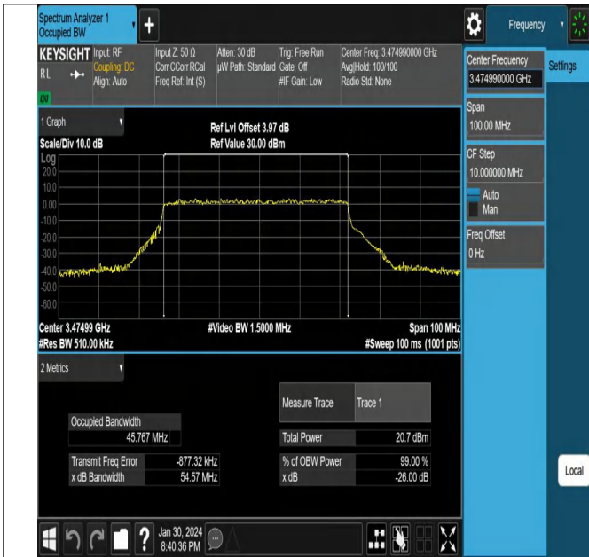
NTV_N78-3450-3550_PC2_30_50_L_TID3_Ant1#1
