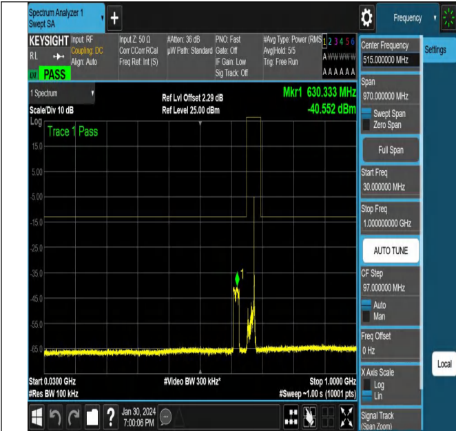
NTNV_N71_PC3_15_20_L_TID18_NS_01_30_1000_#1
