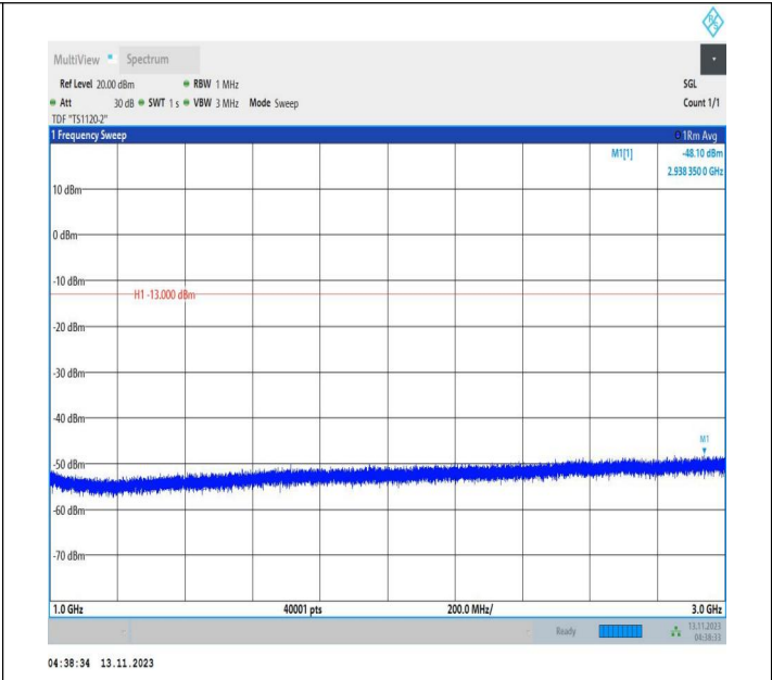
Band71_10MHz_QPSK_133172_1RB#0_1000~3000_1000~3000
