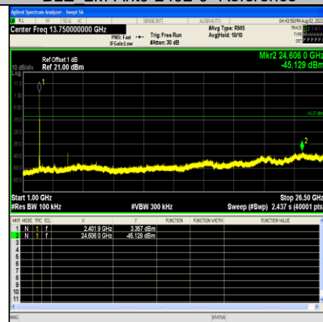
BLE 2M-Ant0-2402-1000~26500
