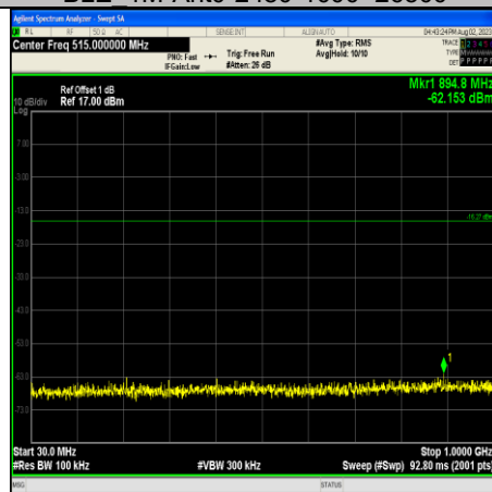
BLE 2M-Ant0-2402-30~1000
