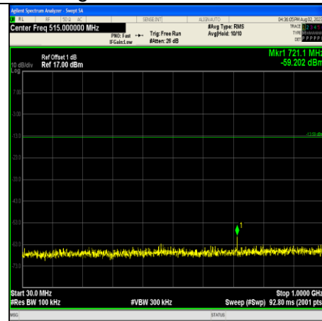
BLE 1M-Ant0-2480-30~1000
