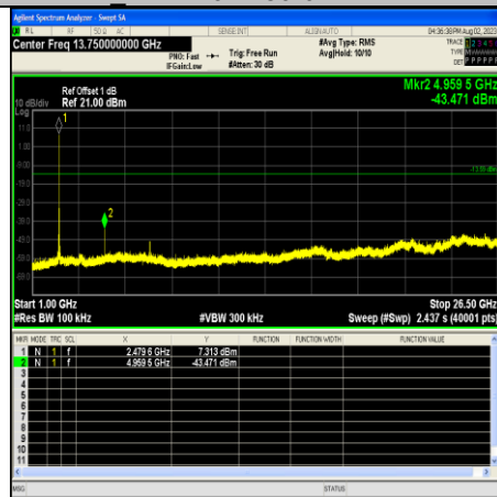
BLE 1M-Ant0-2480-1000~26500
