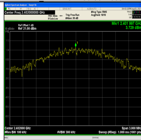
BLE 2M-Ant0-2402-0~Reference
