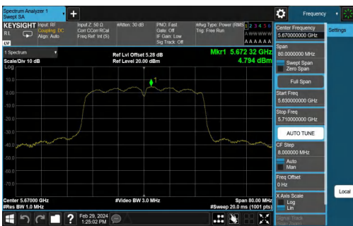
11N40SISO-Ant1-5710_UNII-2C-PASS
