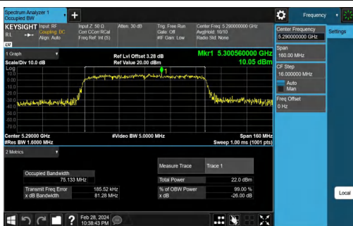
11AC80MIMO-Ant1-5290
