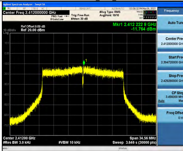
11ax20MIMO Ant0 2412
