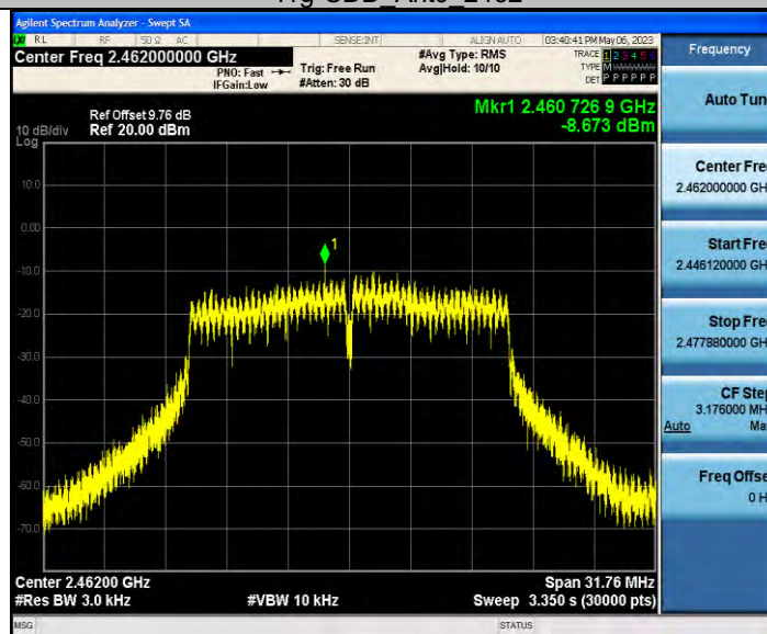
11g-CDD Ant0 2462
