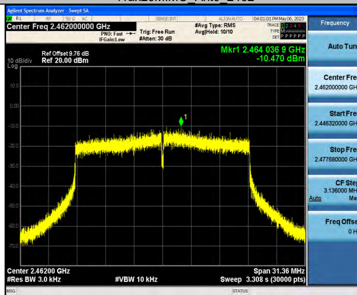
11ax20MIMO Ant0 2462
