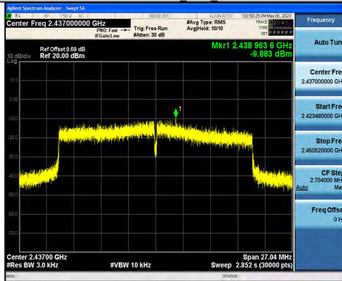
11ax20MIMO Ant0 2437
