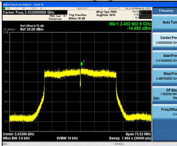
11ax40MIMO Ant0 2452
