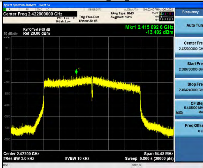
11ax40MIMO Ant0 2422
