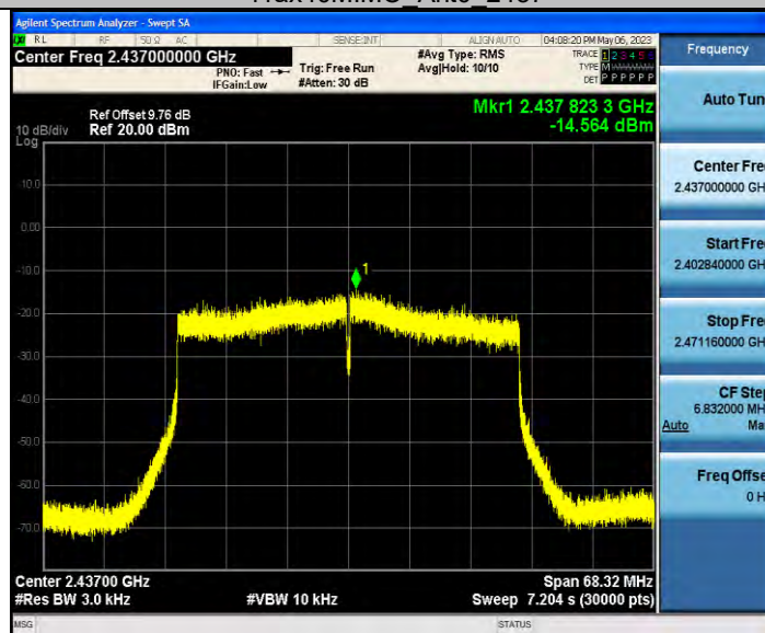
11ax40MIMO Ant0 2437
