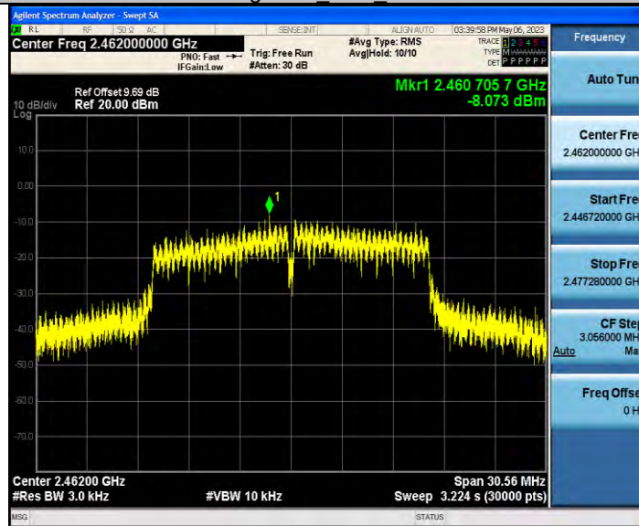
11g-CDD Ant0 2462
