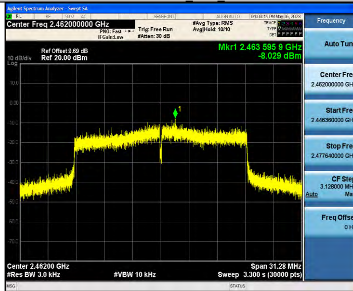
11ax20MIMO Ant0 2462
