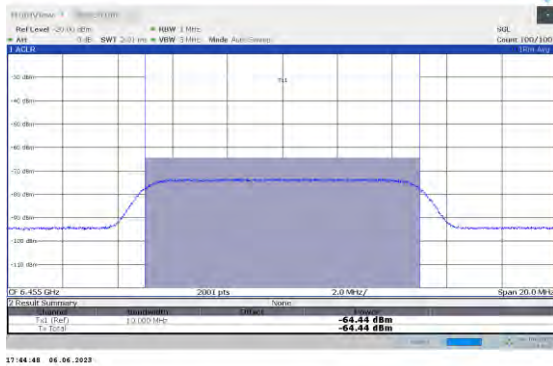
802.11 ax (HE20) /6455MHz Threshold Level (TL)
