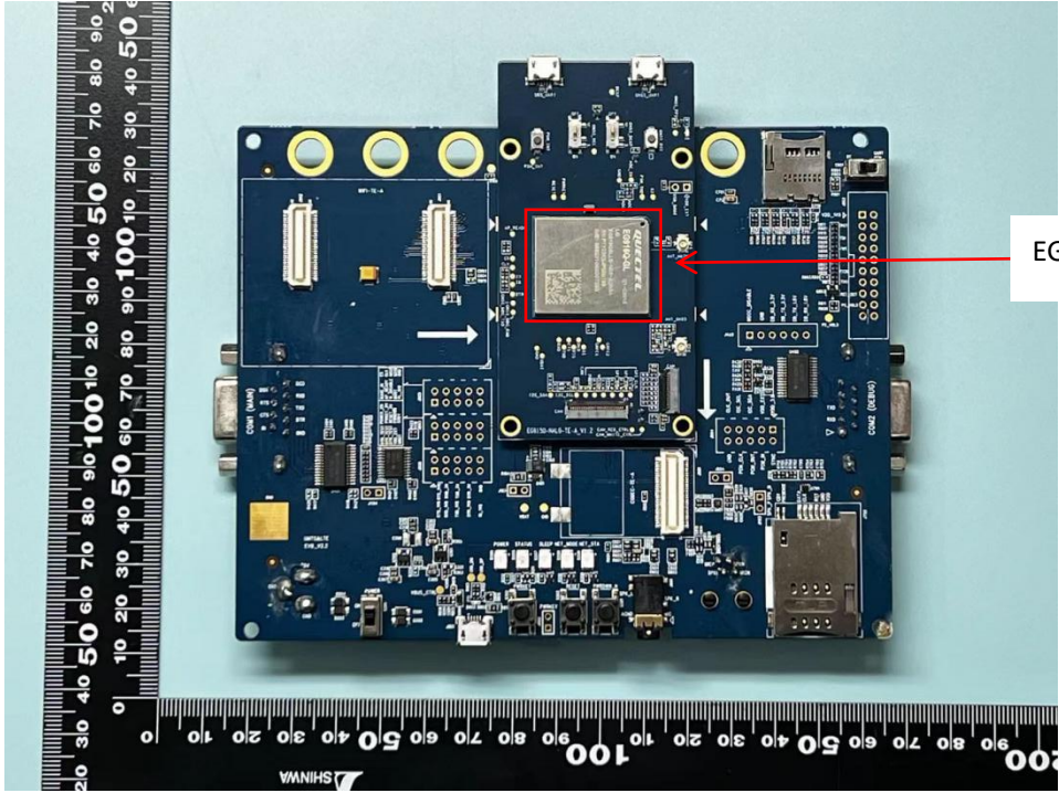
EG916Q-GL + EVB_Top
