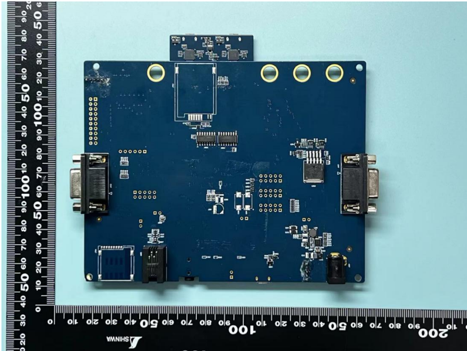
EG916Q-GL + EVB_Bottom
