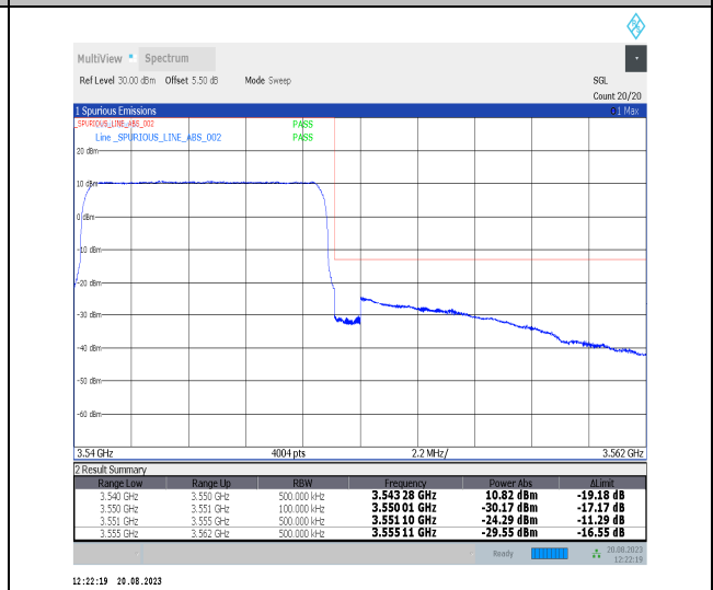
Band42_10MHz_QPSK_43040_50RB#0
