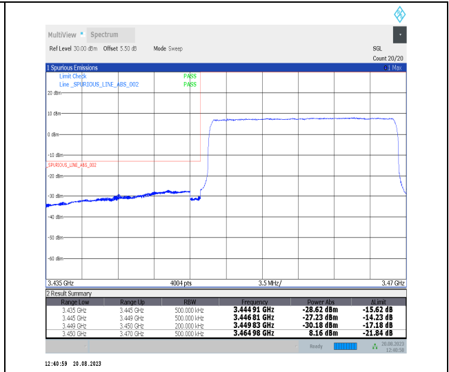
Band42_20MHz_QPSK_42190_100RB#0
