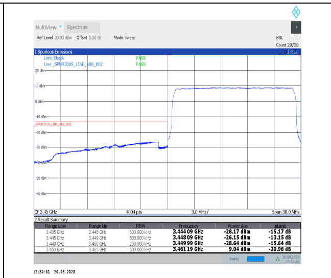
Band42_15MHz_QPSK_42165_75RB#0
