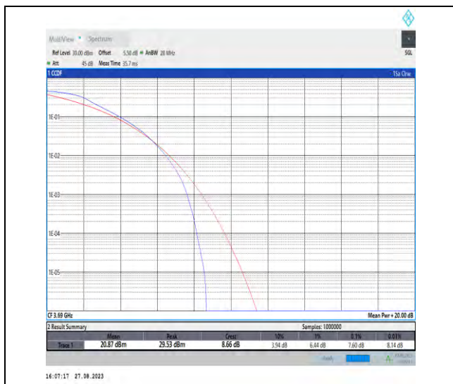
Band43-20MHz-QPSK-44490-100RB#0-PASS
