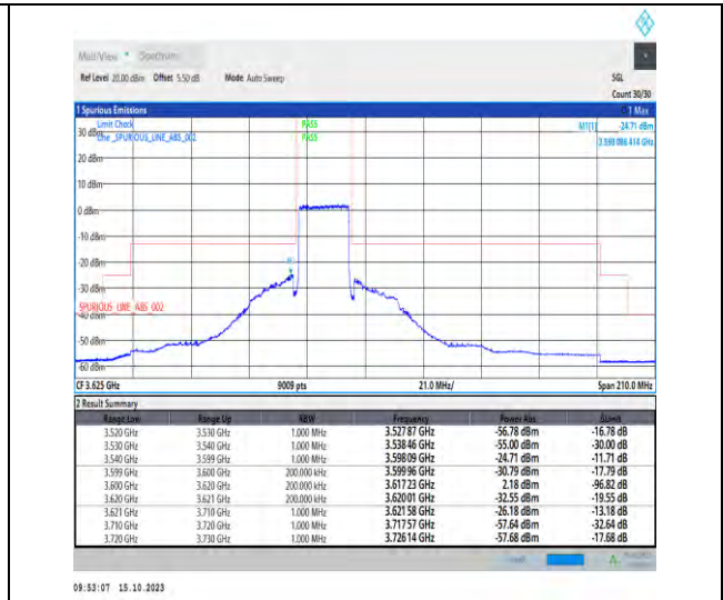
Band43_20MHz_QPSK_43690_100RB#0
