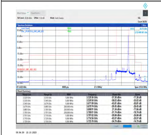
Band43_20MHz_QPSK_44490_1RB#99
