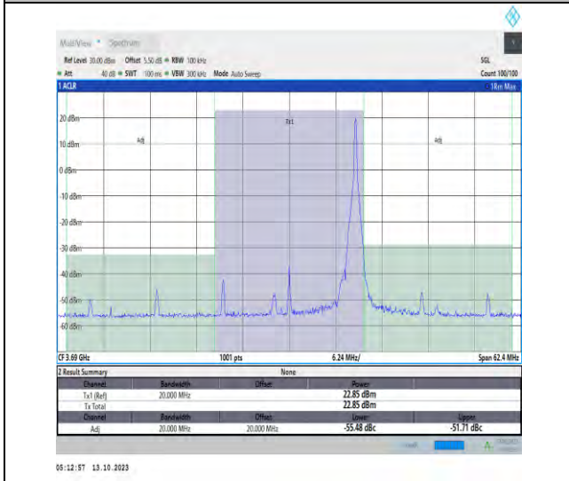
43(3600-3700)-20MHz-QPSK-44490-1RB#99-PASS
