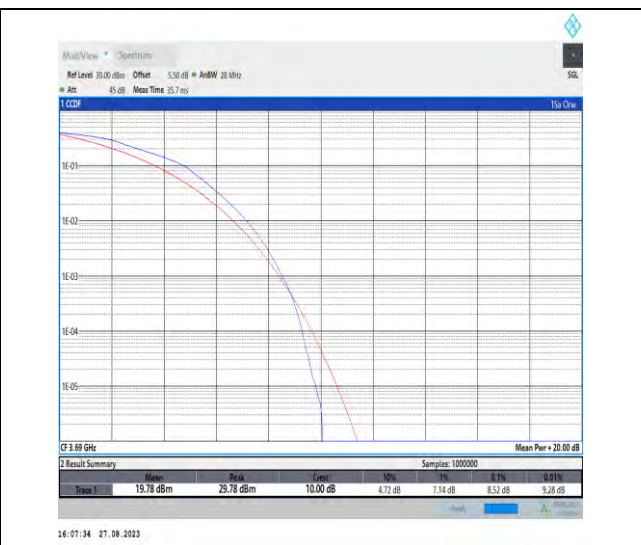
Band43-20MHz-16QAM-44490-100RB#0-PASS
