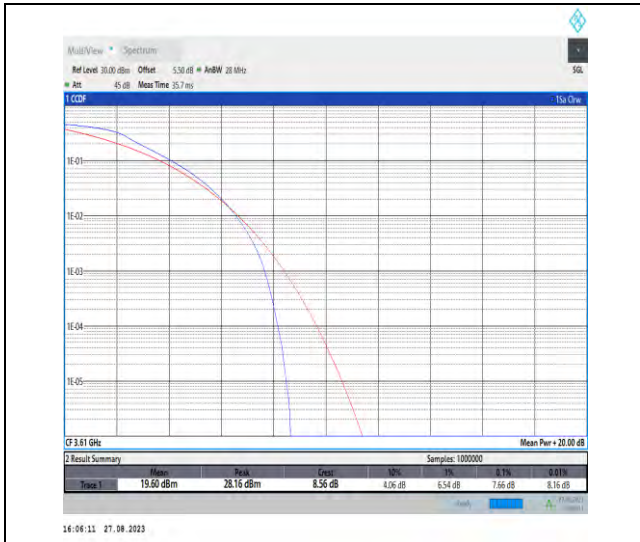
Band43-20MHz-QPSK-43690-100RB#0-PASS
