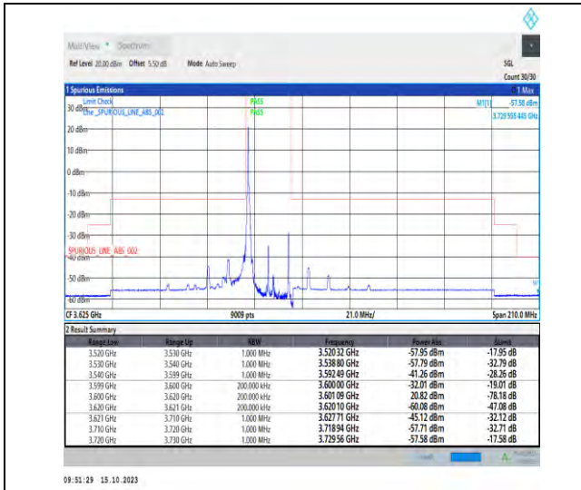
Band43_20MHz_QPSK_43690_1RB#0
