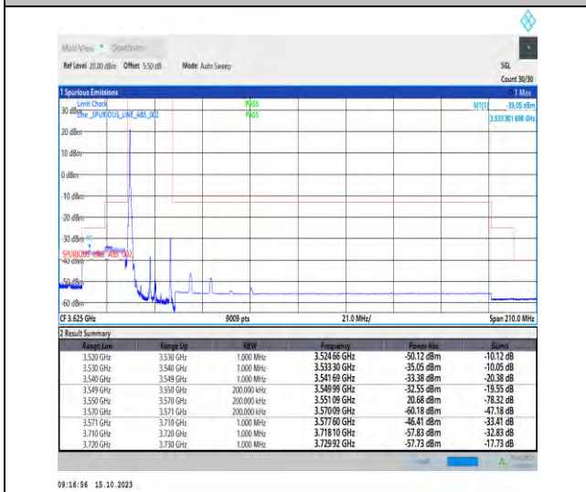
Band42_20MHz_QPSK_43190_1RB#0
