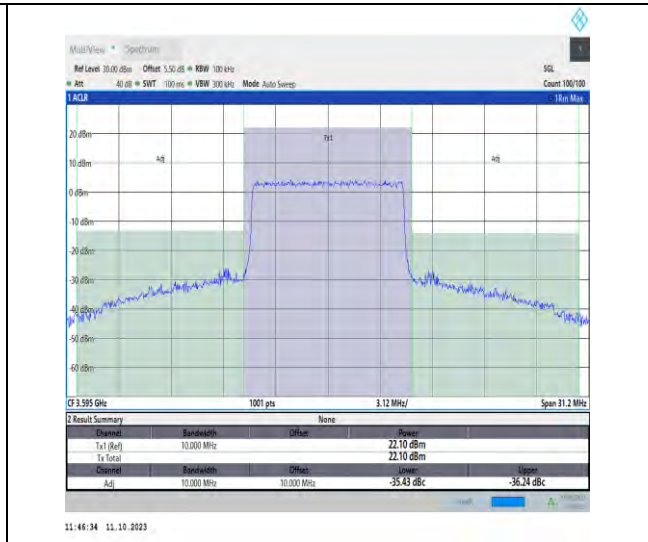
42(3550-3600)-10MHz-QPSK-43540-50RB#0-PASS
