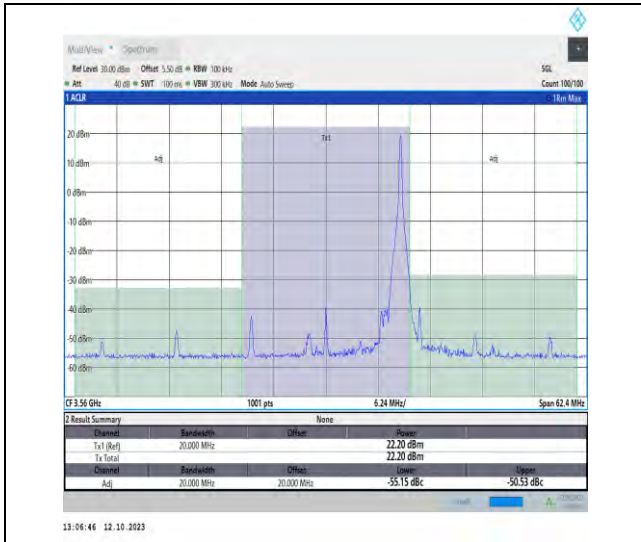
42(3550-3600)-20MHz-QPSK-43190-1RB#99-PASS
