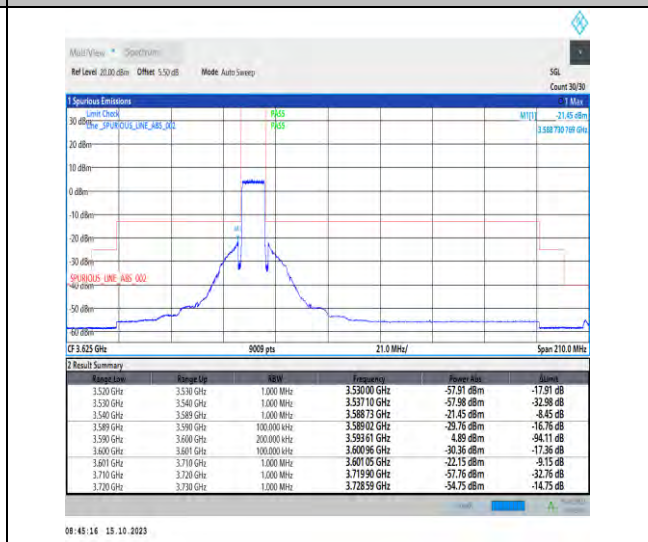
Band42_10MHz_QPSK_43540_50RB#0
