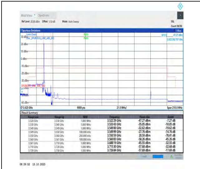
Band42_10MHz_QPSK_43140_1RB#0
