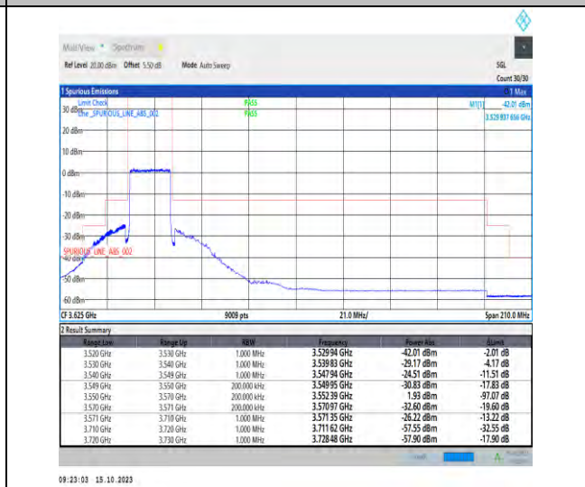
Band42_20MHz_QPSK_43190_100RB#0
