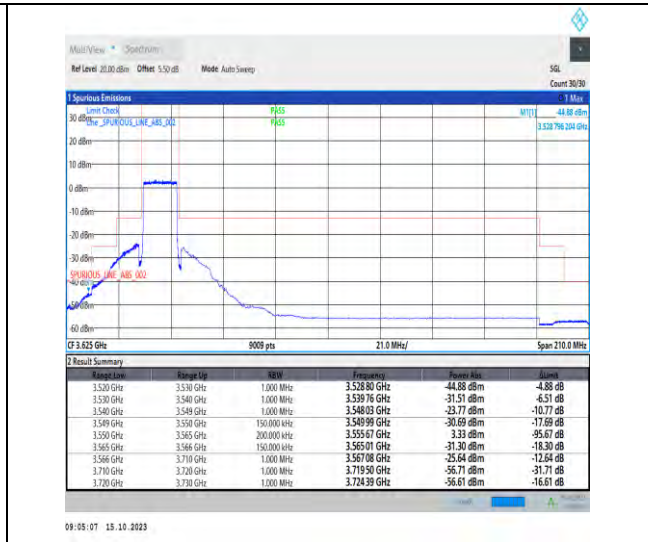
Band42_15MHz_QPSK_43165_75RB#0
