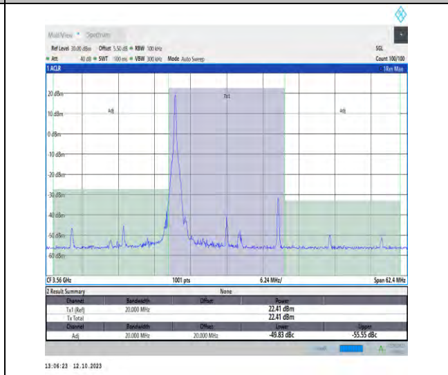
42(3550-3600)-20MHz-QPSK-43190-1RB#0-PASS
