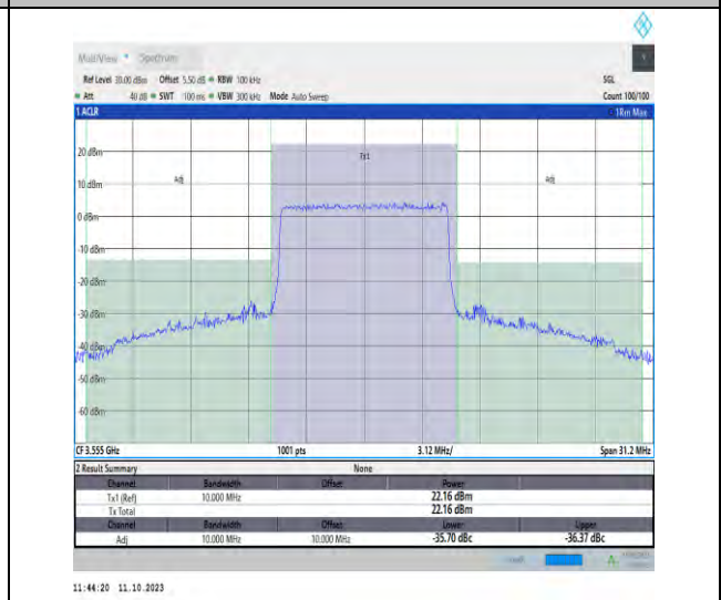
42(3550-3600)-10MHz-QPSK-43140-50RB#0-PASS
