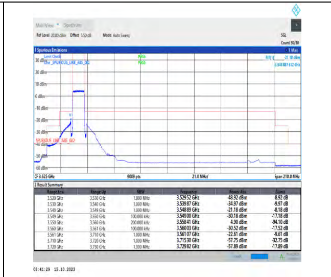
Band42_10MHz_QPSK_43140_50RB#0
