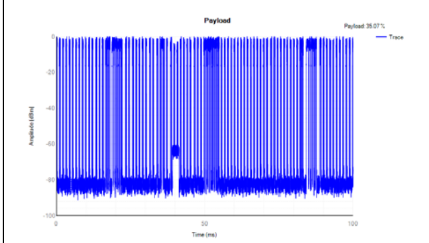
Bandwidth 20MHz
