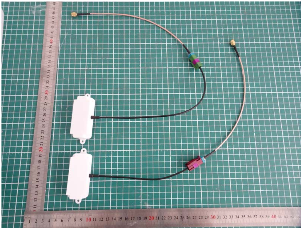
b: Antenna
