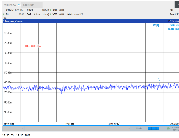
Band13-10MHz-QPSK-23230-1RB#0-Range2:0.15~30MHz
