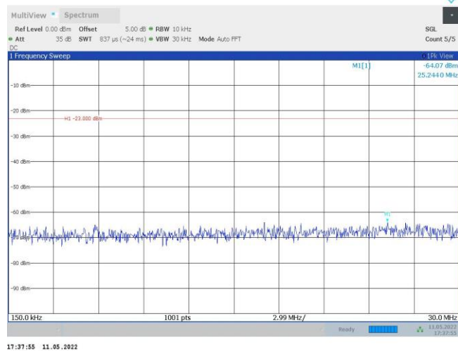
Band66-20MHz-QPSK-132072-1RB#0-Range2:0.15~30MHz
