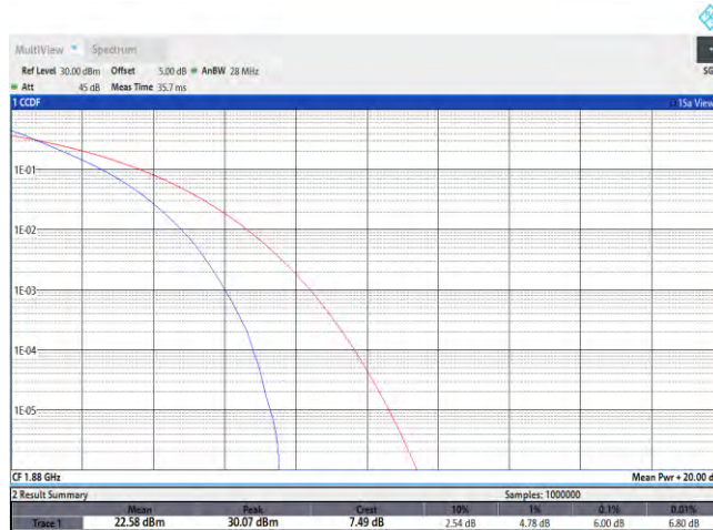
Band2-20MHz-QPSK-18900-100RB#0
