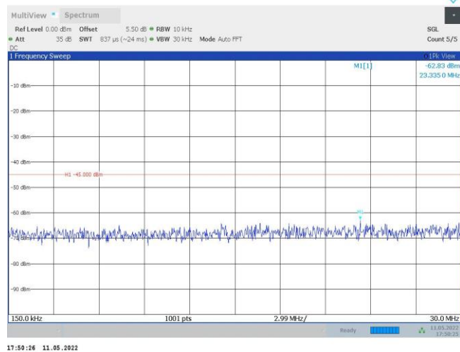
Band41-20MHz-QPSK-39750-1RB#0-Range2:0.15~30MHz
