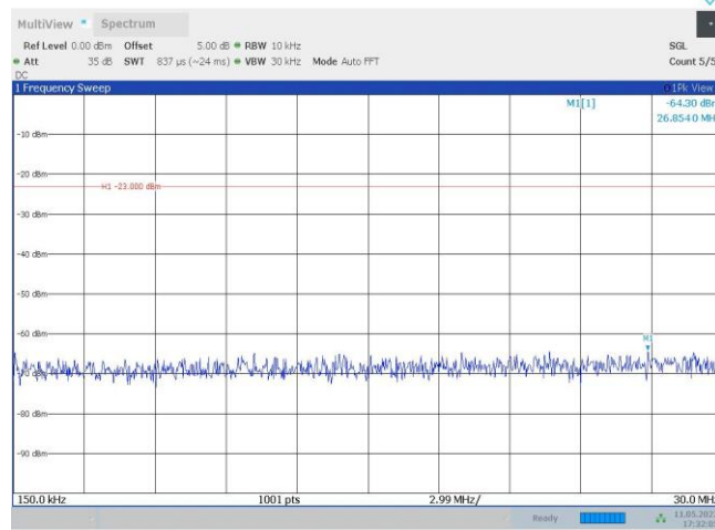
Band4-20MHz-QPSK-20050-1RB#0-Range2:0.15~30MHz
