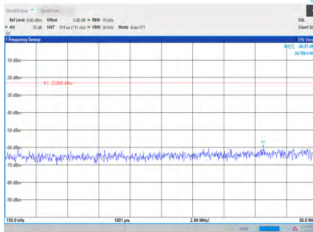
Band2-20MHz-QPSK-18700-1RB#0-Range2:0.15~30MHz
