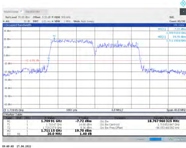
66-66-10MHz-10MHz-QPSK-QPSK-132373-132472-50RB#0-50RB#0
