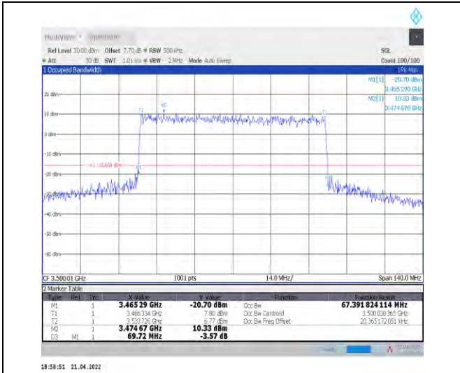
1-N78-3450-3550--30-70-M-7-CP-16QAM-Outer_Full -189@0-Ant1-67.392-69.720-≤70-PASS
