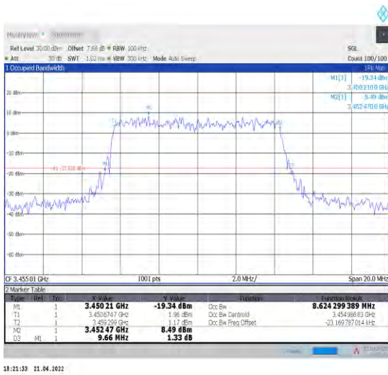
1-N78-3450-3550--30-10-L-9-CP-256QAM-Outer_Fu ll-24@0-Ant1-8.624-9.660-≤10-PASS
