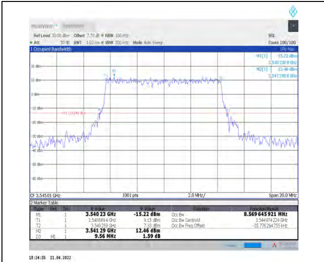
1-N78-3450-3550--30-10-H-3-DFT-16QAM-Outer_Fu II-24@0-Ant1-8.57-9.560-≤10-PASS
