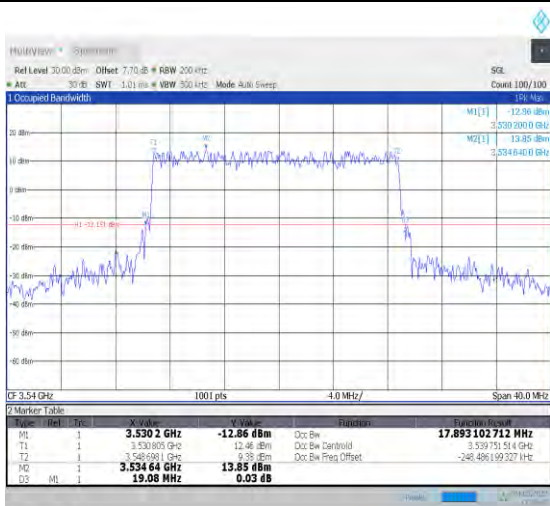
1-N78-3450-3550--30-20-H-1-DFT-QPSK-Outer_Full -50@0-Ant1-17.854-19.440-≤20-PASS
