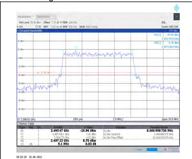
1-N78-3450-3550--30-10-M-9-CP-256QAM-Outer_Full -24@0-Ant1-8.567-9.100-≤10-PASS
