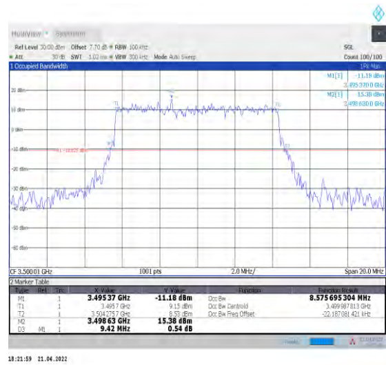
1-N78-3450-3550--30-10-M-1-DFT-QPSK-Outer_Full -24@0-Ant1-8.576-9.420-≤10-PASS
