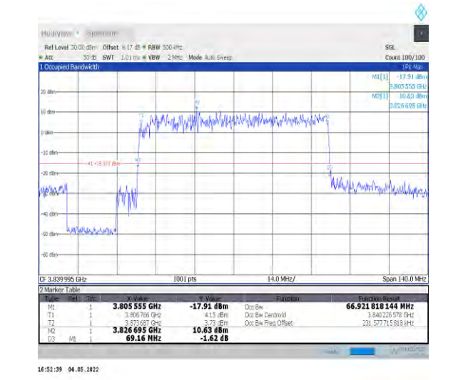
1-N77-3700-3980--30-70-M-6-CP-QPSK-Outer_Full-189@0-Ant1-66.922-69.160-≤70-PASS
