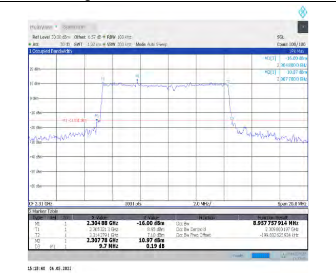
1-N30--15-10-L-3-DFT-16QAM-Outer_Full-50@0-Ant 1-8.958-9.700-≤10-PASS
