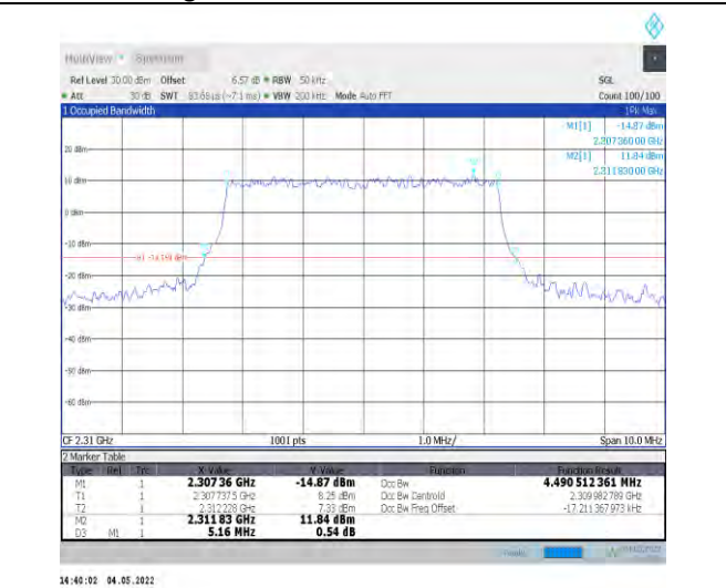
1-N30--15-5-M-1-DFT-QPSK-Outer_Full-25@0-Ant1 4.491-5.160-≤5-PASS
