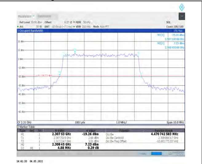
1-N30--15-5-M-9-CP-256QAM-Outer_Full-25@0-Ant1 1-4.471-4.880-≤5-PASS
