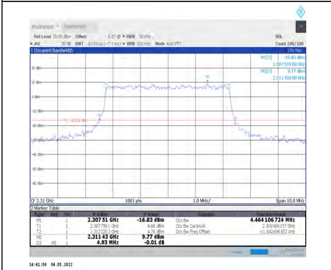
1-N30--15-5-M-6-CP-QPSK-Outer_Full-25@0-Ant1 4.464-4.930-≤5-PASS
