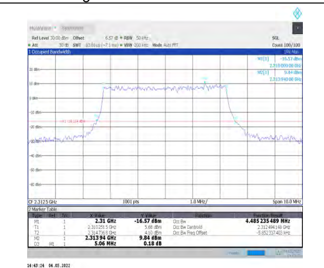
1-N30--15-5-H-8-CP-64QAM-Outer_Full-25@0-Ant1 4.485-5.060-≤5-PASS
