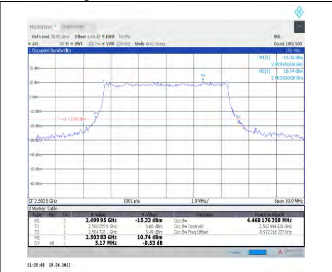
1-N7--15-5-L-6-CP-QPSK-Outer_Full-25@0-Ant1-4. 468-5.170-≤5-PASS
