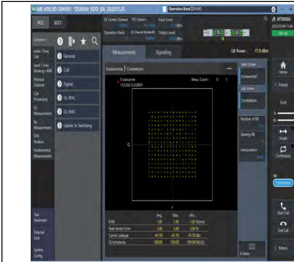
1-N7-PC3-15-40-M-9-CP-256QAM-Outer_Full-216@ 0-Ant1-see graph-PASS
