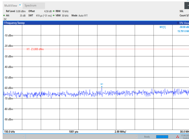
Band14-10MHz-QPSK-23330-1RB#0-Range2:0.15~30MHz
