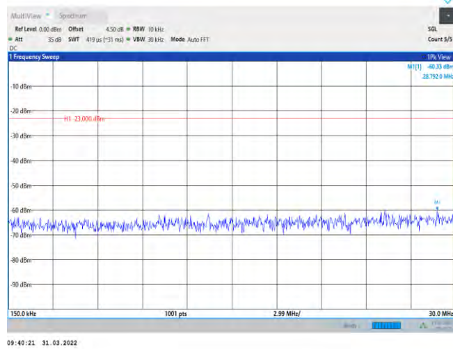
Band12-10MHz-QPSK-23060-1RB#0-Range2:0.15~30MHz
