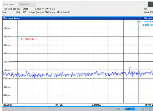
Band2-20MHz-QPSK-18700-1RB#0-Range2:0.15~30MHz
