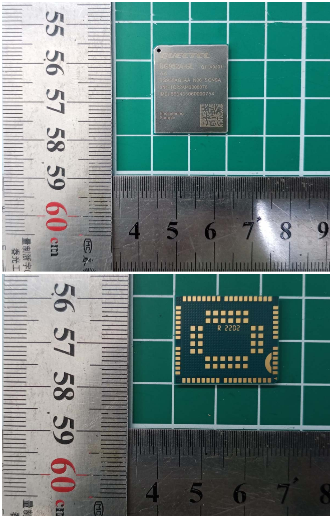
a: EUT
