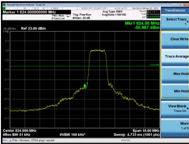
LTE-M Band 5 QPSK 5MHz CH-Low 1RB
